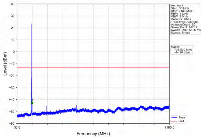
Band12_10MHz_QPSK_MCH_707.5MHz_RB_1_0_NTNV
