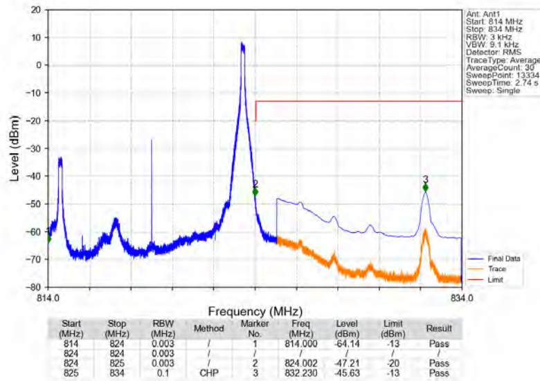
Band26a_10MHz_QPSK_MCH_819MHz_RB_50_0_NTNV
