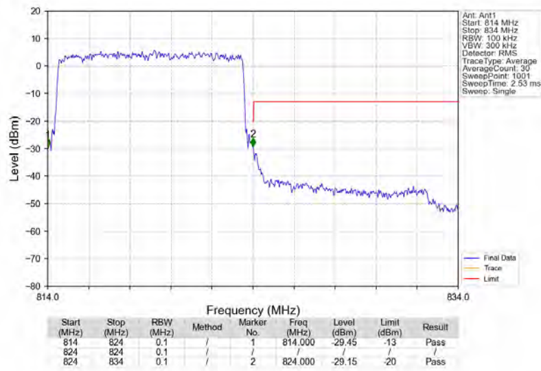
Band26a_10MHz_QPSK_MCH_819MHz_RB_50_0_NTNV
