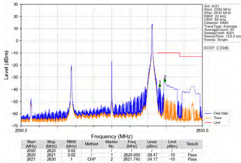
Band38 20MHz 16QAM HCH 2610MHz RB 1 99 NTNV
