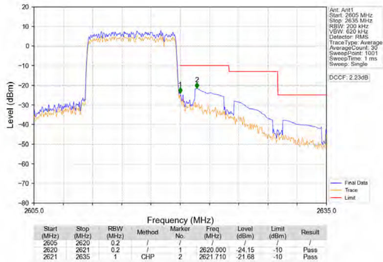
Band38 10MHz 16QAM HCH 2615MHz RB 50 0 NTNV
