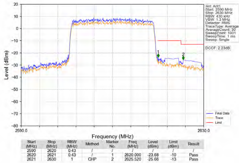
Band38 20MHz QPSK HCH 2610MHz RB 100 0 NTN
