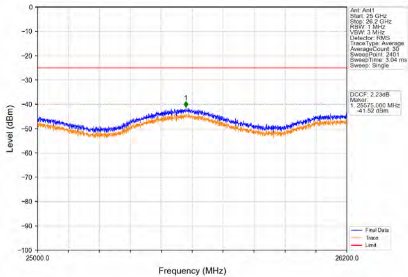
Band38_20MHz_QPSK_HCH_2610MHz_RB_1_99_NTNV
