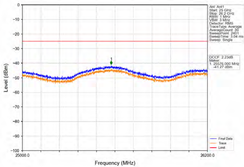
Band38_20MHz_QPSK_LCH_2580MHz_RB_1_0_NTNV
