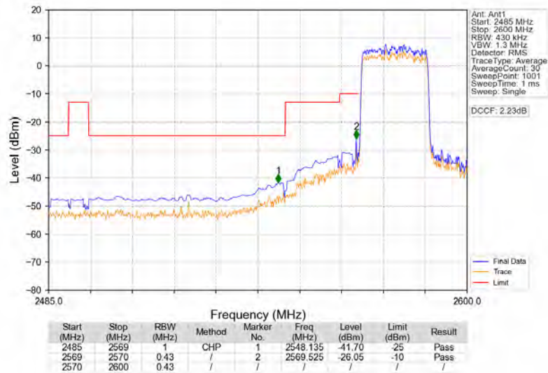
Band38_20MHz_16QAM_LCH_2580MHz_RB_100_0_NTNV
