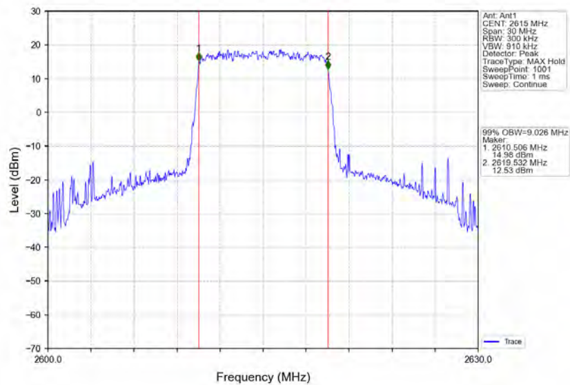
Band38_10MHz_QPSK_HCH_2615MHz_RB_50_0_NTNV
