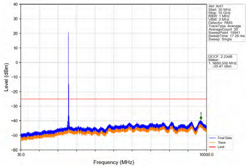
Band38_20MHz_16QAM_MCH_2595MHz_RB_1_0_NTNV
