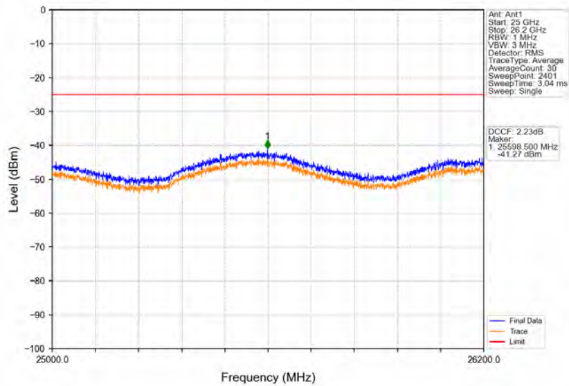
Band38_20MHz_16QAM_LCH_2580MHz_RB_100_0_NTNV
