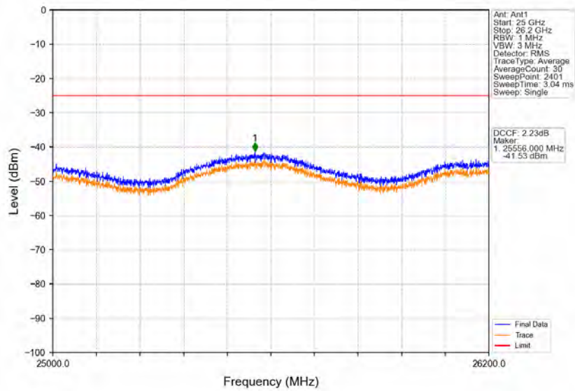
Band38_20MHz_16QAM_HCH_2610MHz_RB_1_0_NTNV
