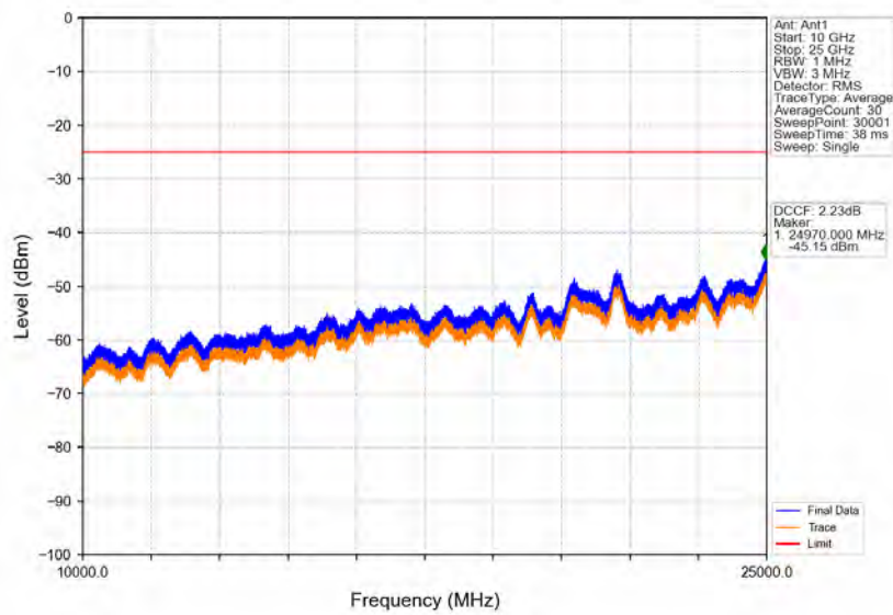
Band38_20MHz_16QAM_MCH_2595MHz_RB_1_0_NTNV
