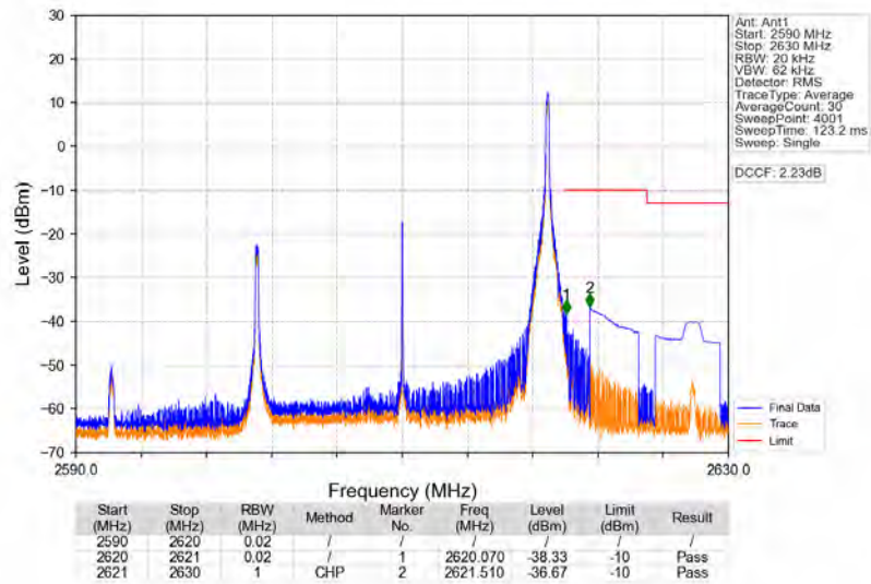
Band38_20MHz_64QAM_HCH_2610MHz_RB_1_99_NTNV
