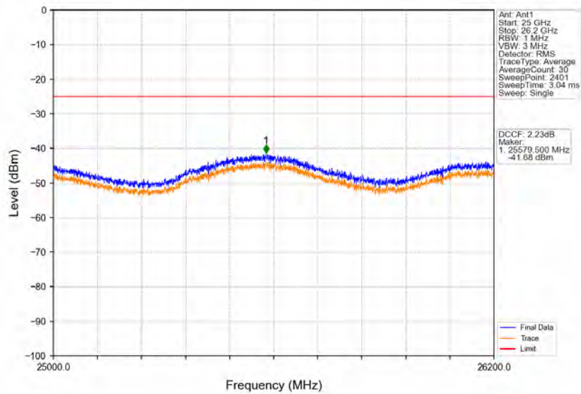
Band38_10MHz_QPSK_HCH_2615MHz_RB_1_49_NTNV
