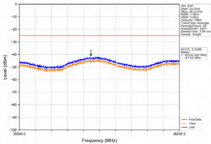
Band38_10MHz_QPSK_LCH_2575MHz_RB_1_0_NTNV
