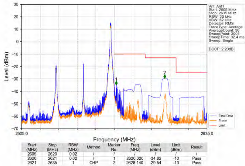
Band38_10MHz_QPSK_HCH_2615MHz_RB_1_49_NTNV
