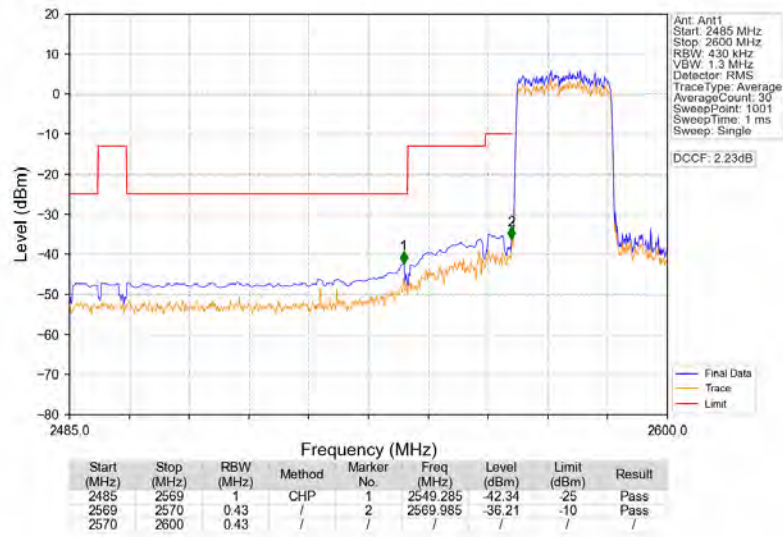
Band38_20MHz_64QAM_LCH_2580MHz_RB_100_0_NTNV
