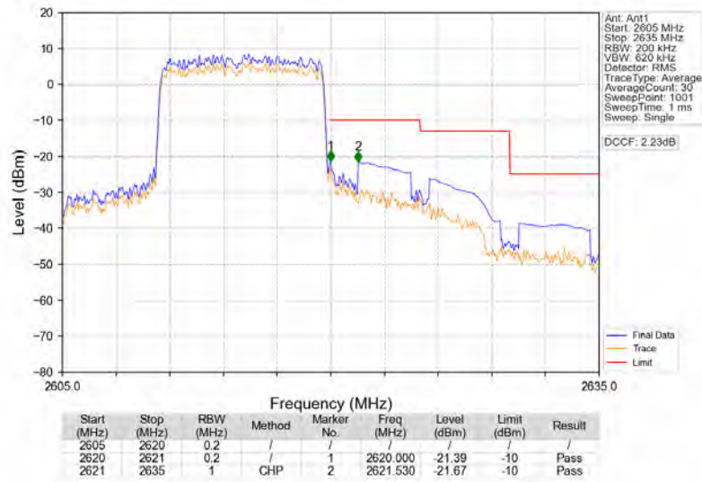
Band38_10MHz_QPSK_HCH_2615MHz_RB_50_0_NTNV
