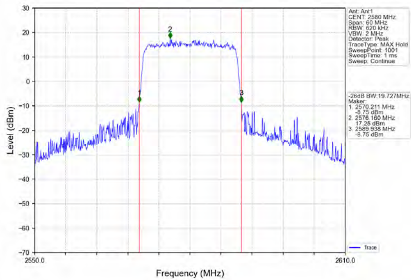
Band38_20MHz_64QAM_LCH_2580MHz_RB_100_0_NTNV
