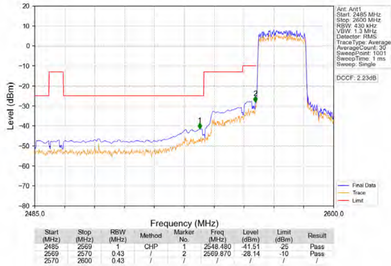
Band38_20MHz_QPSK_LCH_2580MHz_RB_100_0_NTNV
