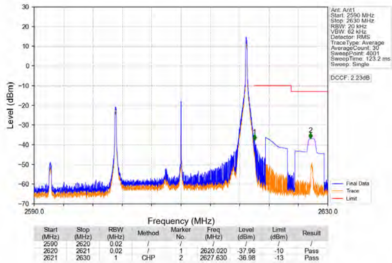
Band38_20MHz_QPSK_HCH_2610MHz_RB_1_99_NTNV
