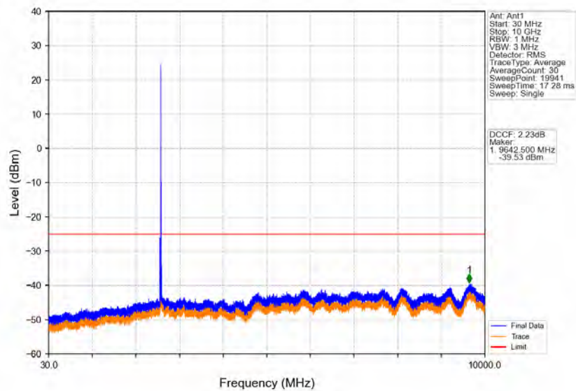
Band38_10MHz_QPSK_MCH_2595MHz_RB_1_0_NTNV
