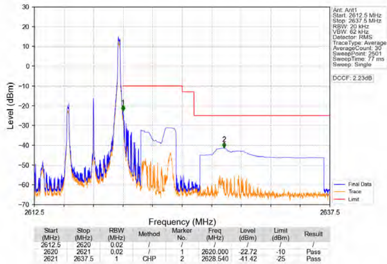
Band38_5MHz_QPSK_HCH_2617.5MHz_RB_1_24_NTNV
