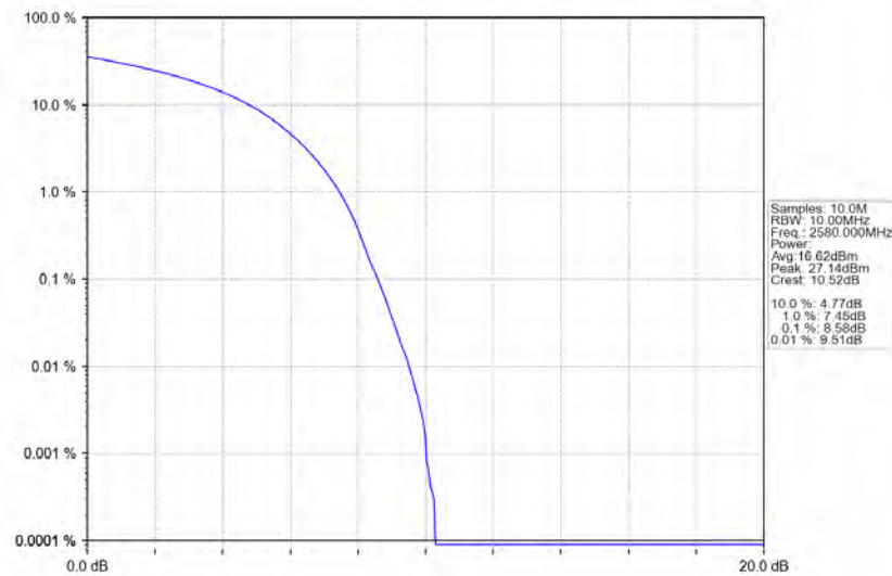
Band38_20MHz_16QAM_LCH_2580MHz_RB_100_0_NTNV
