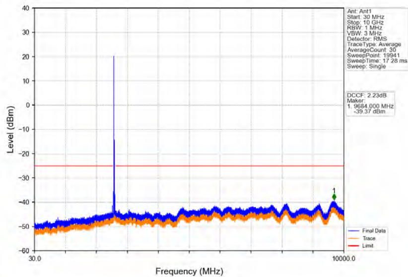
Band38_20MHz_QPSK_MCH_2595MHz_RB_1_0_NTNV
