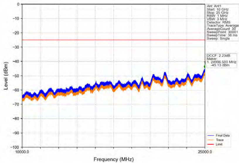
Band38_20MHz_QPSK_MCH_2595MHz_RB_1_0_NTNV
