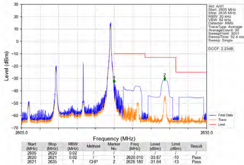
Band38 10MHz 16QAM HCH 2615MHz RB 1 49 NTNV
