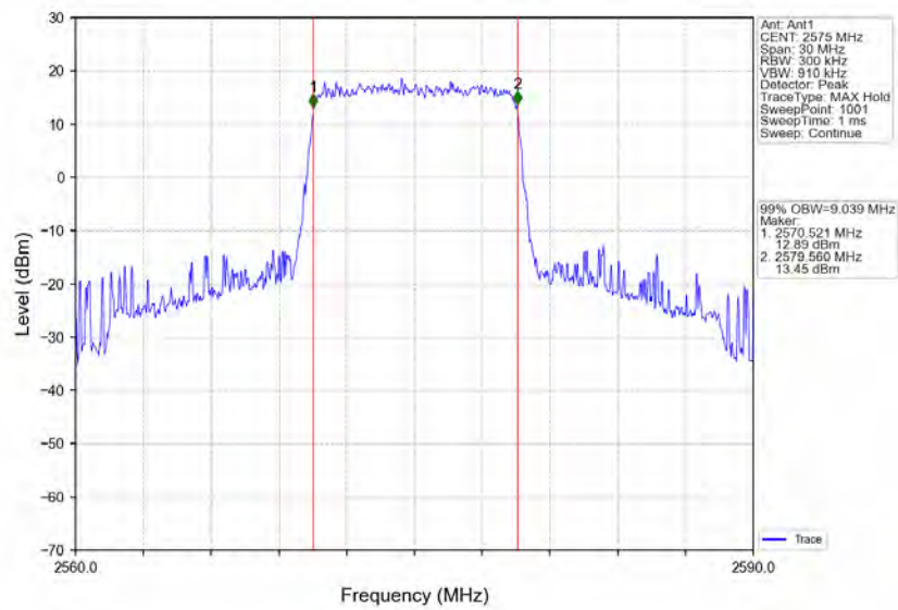
Band38_10MHz_QPSK_LCH_2575MHz_RB_50_0_NTNV
