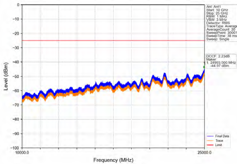
Band38_20MHz_16QAM_LCH_2580MHz_RB_1_0_NTNV
