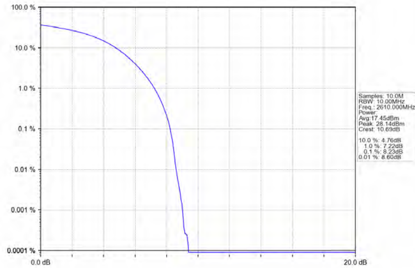
Band38_20MHz_QPSK_HCH_2610MHz_RB_100_0_NTNV
