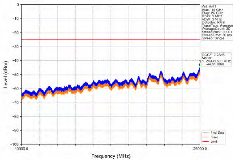
Band38_10MHz_QPSK_HCH_2615MHz_RB_1_0_NTNV
