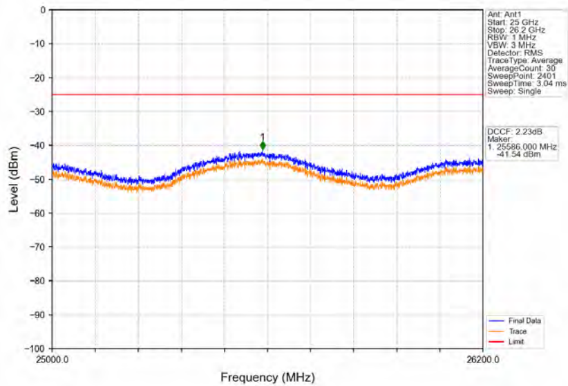
Band38_20MHz_64QAM_HCH_2610MHz_RB_1_99_NTNV
