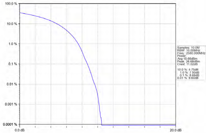
Band38_20MHz_64QAM_LCH_2580MHz_RB_100_0_NTNV
