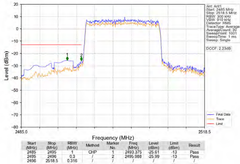
Band41_15MHz_QPSK_LCH_2503.5MHz_RB_75_0_NTNV
