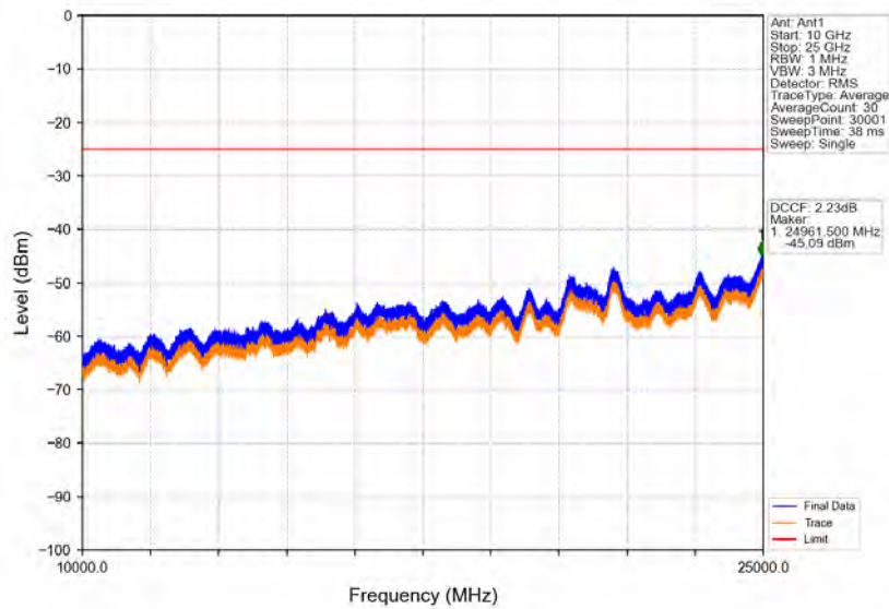
Band41_10MHz_16QAM_HCH_2685MHz_RB_1_0_NTNV
