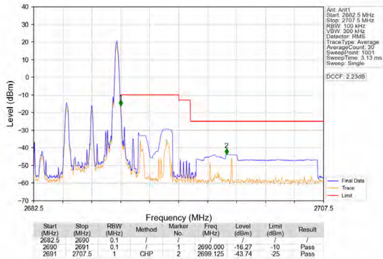
Band41_5MHz_QPSK_HCH_2687.5MHz_RB_1_24_NTNV
