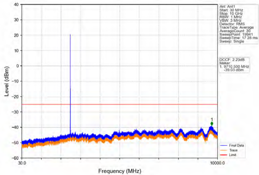
Band41_10MHz_16QAM_LCH_2501MHz_RB_1_0_NTNV
