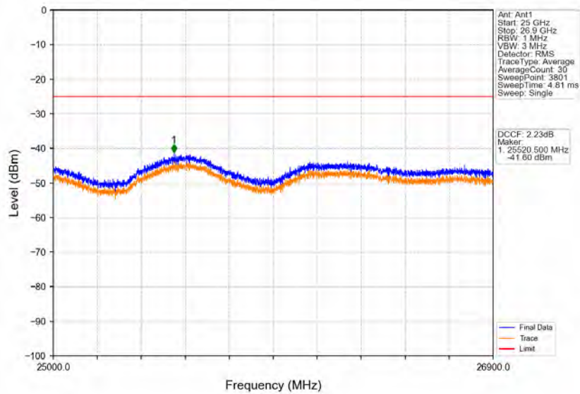
Band41_10MHz_16QAM_LCH_2501MHz_RB_50_0_NTNV
