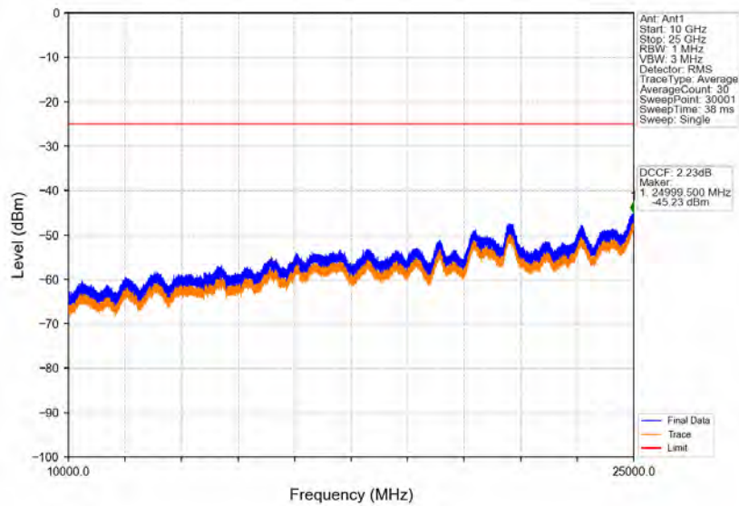
Band41_10MHz_QPSK_MCH_2593MHz_RB_1_0_NTNV
