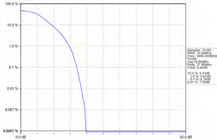
Band41_10MHz_QPSK_HCH_2685MHz_RB_50_0_NTNV
