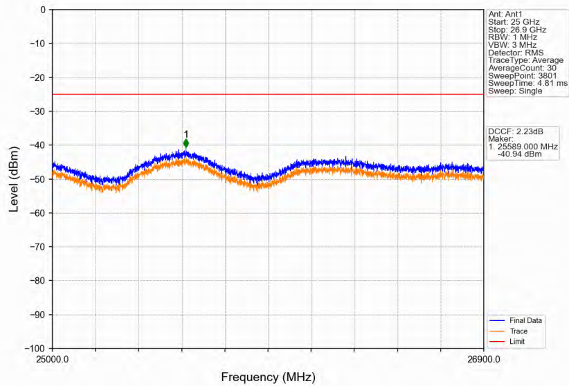
Band41_15MHz_QPSK_HCH_2682.5MHz_RB_1_74_NTNV
