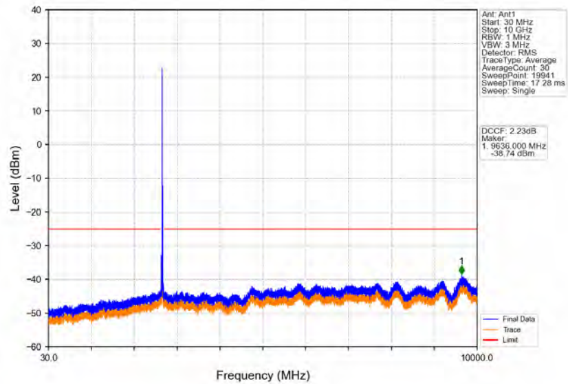
Band41_20MHz_QPSK_HCH_2680MHz_RB_1_0_NTNV
