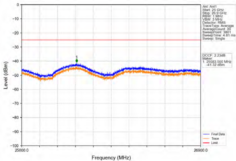
Band41_10MHz_QPSK_LCH_2501MHz_RB_1_0_NTNV
