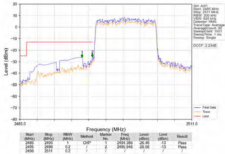
Band41_10MHz_QPSK_LCH_2501MHz_RB_50_0_NTNV
