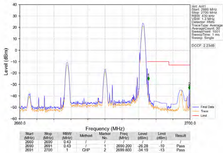
Band41_20MHz_QPSK_HCH_2680MHz_RB_1_99_NTNV
