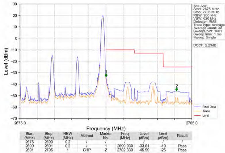
Band41_10MHz_64QAM_HCH_2685MHz_RB_1_49_NTNV
