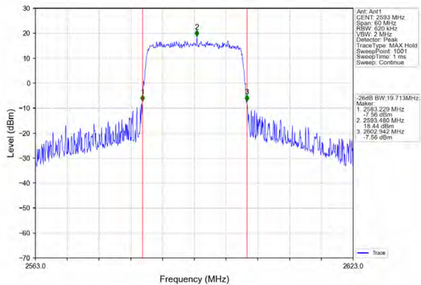
Band41_20MHz_16QAM_MCH_2593MHz_RB_100_0_NTNV
