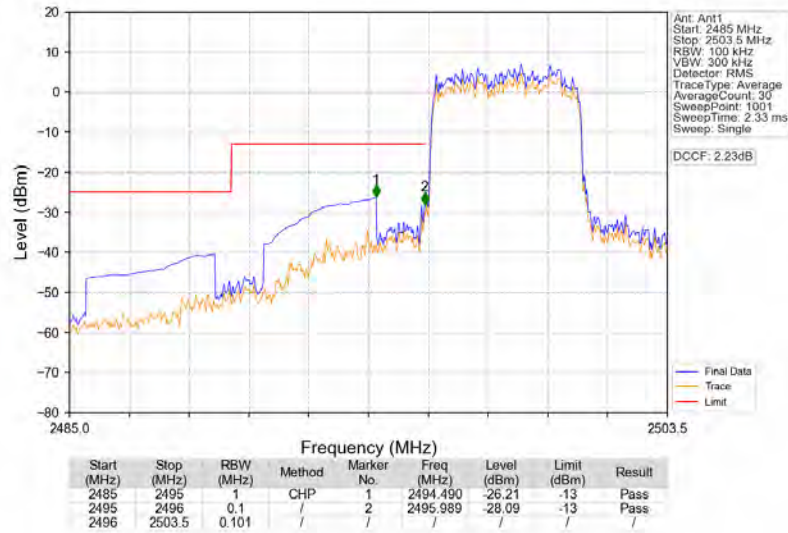
Band41_5MHz_QPSK_LCH_2498.5MHz_RB_25_0_NTNV
