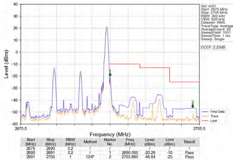
Band41_10MHz_16QAM_HCH_2685MHz_RB_1_49_NTNV
