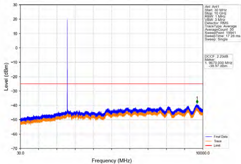
Band41_5MHz_QPSK_MCH_2593MHz_RB_1_0_NTNV
