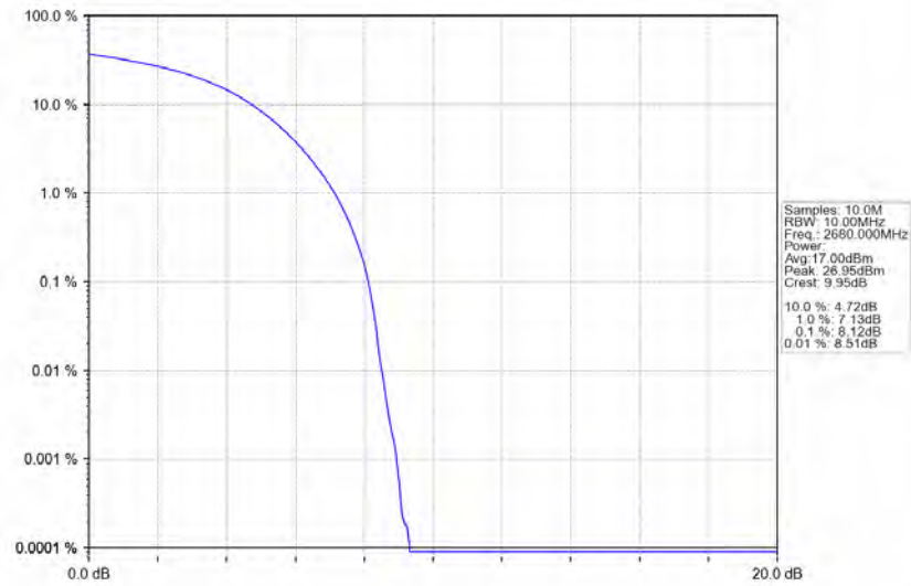
Band41_20MHz_QPSK_HCH_2680MHz_RB_100_0_NTNV
