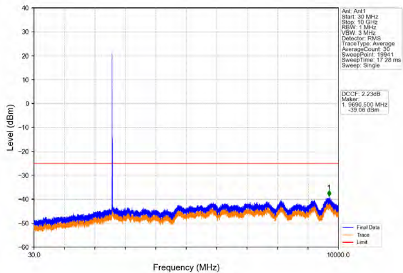
Band41_10MHz_QPSK_MCH_2593MHz_RB_1_0_NTNV
