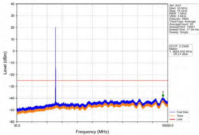
Band41_20MHz_QPSK_MCH_2593MHz_RB_1_0_NTNV
