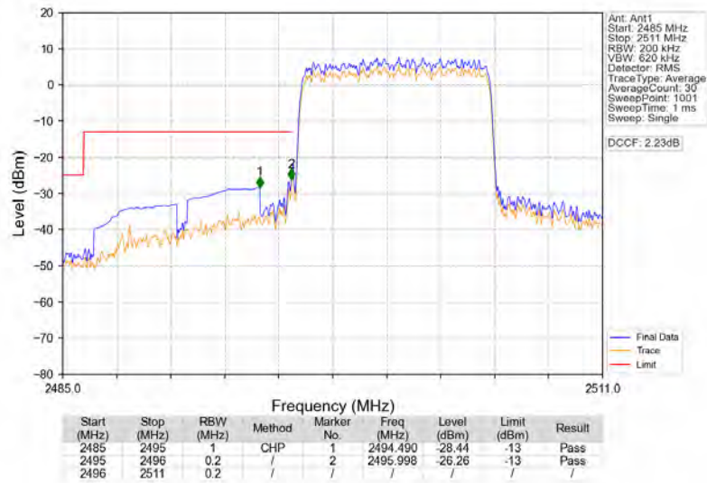
Band41_10MHz_16QAM_LCH_2501MHz_RB_50_0_NTNV
