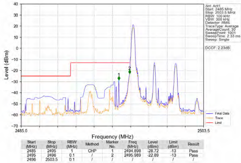
Band41_5MHz_QPSK_LCH_2498.5MHz_RB_1_0_NTNV
