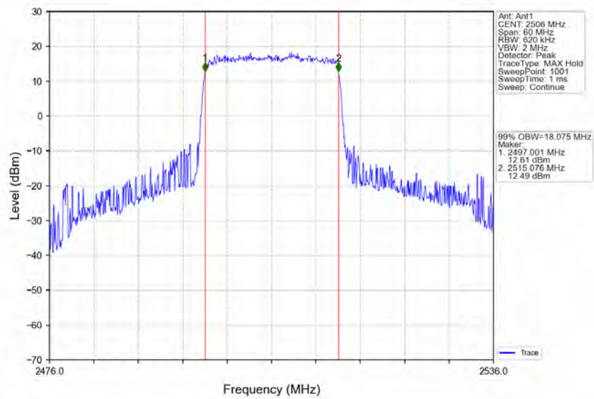
Band41_20MHz_QPSK_LCH_2506MHz_RB_100_0_NTNV
