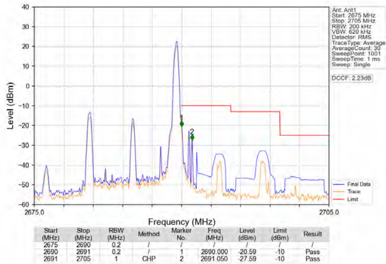
Band41_10MHz_QPSK_HCH_2685MHz_RB_1_49_NTNV
