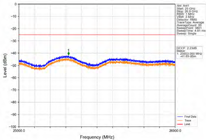
Band41_15MHz_QPSK_LCH_2503.5MHz_RB_1_0_NTNV
