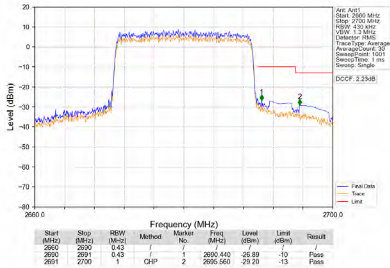
Band41_20MHz_QPSK_HCH_2680MHz_RB_100_0_NTNV
