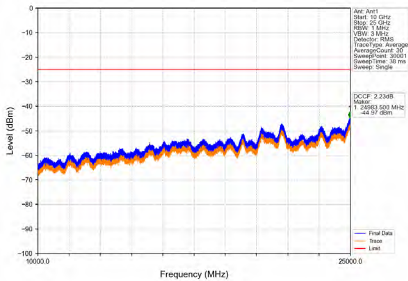
Band41_20MHz_16QAM_MCH_2593MHz_RB_1_0_NTNV
