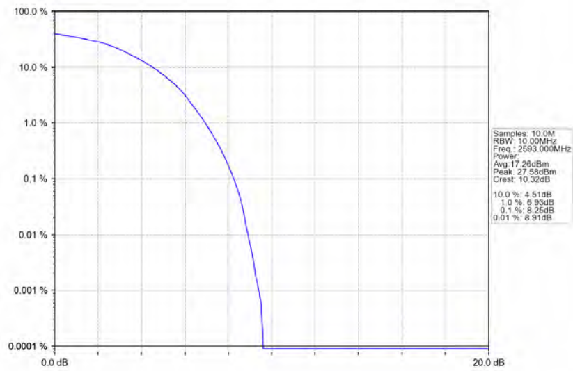
Band41_10MHz_64QAM_MCH_2593MHz_RB_50_0_NTNV
