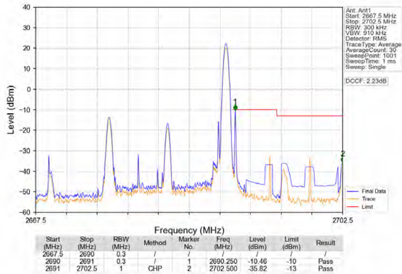
Band41_15MHz_QPSK_HCH_2682.5MHz_RB_1_74_NTNV
