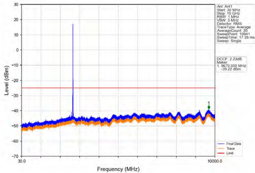
Band41_15MHz_QPSK_HCH_2682.5MHz_RB_1_0_NTNV
