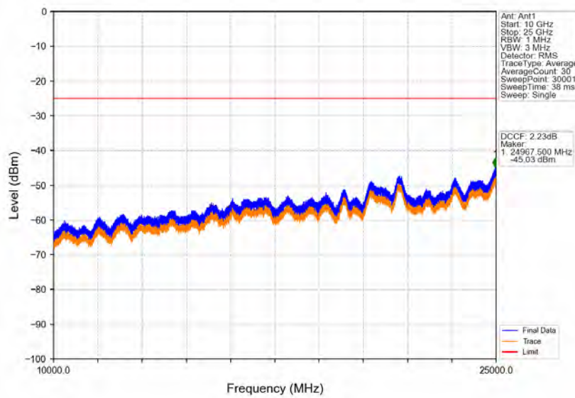
Band41_20MHz_QPSK_HCH_2680MHz_RB_1_0_NTNV
