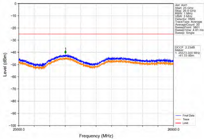
Band41_10MHz_64QAM_HCH_2685MHz_RB_1_49_NTNV
