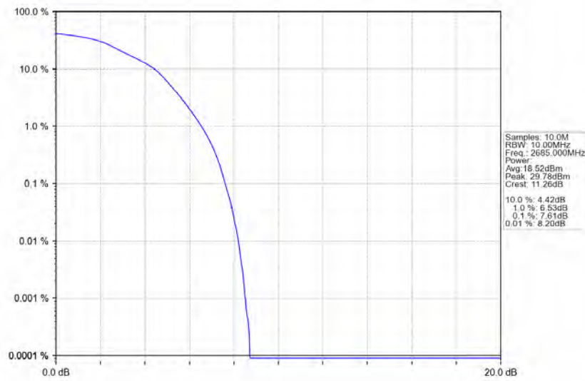
Band41_10MHz_16QAM_HCH_2685MHz_RB_50_0_NTNV
