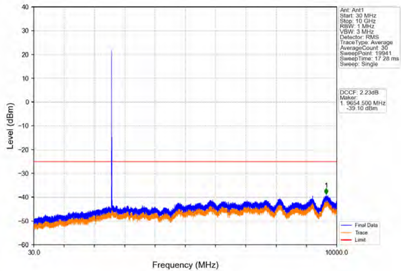
Band41_10MHz_16QAM_MCH_2593MHz_RB_1_0_NTNV
