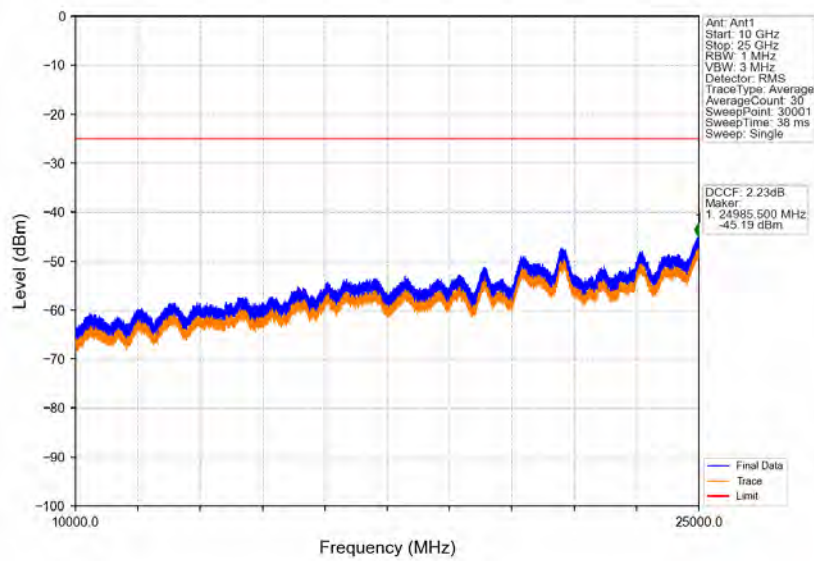
Band41_10MHz_16QAM_LCH_2501MHz_RB_1_0_NTNV
