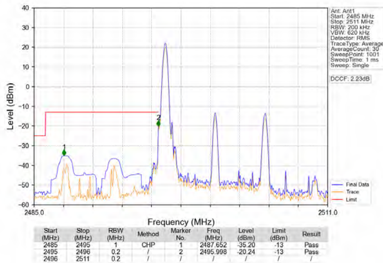
Band41_10MHz_16QAM_LCH_2501MHz_RB_1_0_NTNV
