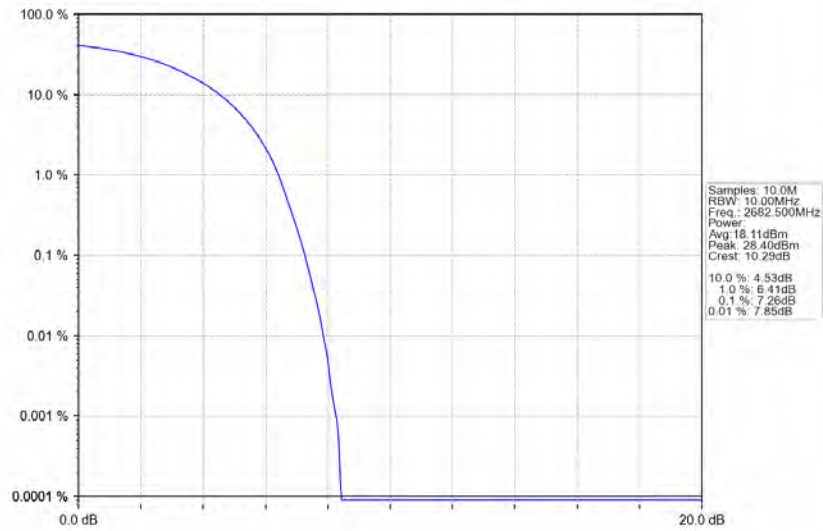
Band41_15MHz_QPSK_HCH_2682.5MHz_RB_75_0_NTNV
