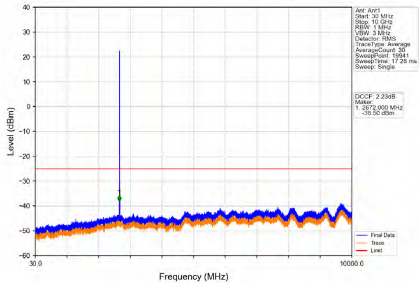
Band41_5MHz_QPSK_HCH_2687.5MHz_RB_1_0_NTNV
