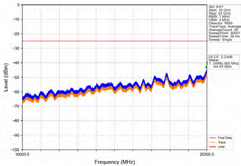
Band41_5MHz_QPSK_HCH_2687.5MHz_RB_1_0_NTNV
