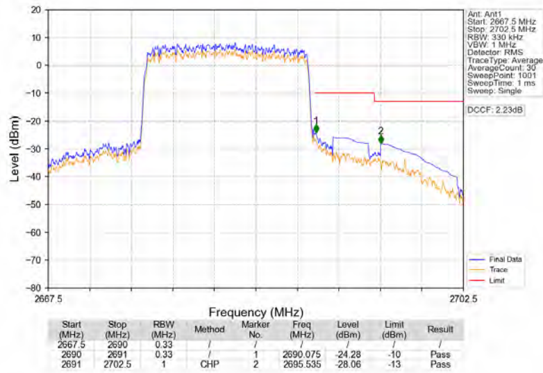
Band41_15MHz_QPSK_HCH_2682.5MHz_RB_75_0_NTNV
