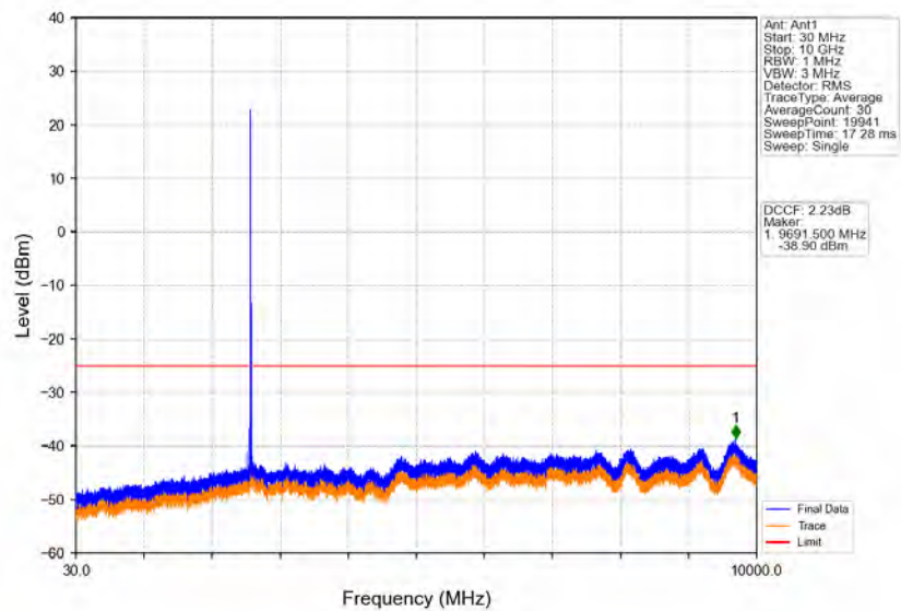
Band41_15MHz_QPSK_MCH_2593MHz_RB_1_0_NTNV
