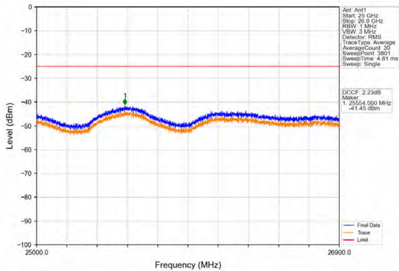
Band41_20MHz_QPSK_HCH_2680MHz_RB_1_99_NTNV
