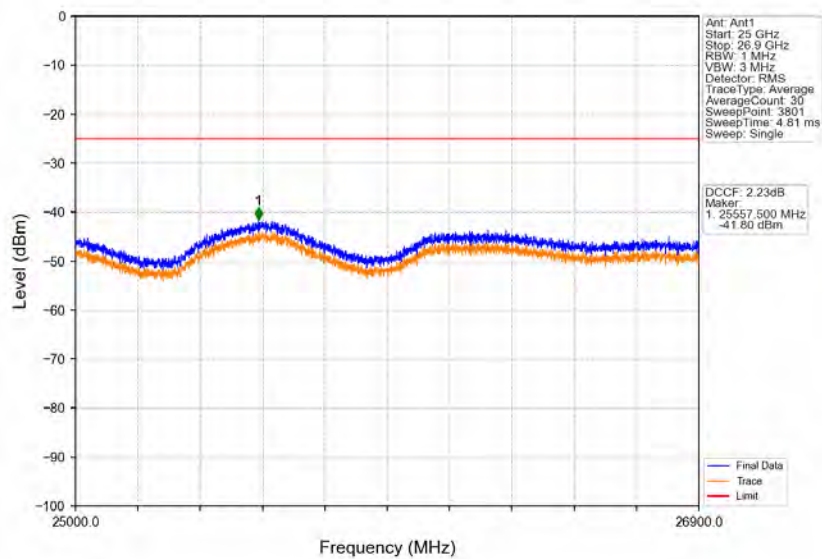
Band41_20MHz_QPSK_LCH_2506MHz_RB_1_0_NTNV
