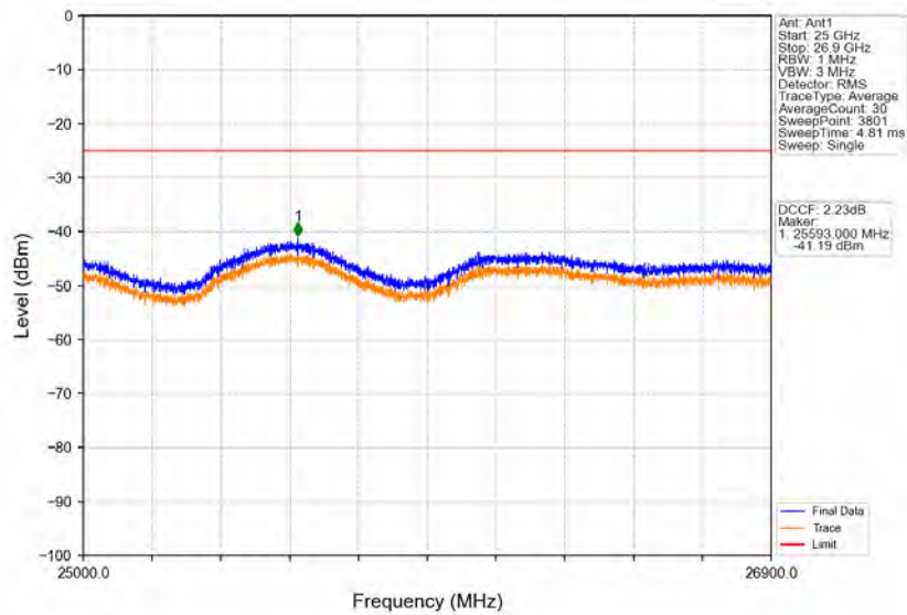
Band41_10MHz_QPSK_HCH_2685MHz_RB_1_49_NTNV
