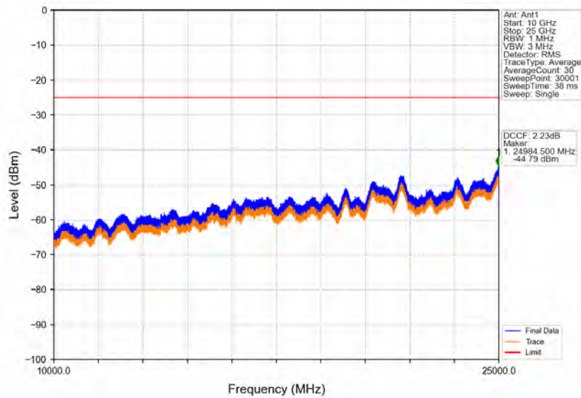
Band41_5MHz_QPSK_MCH_2593MHz_RB_1_0_NTNV
