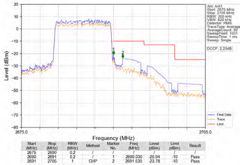
Band41_10MHz_QPSK_HCH_2685MHz_RB_50_0_NTNV
