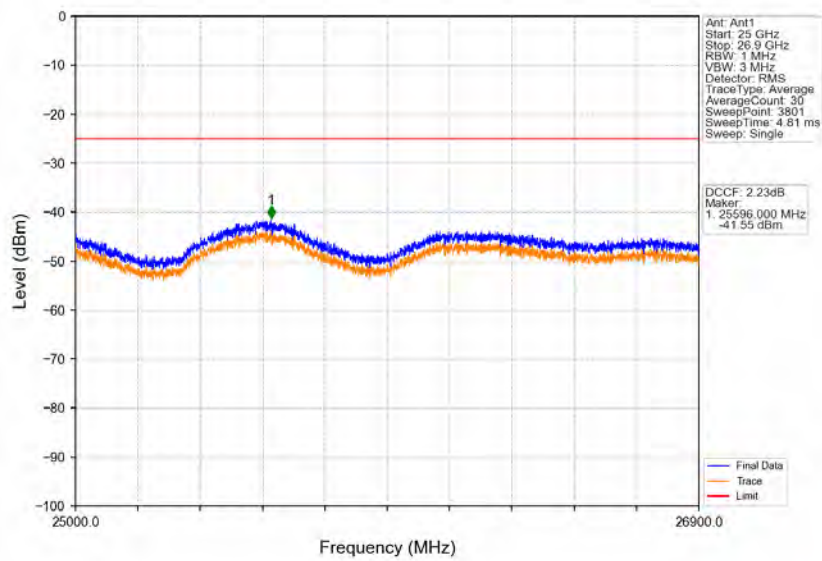
Band41_10MHz_16QAM_HCH_2685MHz_RB_1_0_NTNV
