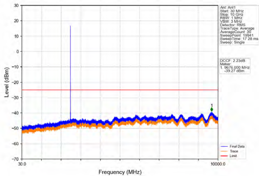
Band41_5MHz_QPSK_LCH_2498.5MHz_RB_1_0_NTNV
