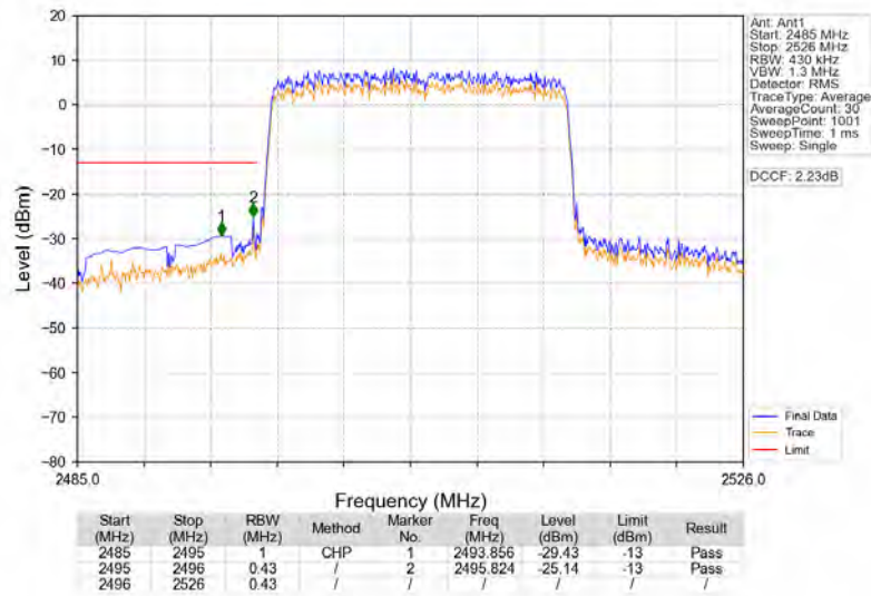
Band41_20MHz_QPSK_LCH_2506MHz_RB_100_0_NTNV
