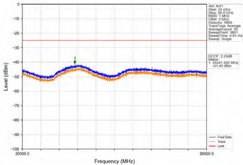
Band41_5MHz_QPSK_HCH_2687.5MHz_RB_1_24_NTNV
