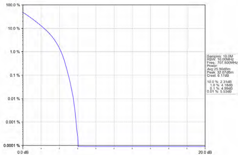
Band12_10MHz_QPSK_MCH_707.5MHz_RB_50_0_NTNV
