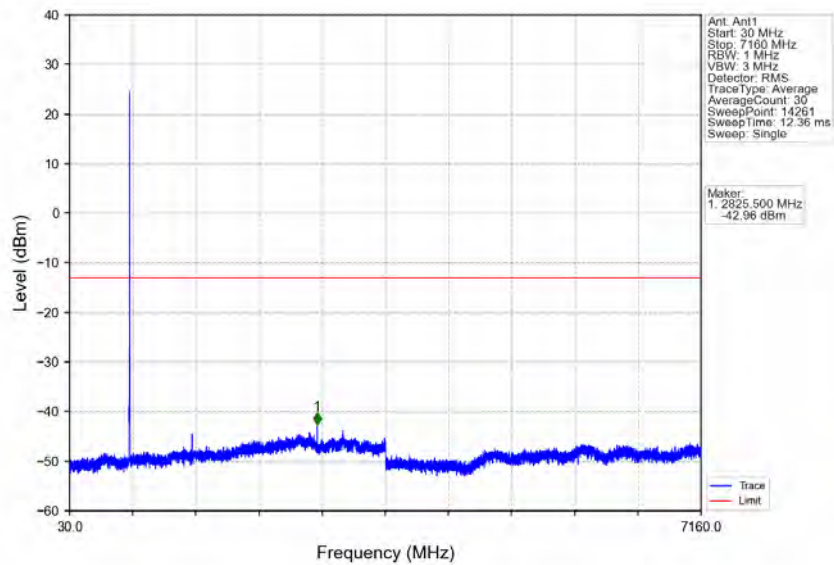
Band12_3MHz_QPSK_MCH_707.5MHz_RB_1_0_NTNV
