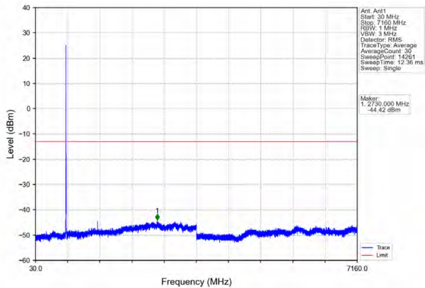
Band12_10MHz_QPSK_MCH_707.5MHz_RB_1_0_NTNV
