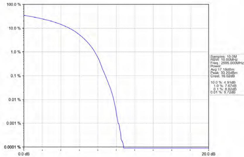
Band38_20MHz_16QAM_MCH_2595MHz_RB_100_0_NTNV
