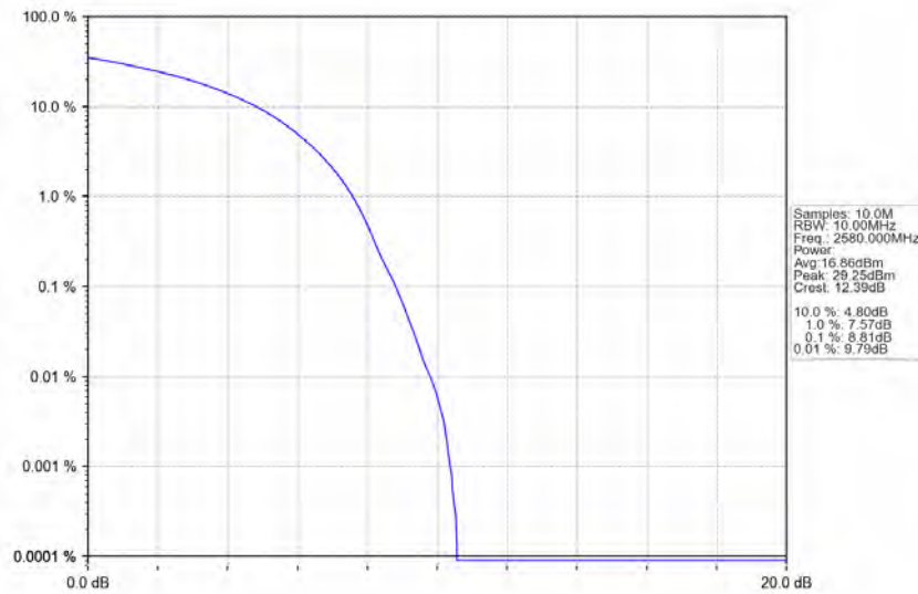
Band38_20MHz_64QAM_LCH_2580MHz_RB_100_0_NTNV
