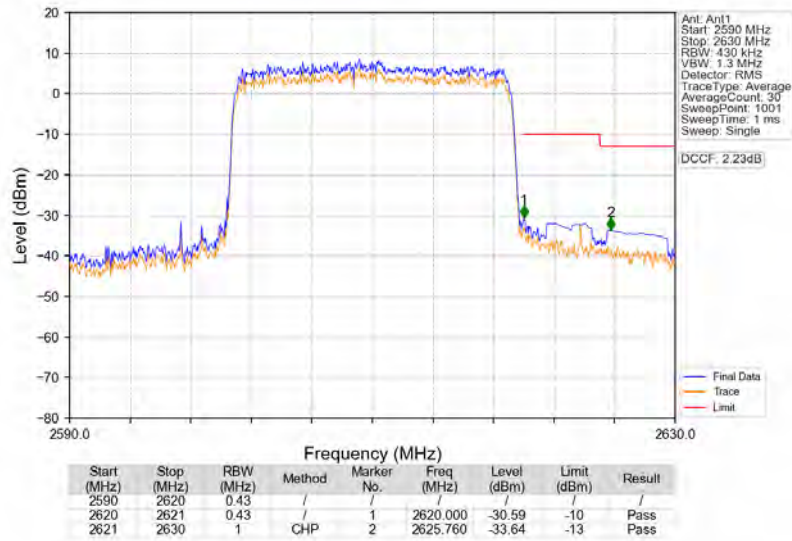
Band38_20MHz_16QAM_HCH_2610MHz_RB_100_0_NTNV
