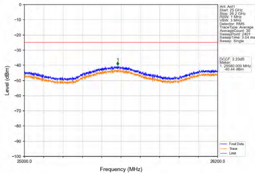
Band38_20MHz_16QAM_HCH_2610MHz_RB_1_0_NTNV
