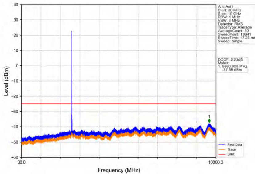
Band38_10MHz_QPSK_HCH_2615MHz_RB_1_0_NTNV
