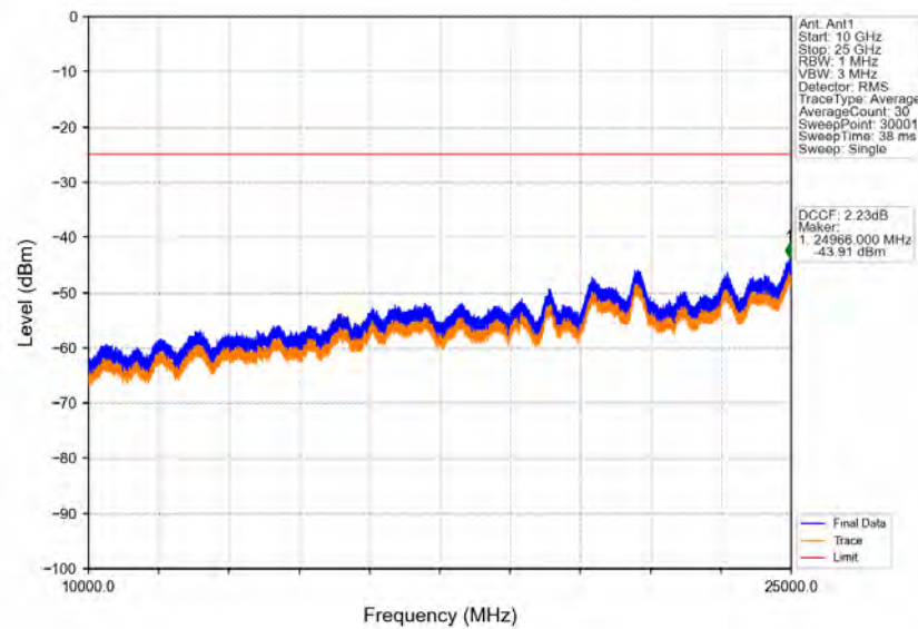
Band38_20MHz_QPSK_MCH_2595MHz_RB_1_0_NTNV
