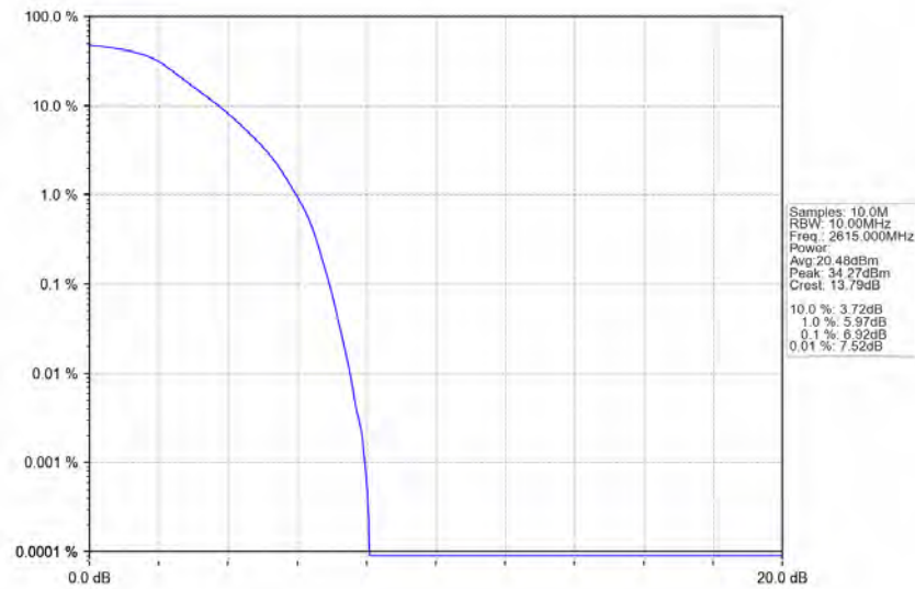
Band38_10MHz_QPSK_HCH_2615MHz_RB_50_0_NTNV
