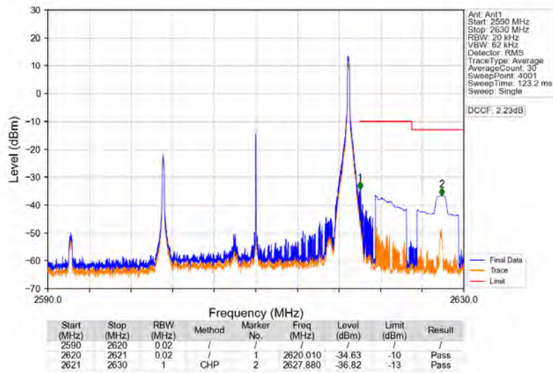
Band38_20MHz_QPSK_HCH_2610MHz_RB_1_99_NTNV
