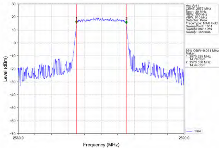
Band38_10MHz_QPSK_LCH_2575MHz_RB_50_0_NTNV
