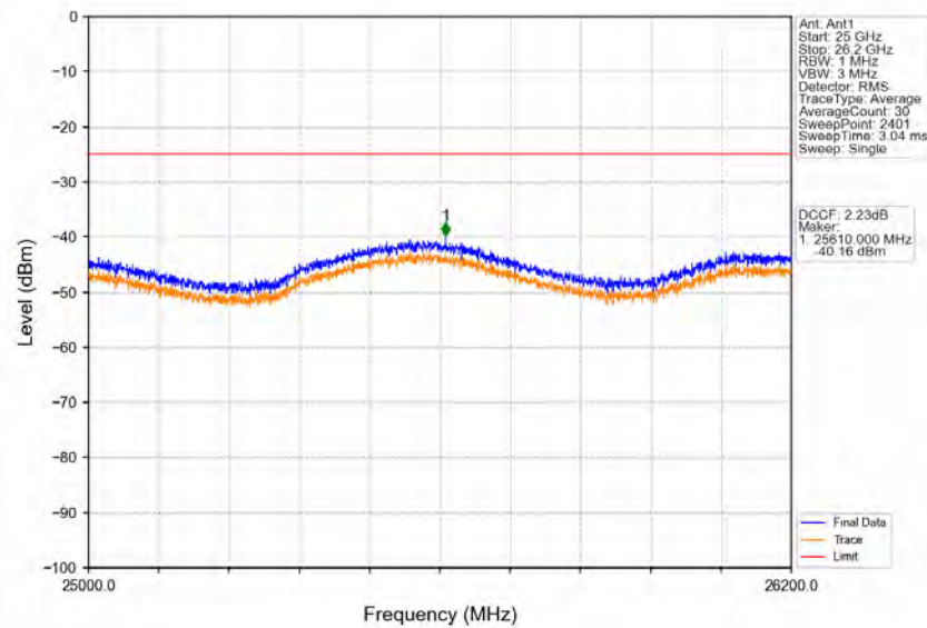
Band38_10MHz_QPSK_LCH_2575MHz_RB_1_0_NTNV
