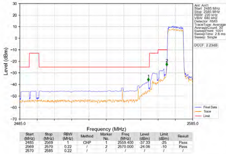
Band38_10MHz_QPSK_LCH_2575MHz_RB_50_0_NTNV
