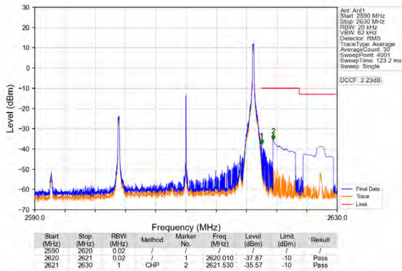
Band38_20MHz_64QAM_HCH_2610MHz_RB_1_99_NTNV
