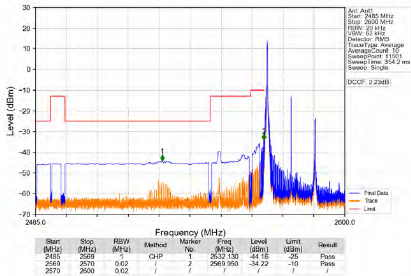
Band38_20MHz_16QAM_LCH_2580MHz_RB_1_0_NTNV
