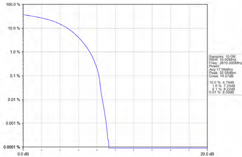
Band38_20MHz_QPSK_HCH_2610MHz_RB_100_0_NTNV
