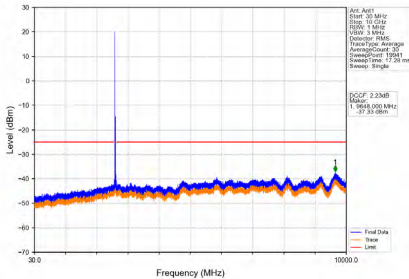
Band38_20MHz_QPSK_HCH_2610MHz_RB_1_0_NTNV
