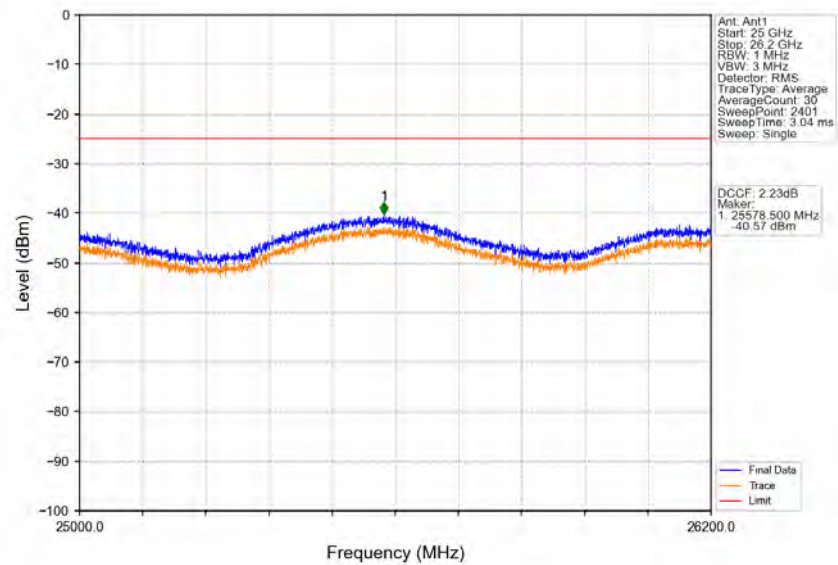
Band38_5MHz_QPSK_HCH_2617.5MHz_RB_1_24_NTNV
