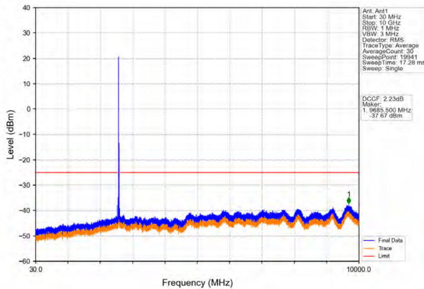
Band38_20MHz_16QAM_MCH_2595MHz_RB_1_0_NTNV
