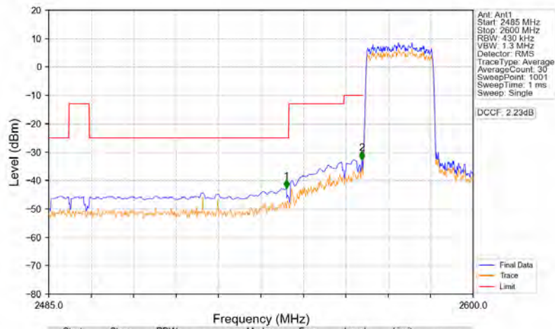
Band38_20MHz_16QAM_LCH_2580MHz_RB_100_0_NTNV
