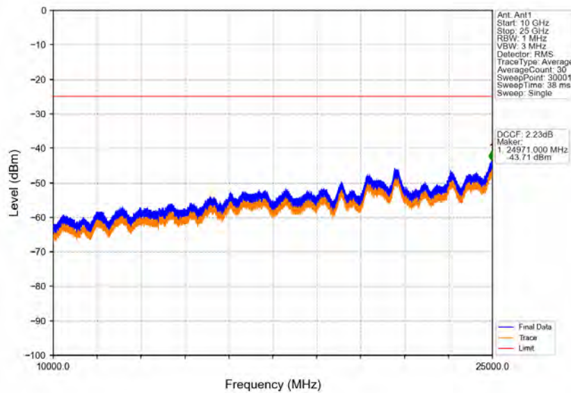
Band38_20MHz_16QAM_MCH_2595MHz_RB_1_0_NTNV
