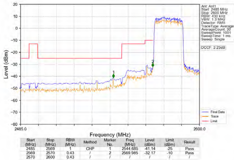
Band38_20MHz_QPSK_LCH_2580MHz_RB_100_0_NTNV
