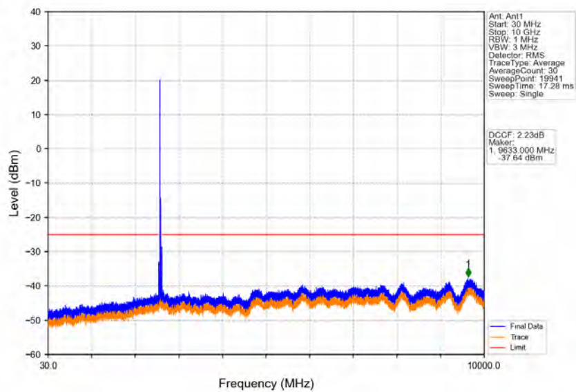
Band38_20MHz_QPSK_MCH_2595MHz_RB_1_0_NTNV
