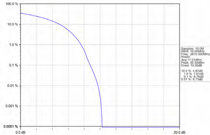
Band38_20MHz_16QAM_HCH_2610MHz_RB_100_0_NTNV
