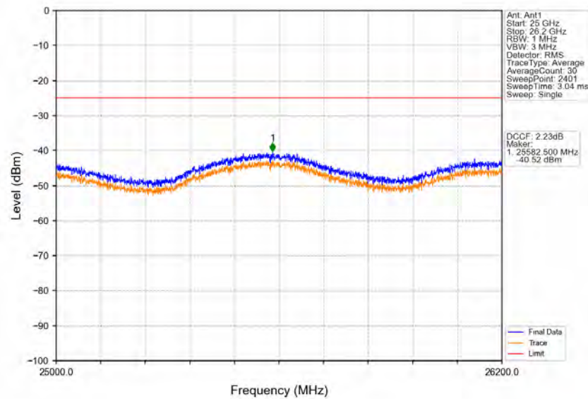
Band38_5MHz_QPSK_LCH_2572.5MHz_RB_1_0_NTNV
