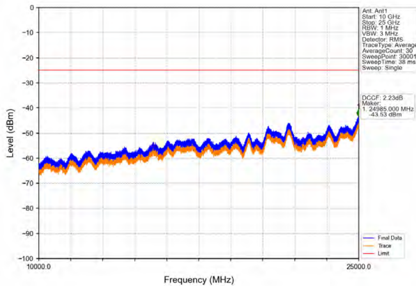
Band38_20MHz_16QAM_LCH_2580MHz_RB_1_0_NTNV
