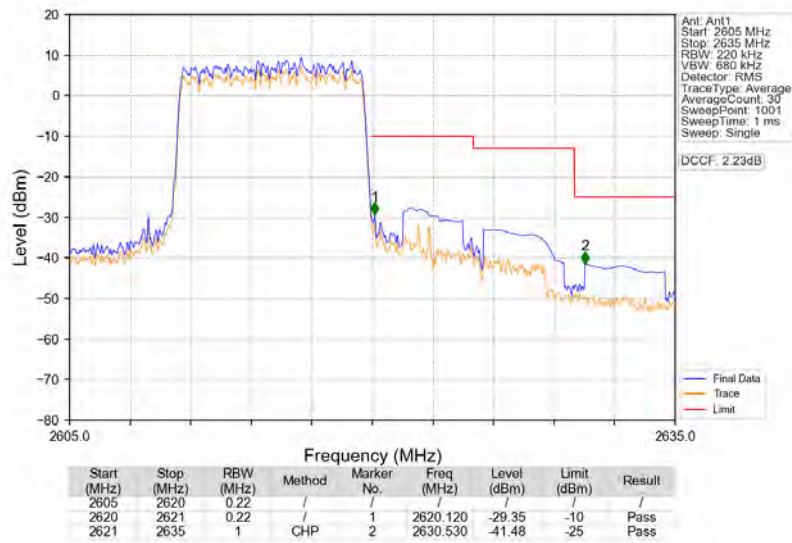
Band38_10MHz_QPSK_HCH_2615MHz_RB_50_0_NTNV
