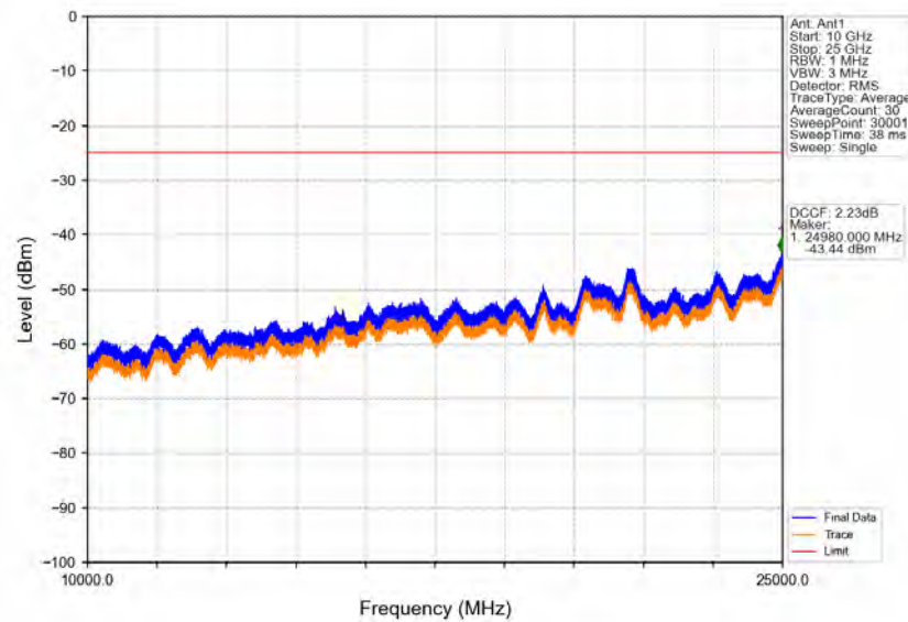
Band38_20MHz_QPSK_LCH_2580MHz_RB_1_0_NTNV
