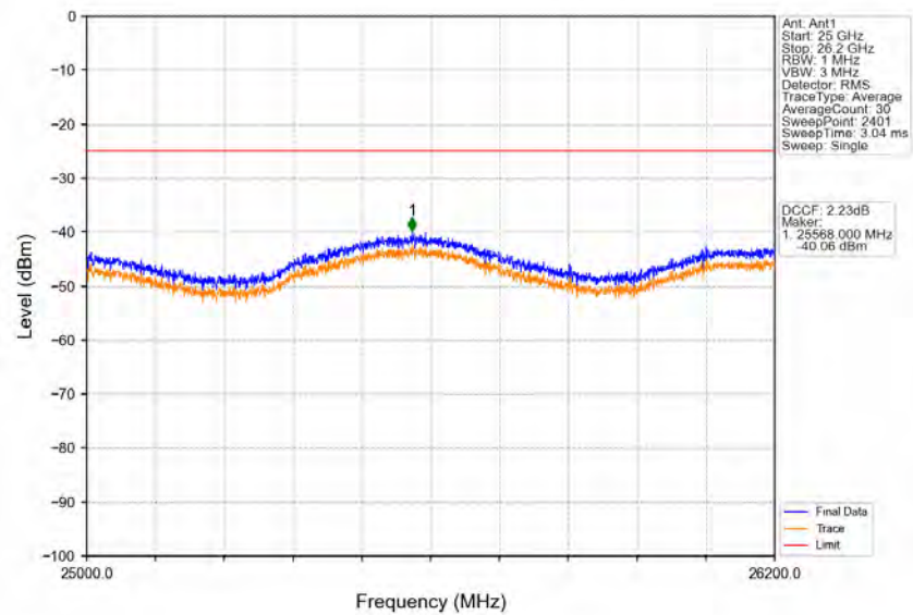
Band38_20MHz_16QAM_HCH_2610MHz_RB_1_0_NTNV
