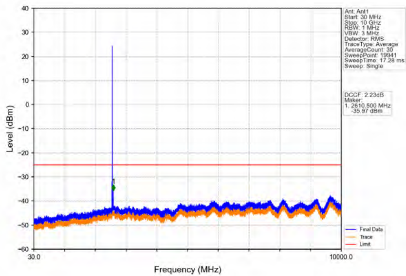
Band38_10MHz_QPSK_LCH_2575MHz_RB_1_0_NTNV
