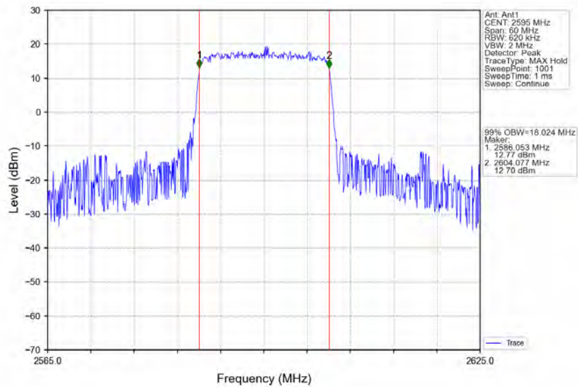
Band38_20MHz_16QAM_MCH_2595MHz_RB_100_0_NTNV
