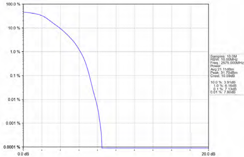
Band38_10MHz_QPSK_LCH_2575MHz_RB_50_0_NTNV
