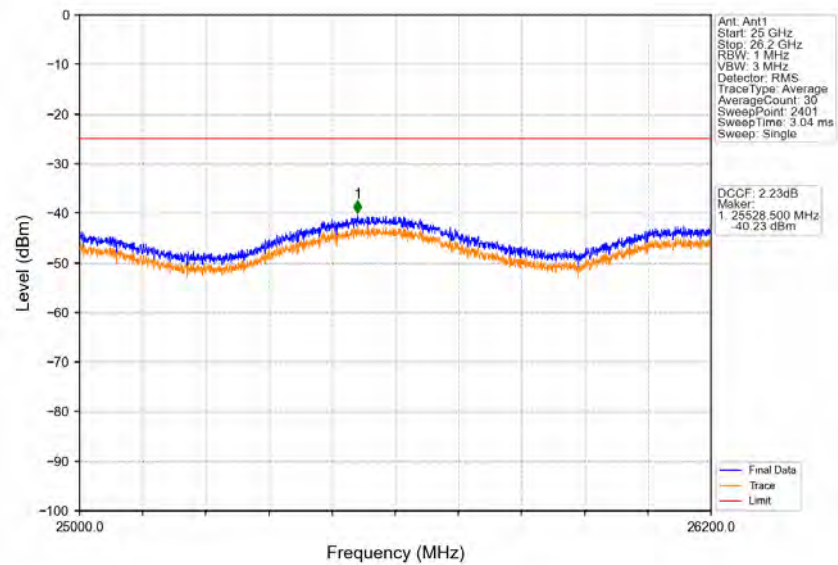
Band38_10MHz_QPSK_HCH_2615MHz_RB_1_49_NTNV
