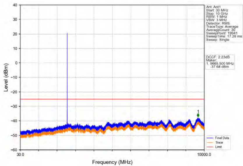
Band38_5MHz_QPSK_LCH_2572.5MHz_RB_1_0_NTNV
