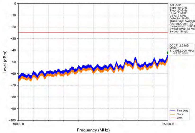
Band38_20MHz_QPSK_HCH_2610MHz_RB_1_0_NTNV
