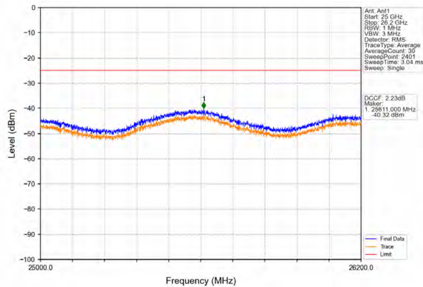
Band38_20MHz_QPSK_LCH_2580MHz_RB_1_0_NTNV
