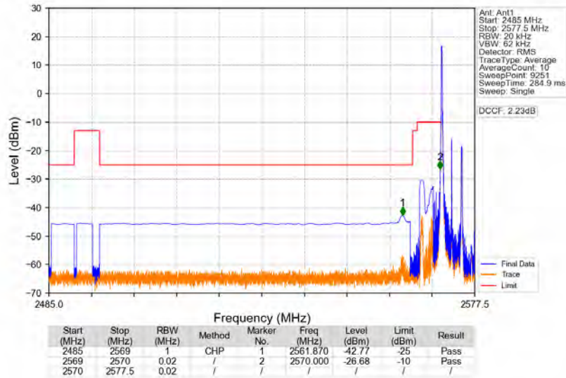
Band38_5MHz_QPSK_LCH_2572.5MHz_RB_1_0_NTNV
