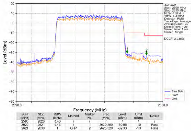
Band38_20MHz_QPSK_HCH_2610MHz_RB_100_0_NTNV
