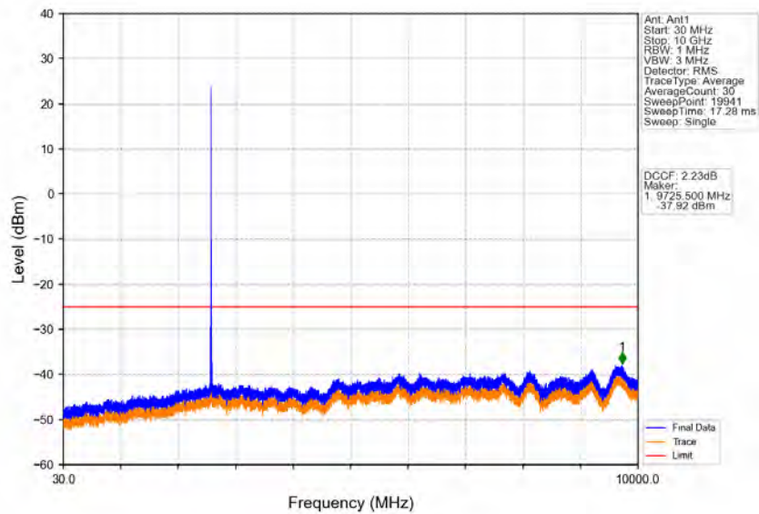
Band38_10MHz_QPSK_MCH_2595MHz_RB_1_0_NTNV
