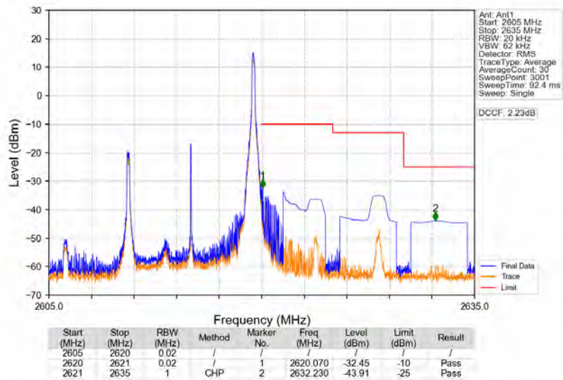
Band38_10MHz_QPSK_HCH_2615MHz_RB_1_49_NTNV
