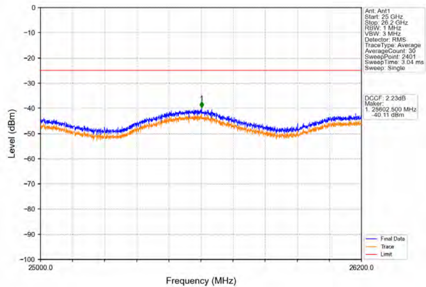
Band38_20MHz_64QAM_HCH_2610MHz_RB_1_99_NTNV
