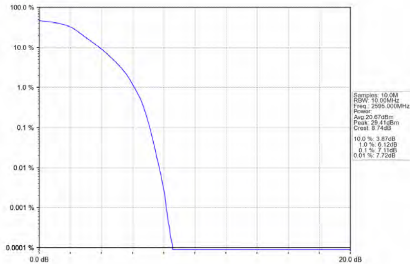
Band38_10MHz_QPSK_MCH_2595MHz_RB_50_0_NTNV
