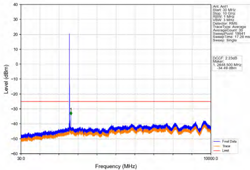
Band38_20MHz_16QAM_LCH_2580MHz_RB_1_0_NTNV
