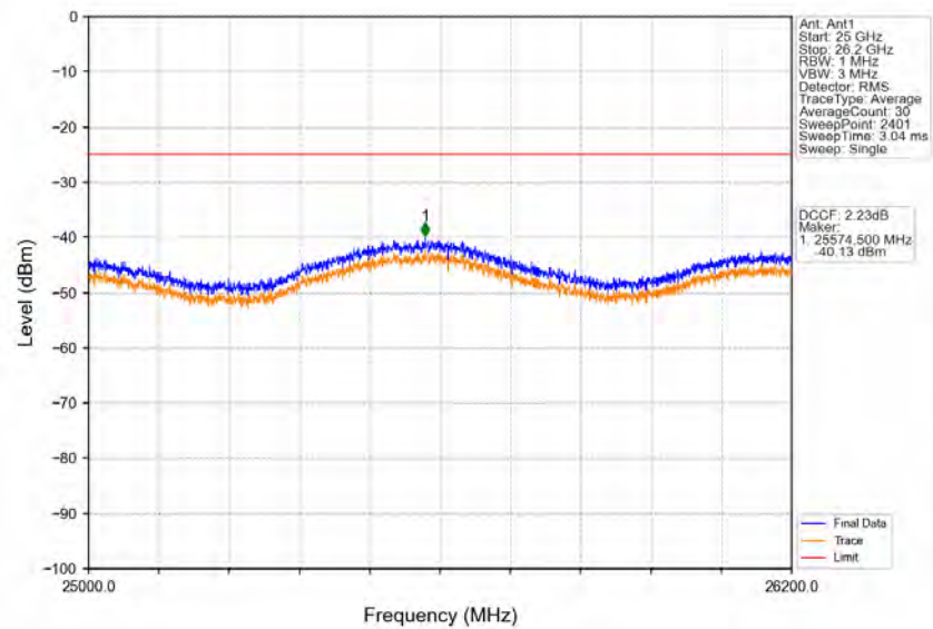
Band38_20MHz_QPSK_HCH_2610MHz_RB_1_99_NTNV
