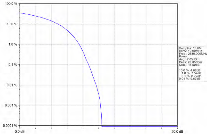
Band38_20MHz_16QAM_LCH_2580MHz_RB_100_0_NTNV
