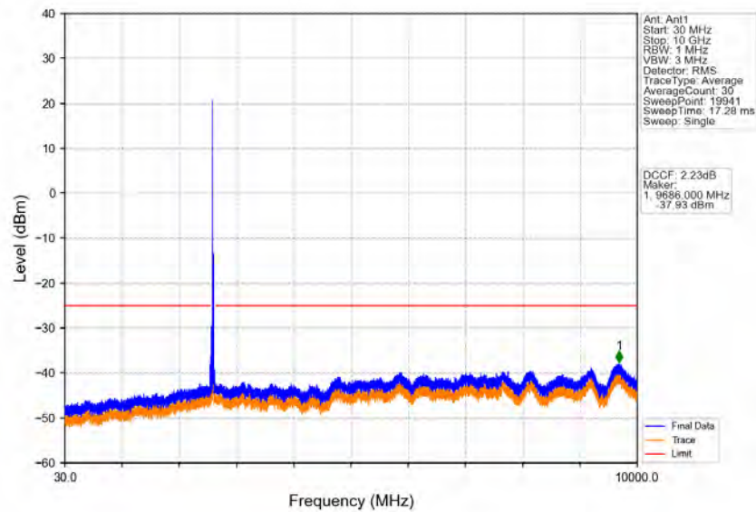
Band38_20MHz_16QAM_HCH_2610MHz_RB_1_0_NTNV
