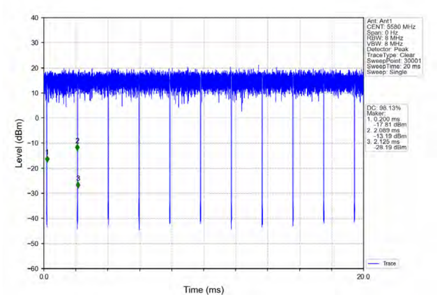
802.11n(HT20) MCH_5580MHz_Ant1_NTNV
