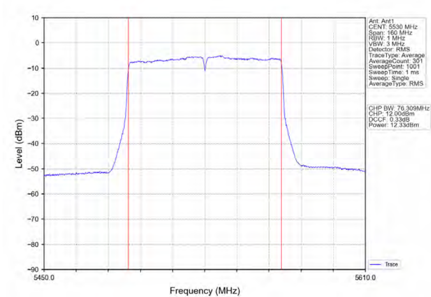
802.11ac(VHT80) LCH_5530MHz_Ant1_NTNV
