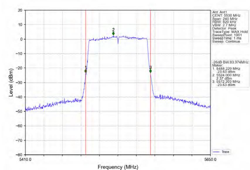
802.11ac(VHT80) LCH_5530MHz_Ant1_NTNV
