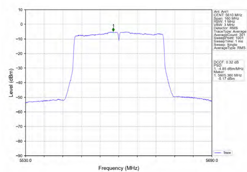
802.11ac(VHT80) HCH 5610MHz Ant1 NTNV
