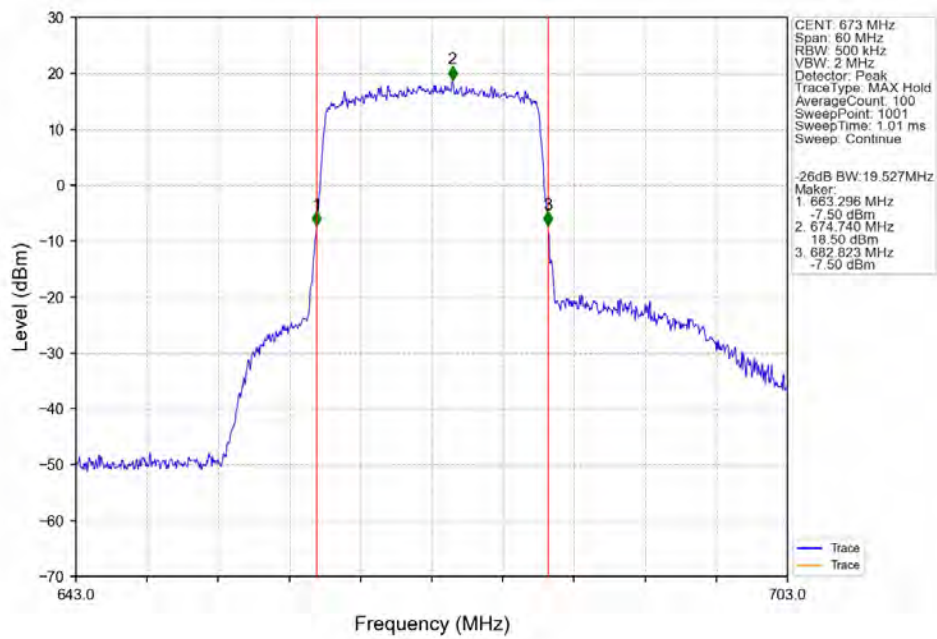
Band71_20MHz_QPSK_LCH_673MHz_RB_100_0_NTNV
