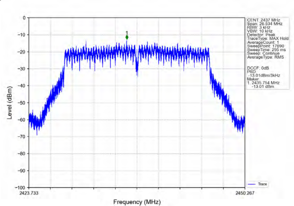
802.11n(HT20)_MCH_2437MHz_Ant1 (SISO)_NTNV
