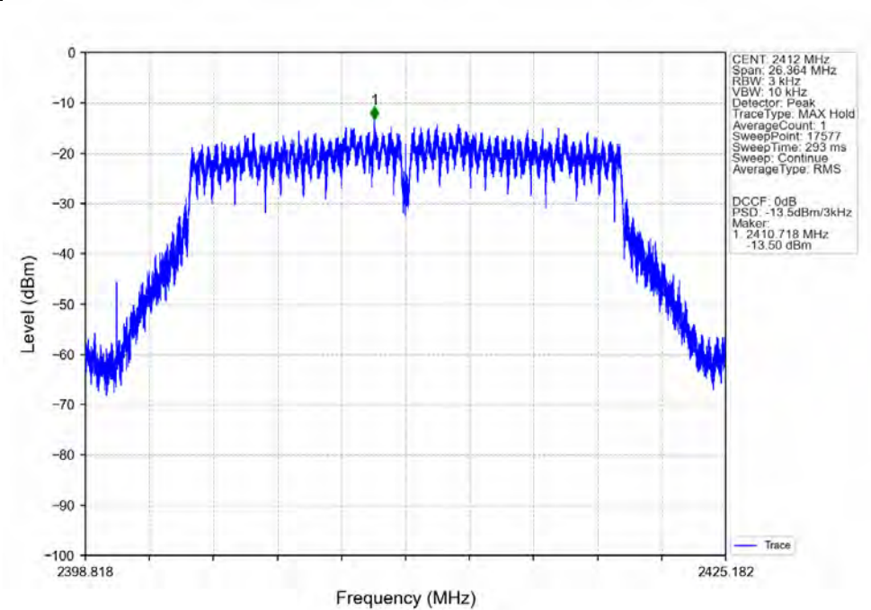
802.11n(HT20)_LCH_2412MHz_Ant1 (SISO)_NTNV
