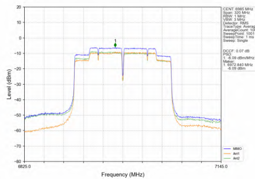
802.11ac(VHT160)_MCH_6985MHz_MIMO_NTNV
