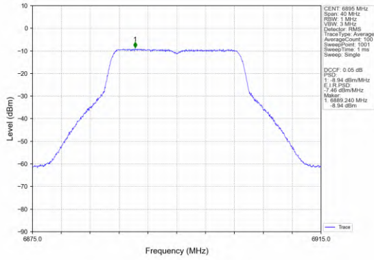
802.11n(HT20)_LCH_6895MHz_MIMO_NTNV
