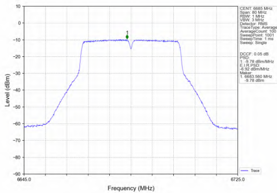
802.11n(HT40)_MCH_6685MHz_Ant2_NTNV
