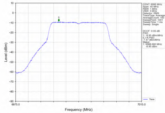
802.11n(HT20)_MCH_6995MHz_MIMO_NTNV
