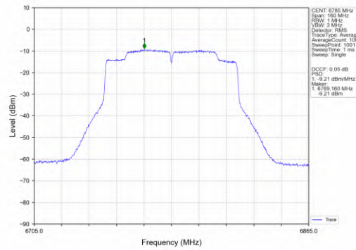
802.11ac(VHT80)_HCH_6785MHz_MIMO_NTNV
