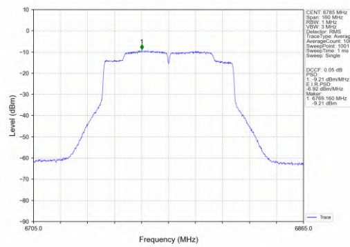
802.11ac(VHT80)_HCH_6785MHz_MIMO_NTNV
