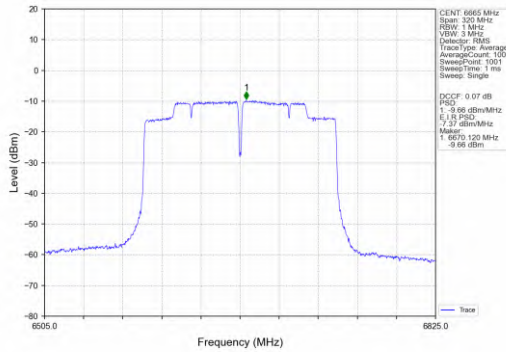
802.11ac(VHT160)_MCH_6665MHz_MIMO_NTNV
