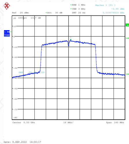
11AC80SISO-Ant1-5530--4.49-0.50-0.00-0.00
