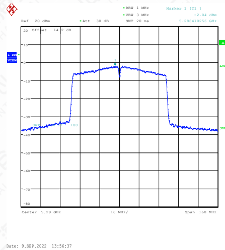
11AC80SISO-Ant1-5290--2.54-0.50-0.00-0.00
