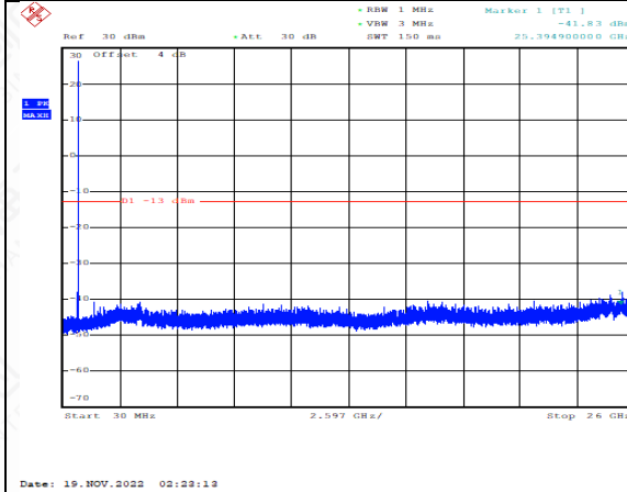
FDD17_HighRange_5MHz_30MHz~26GHz
