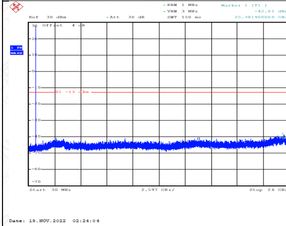
FDD17_HighRange_5MHz_30MHz~26GHz
