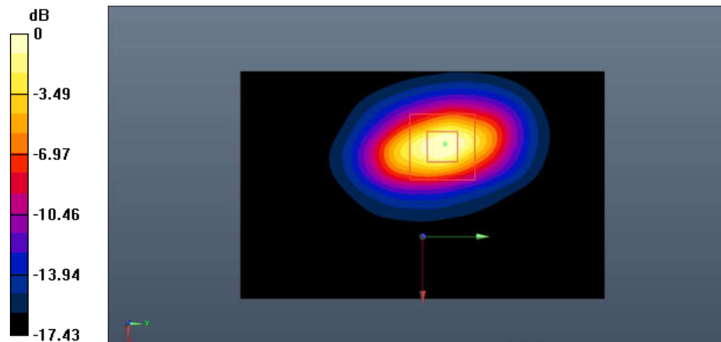
Fig.B.4. Check 1750MHz 50mW
