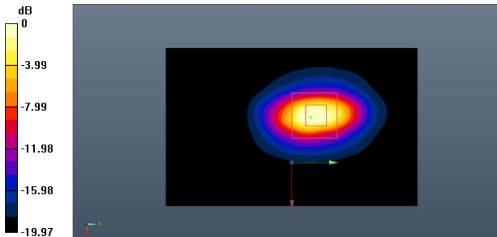
Fig.B.8. Check 2300MHz 50mW
