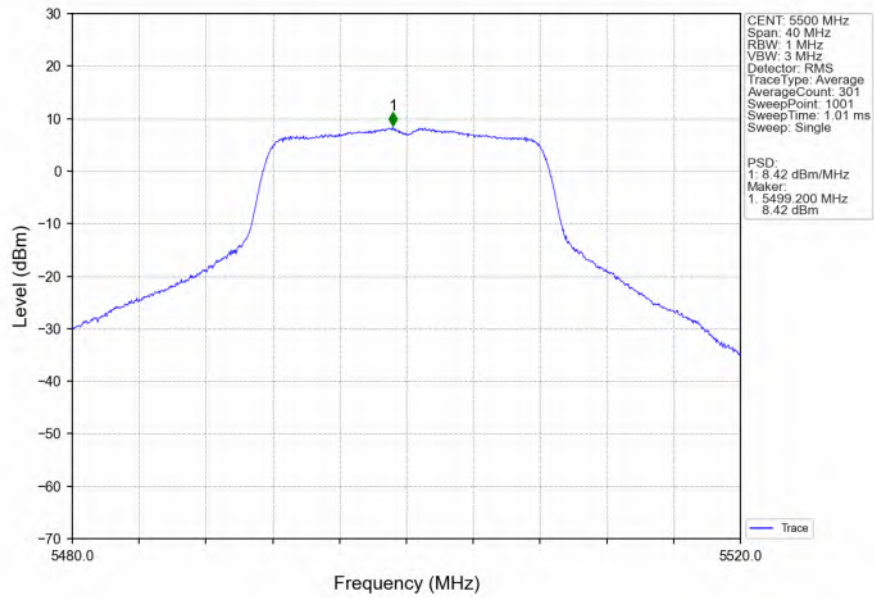
802.11a_LCH_5500MHz_Ant1_NTNV
