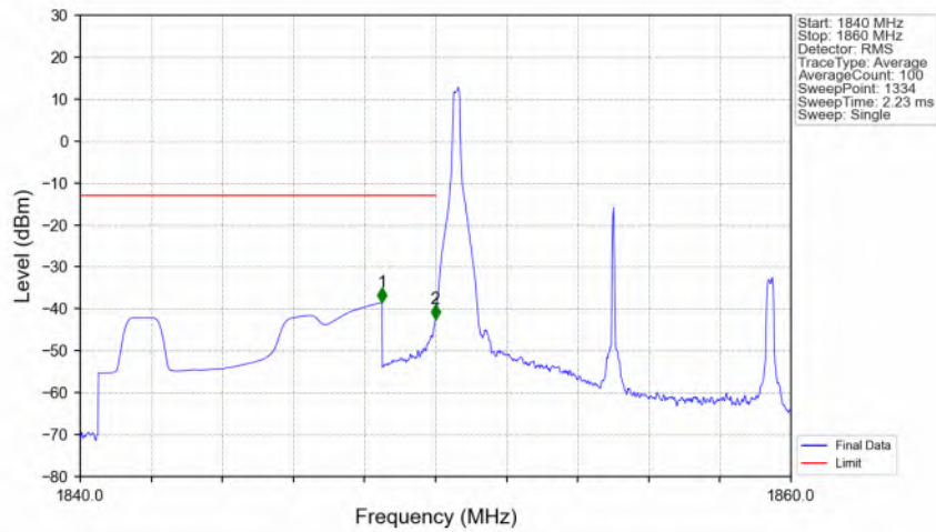
Band25_10MHz_QPSK_LCH_1855MHz_RB_1_0_NTNV
