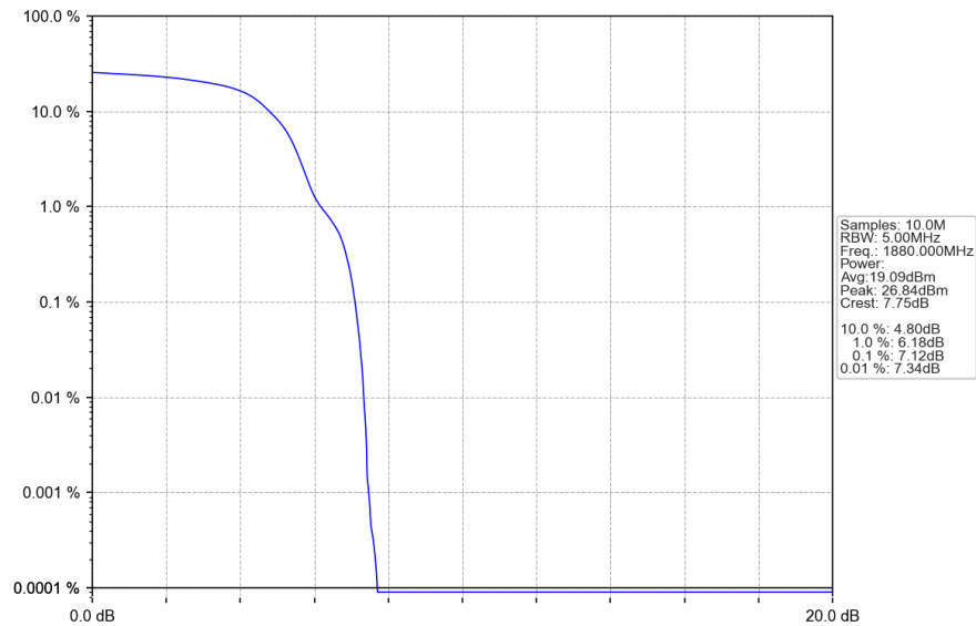
Band2_HSUPA_MCH_1880MHz_Subtest 1_NTNV
