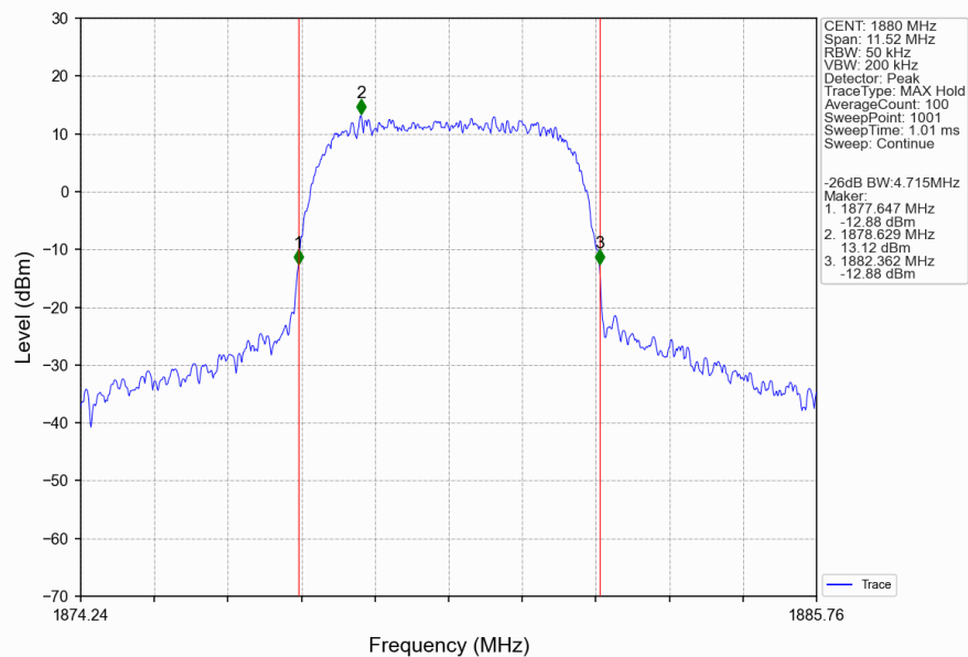
Band2_HSUPA_MCH_1880MHz_Subtest 1_NTNV
