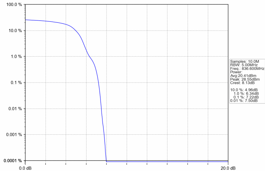
Band5_HSUPA_MCH_836.6MHz_Subtest 1_NTNV
