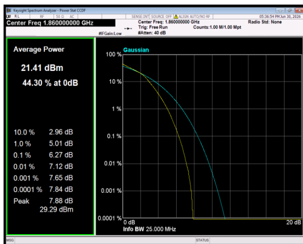
Band2 16QAM BW=20MHz Channel=18700 RB Size=100 Position=#0
