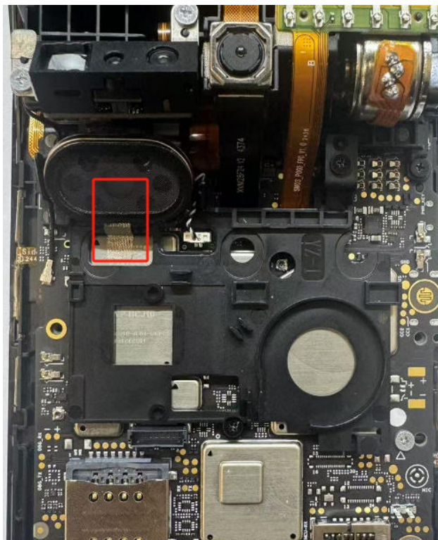
喇叭贴导电布与主板接地
