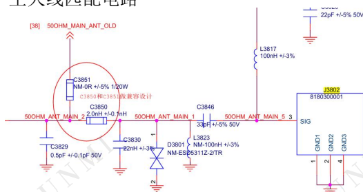
主天线匹配电路
