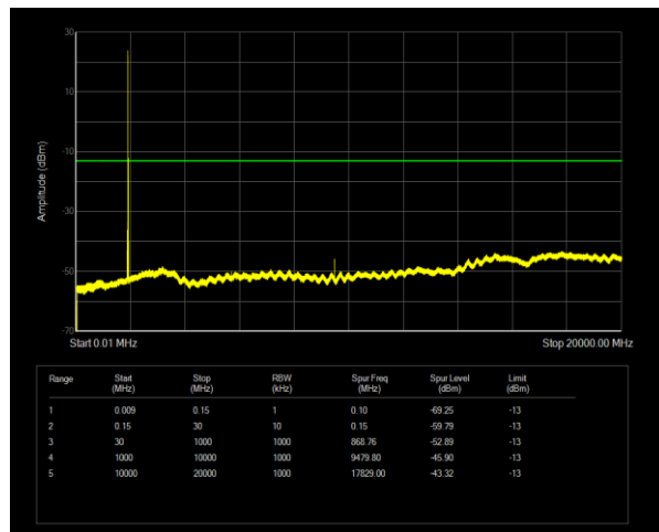
Band2 QPSK BW=15MHz Channel=19125 RB Size=1 Position=#0
