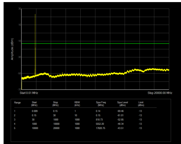
Band2 QPSK BW=10MHz Channel=18650 RB Size=1 Position=#0
