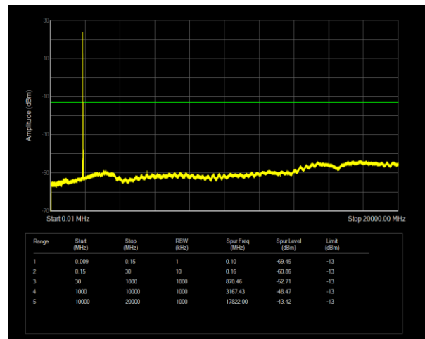
Band2 QPSK BW=20MHz Channel=18700 RB Size=1 Position=#0
