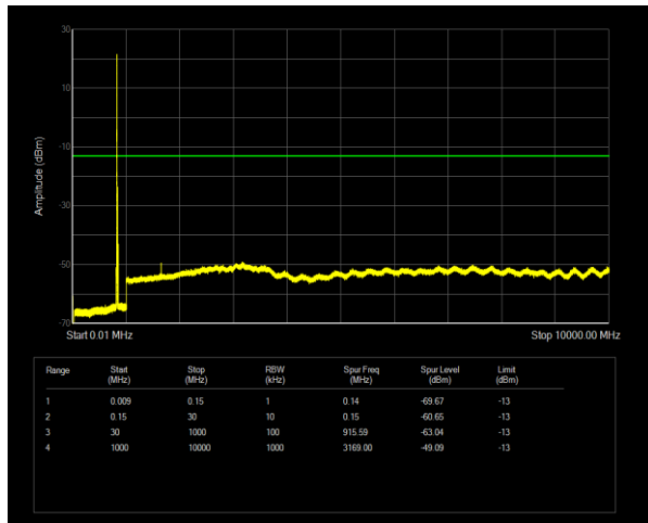
Band26(824-849) QPSK BW=15MHz Channel=26865 RB Size=1 Position=#0
