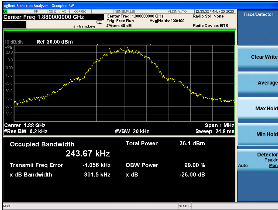
OCB\GSM1900 M
