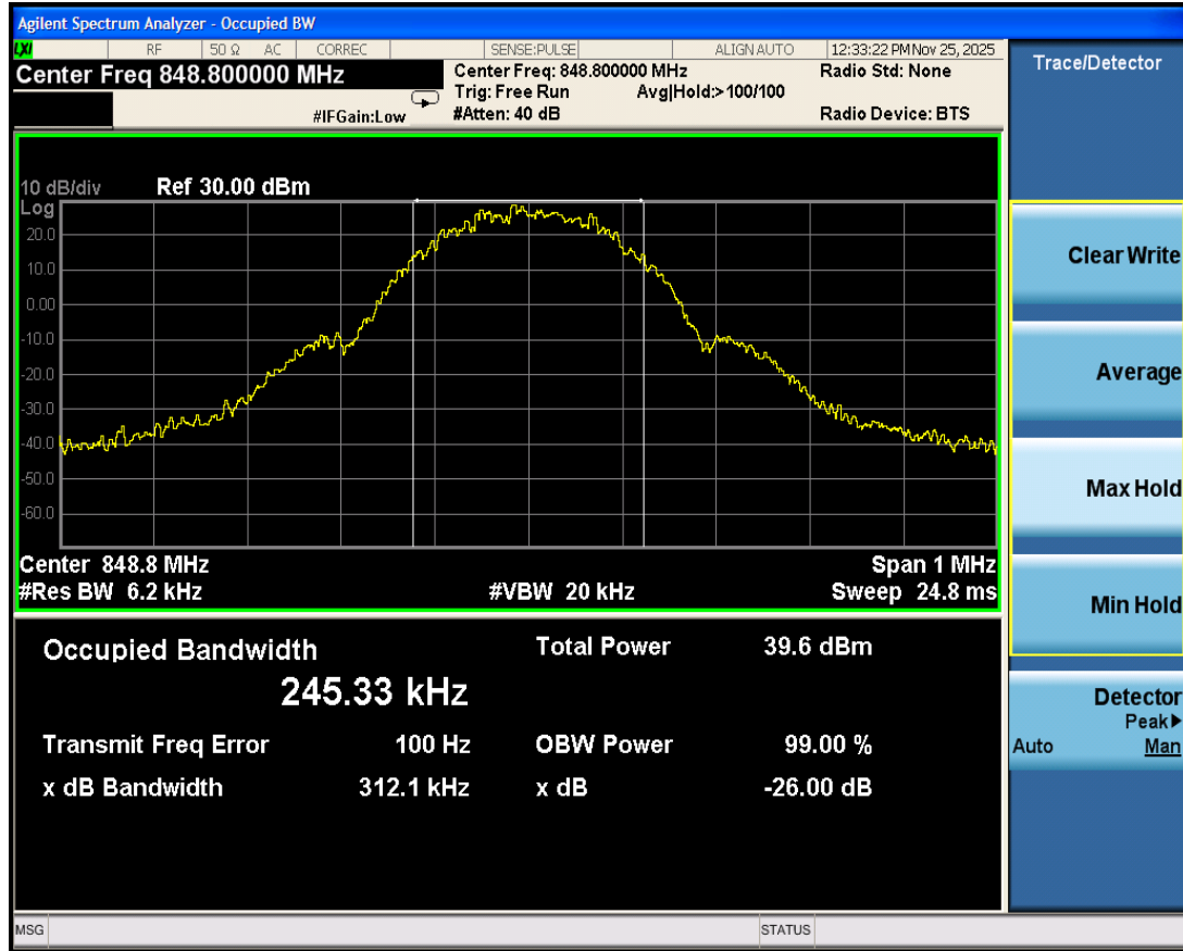
OCB\GSM850 H
