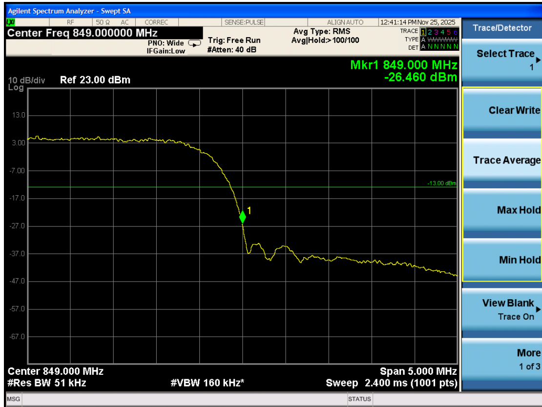
Band edge\WCDMA B5\H
