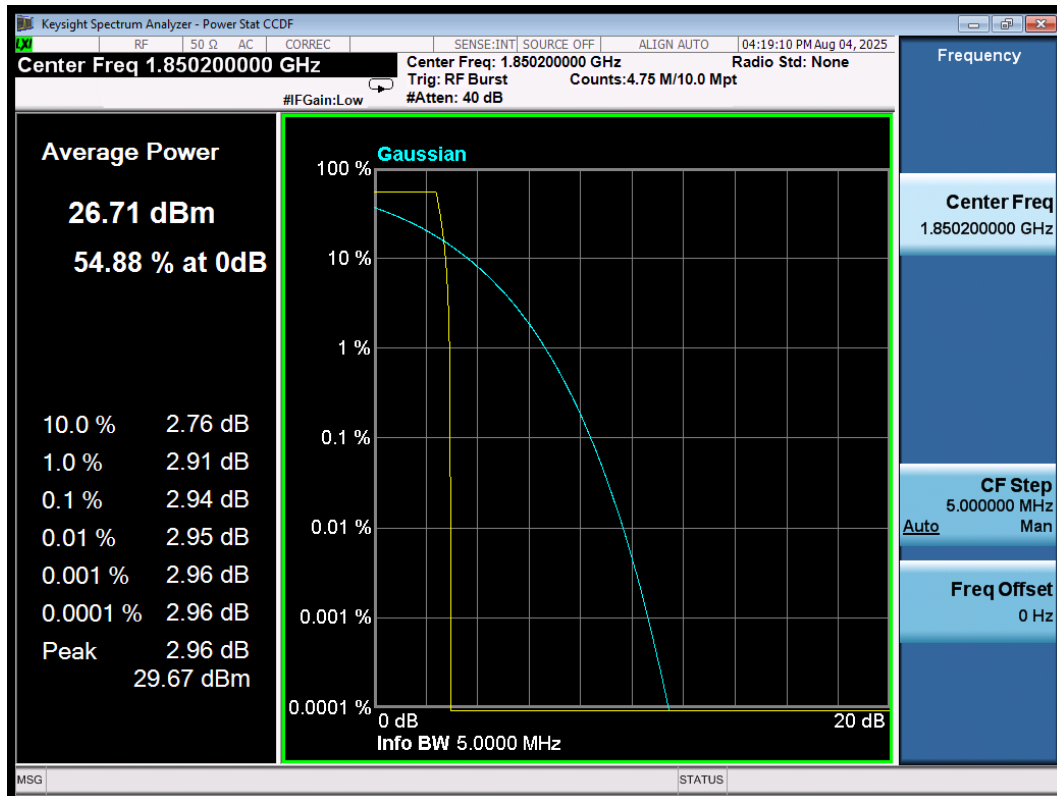
PAPR\GSM1900\GPRS\L
