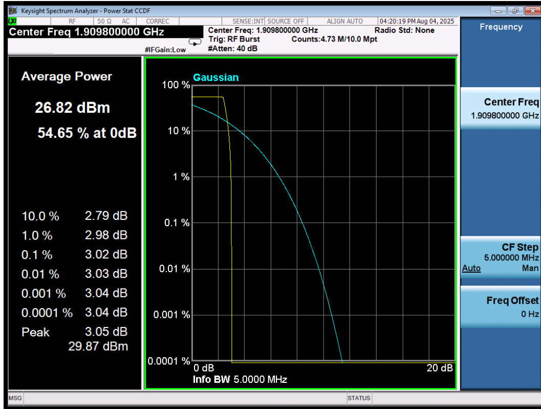
PAPR\GSM1900\GPRS\H
