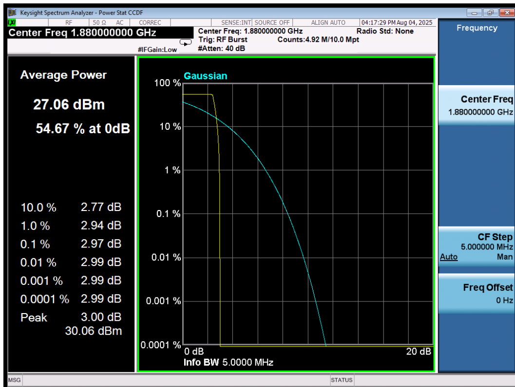
PAPR\GSM1900\GSM\
