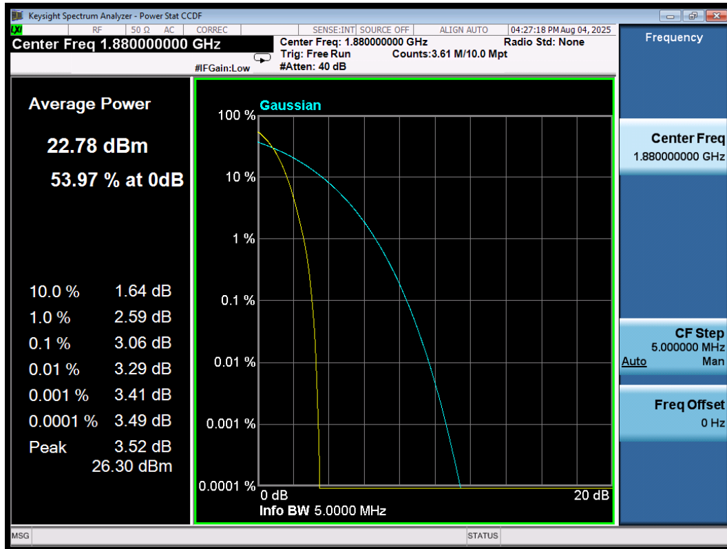
PAPR\B2\1M
