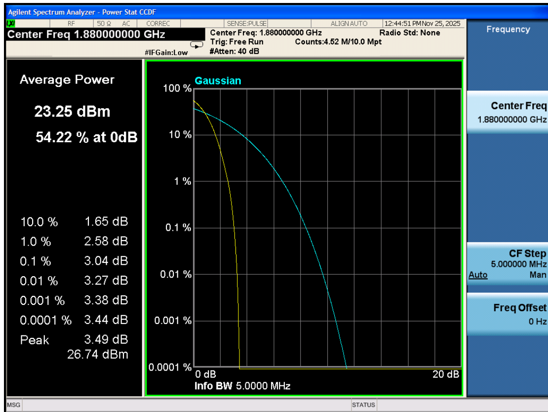
PAPR\WCDMA B2 M
