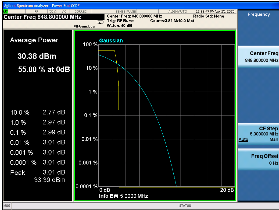
PAPR\GSM850 H
