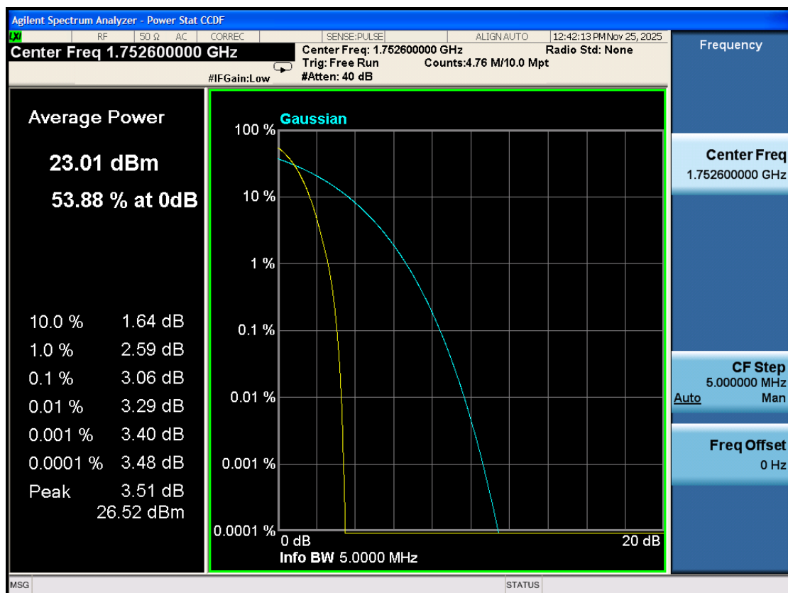
PAPR\WCDMA B4 H
