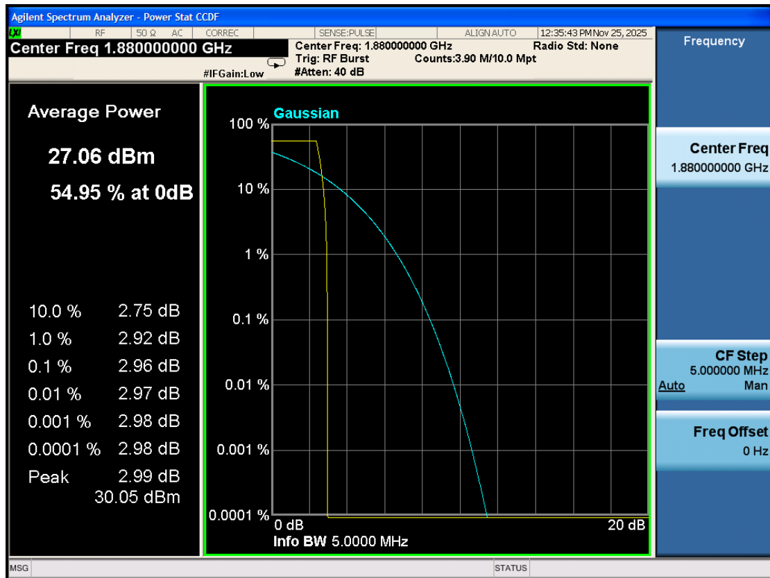
PAPR\GSM1900 M
