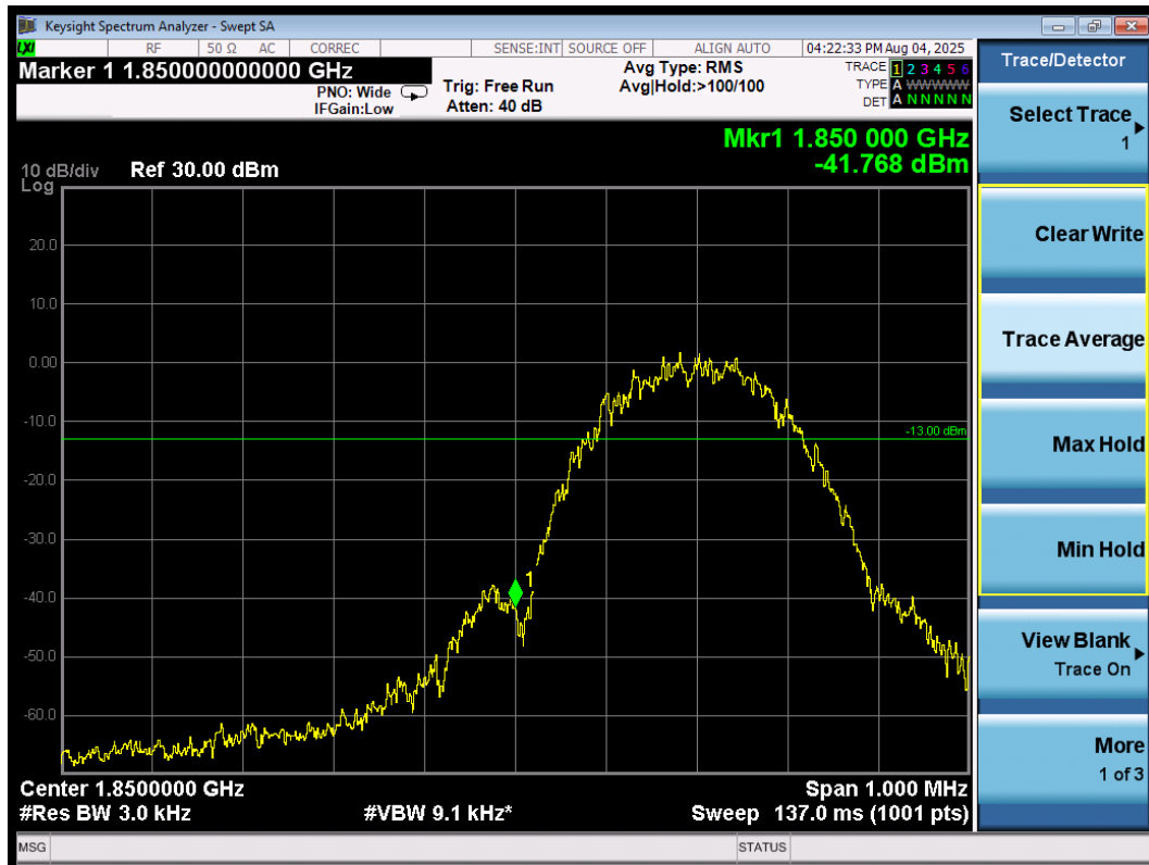
Band edge\GSM1900\EGPRS\L
