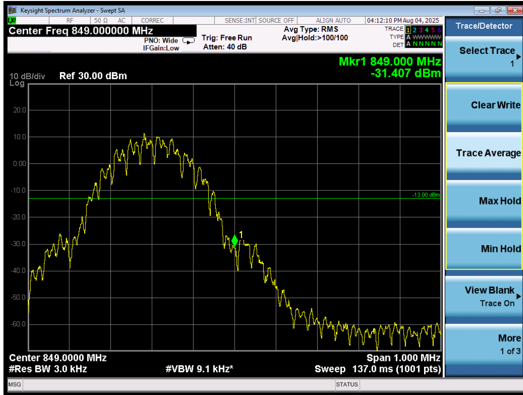
Band edge\GSM850\GPRS\H
