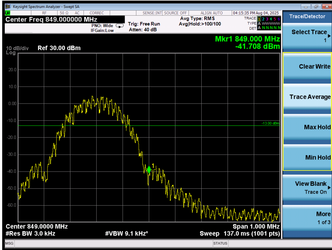
Band edge\GSM850\EGPRS\H
