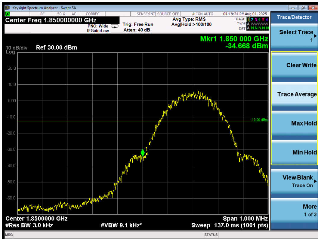
Band edge\GSM1900\GPRS\L
