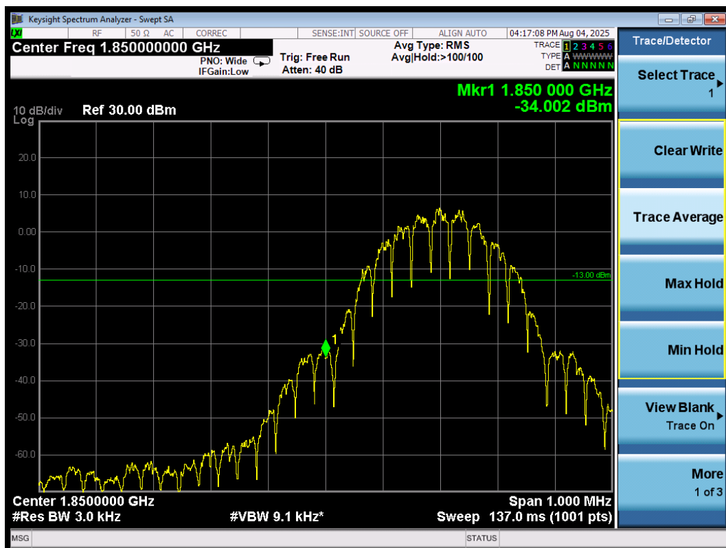
Band edge\GSM1900\GSM\L
