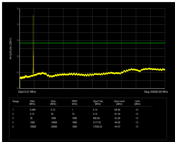
Band2 QPSK BW=20MHz Channel=18700 RB Size=1 Position=#0
