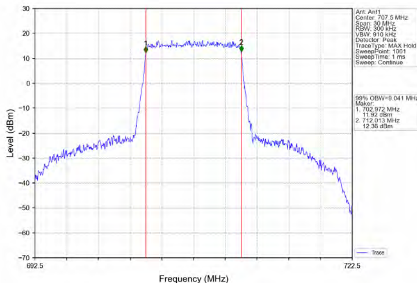
Band12_10MHz_QPSK_MCH_707.5MHz_RB_50_0_NTNV
