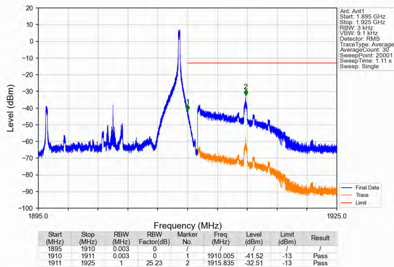
Band2_15MHz_QPSK_HCH_1902.5MHz_RB_1_74_NTNV
