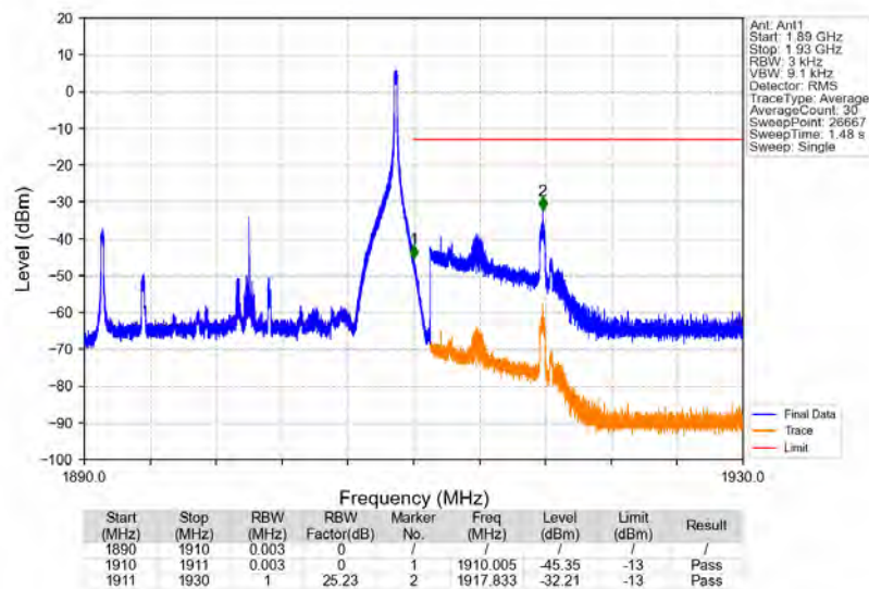
Band2_20MHz_QPSK_HCH_1900MHz_RB_1_99_NTNV
