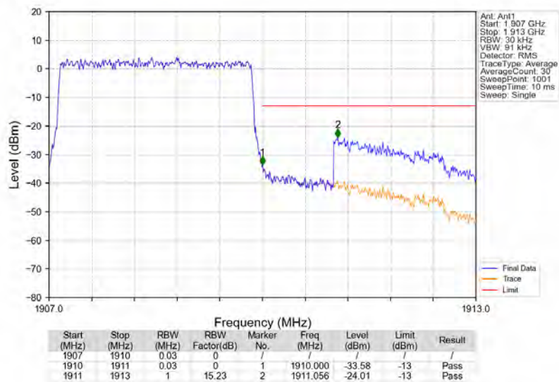
Band2_3MHz_QPSK_HCH_1908.5MHz_RB_15_0_NTNV
