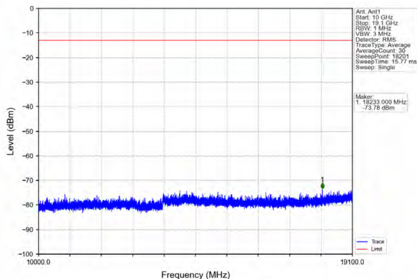
Band2_5MHz_QPSK_MCH_1880MHz_RB_1_0_NTNV
