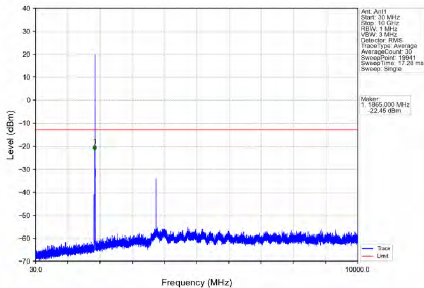
Band2_3MHz_16QAM_MCH_1880MHz_RB_1_0_NTNV
