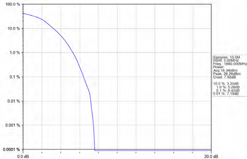
Band2_10MHz_16QAM_MCH_1880MHz_RB_50_0_NTNV
