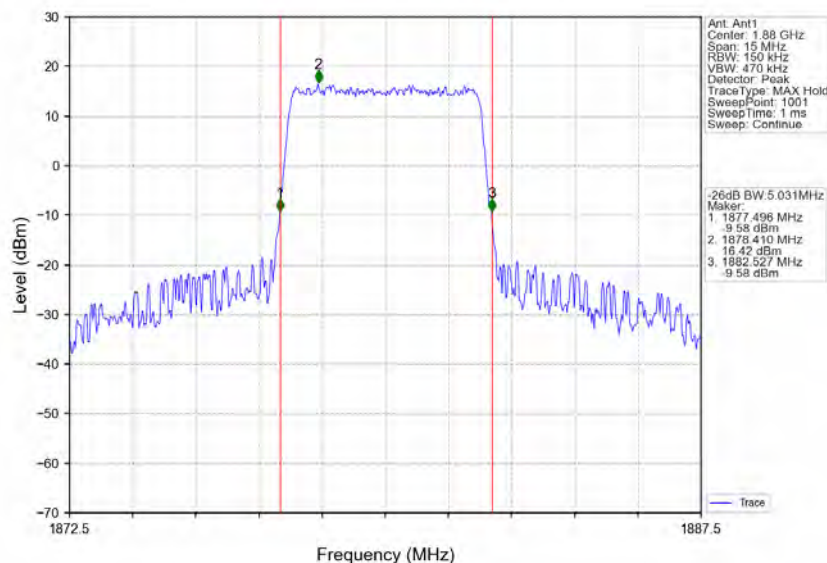
Band2_5MHz_QPSK_MCH_1880MHz_RB_25_0_NTNV
