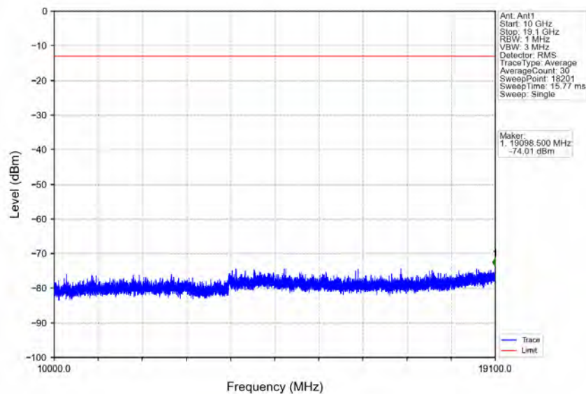
Band2_20MHz_QPSK_LCH_1860MHz_RB_100_0_NTNV
