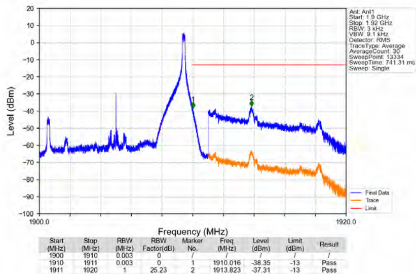
Band2_10MHz_16QAM_HCH_1905MHz_RB_1_49_NTNV
