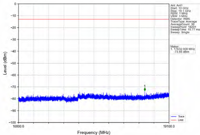
Band2_10MHz_QPSK_LCH_1855MHz_RB_50_0_NTNV
