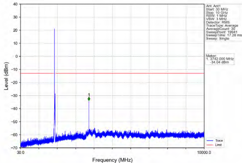
Band2_20MHz_QPSK_MCH_1880MHz_RB_1_0_NTNV
