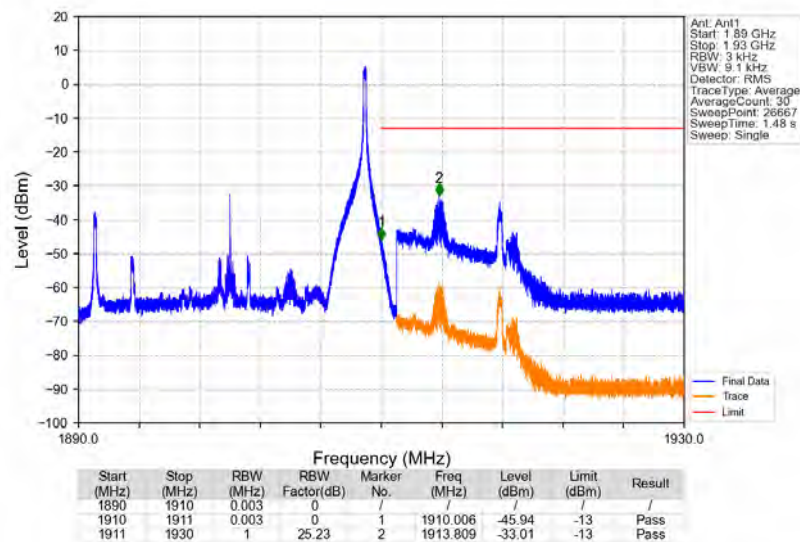
Band2_20MHz_16QAM_HCH_1900MHz_RB_1_99_NTNV
