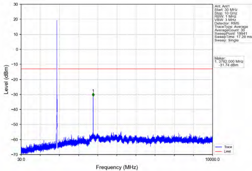
Band2_20MHz_16QAM_HCH_1900MHz_RB_1_0_NTNV
