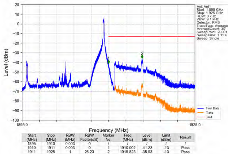
Band2_15MHz_16QAM_HCH_1902.5MHz_RB_1_74_NTNV
