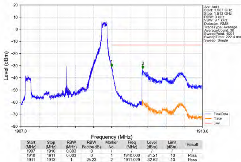
Band2_3MHz_QPSK_HCH_1908.5MHz_RB_1_14_NTNV
