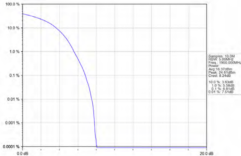
Band2_20MHz_QPSK_HCH_1900MHz_RB_100_0_NTNV
