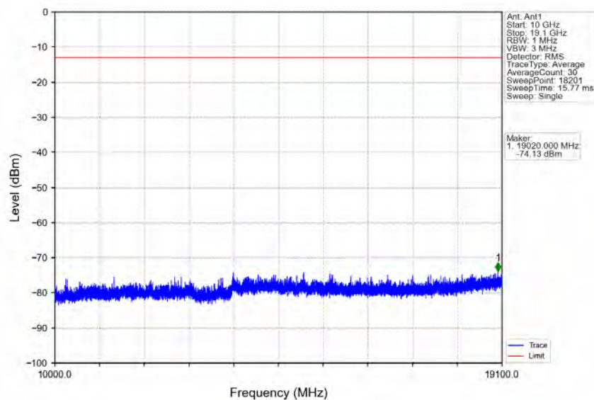
Band2_20MHz_16QAM_HCH_1900MHz_RB_1_0_NTNV
