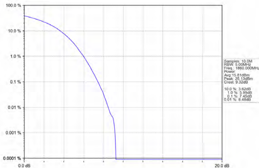
Band2_20MHz_16QAM_LCH_1860MHz_RB_100_0_NTNV
