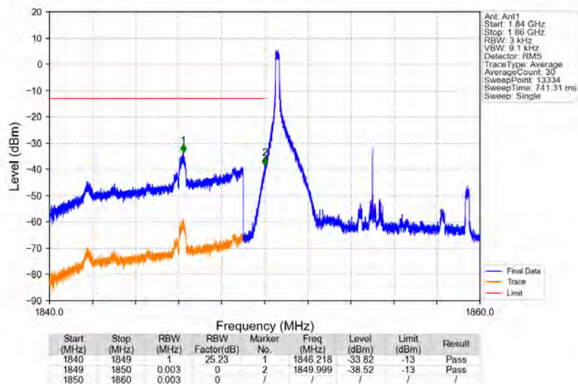
Band2_10MHz_16QAM_LCH_1855MHz_RB_1_0_NTNV
