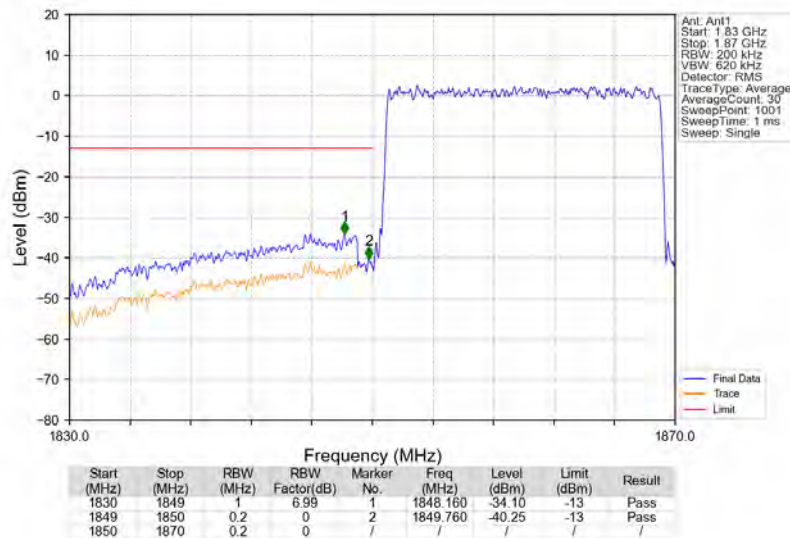
Band2_20MHz_16QAM_LCH_1860MHz_RB_100_0_NTNV
