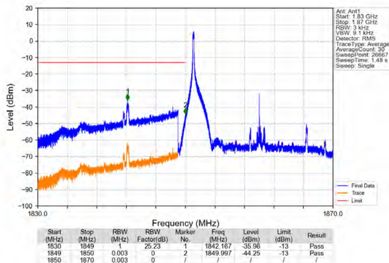
Band2_20MHz_16QAM_LCH_1860MHz_RB_1_0_NTNV
