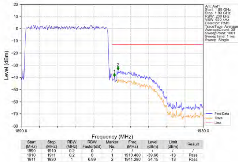
Band2_20MHz_16QAM_HCH_1900MHz_RB_100_0_NTNV
