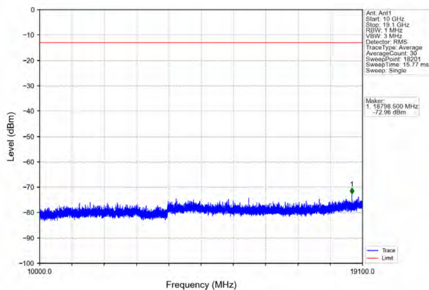
Band2_3MHz_16QAM_MCH_1880MHz_RB_1_0_NTNV
