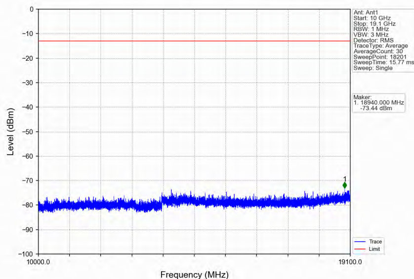
Band2_3MHz_QPSK_HCH_1908.5MHz_RB_1_0_NTNV
