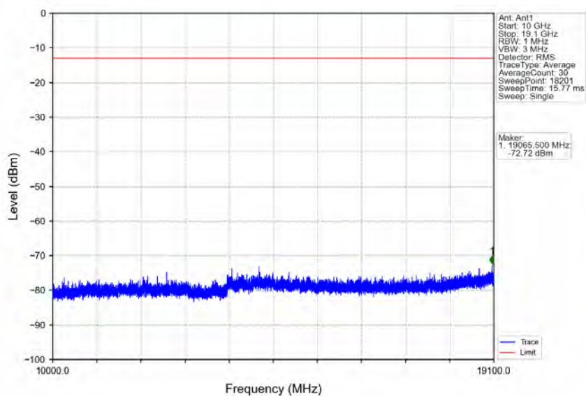
Band2_10MHz_QPSK_MCH_1880MHz_RB_1_0_NTNV
