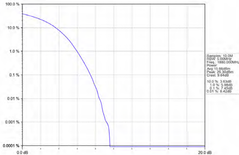
Band2_20MHz_16QAM_MCH_1880MHz_RB_100_0_NTNV
