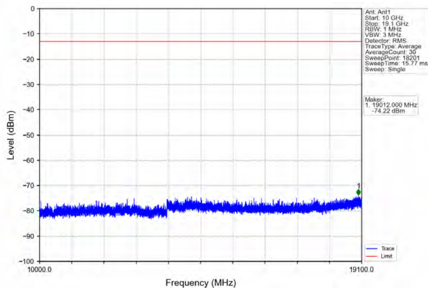
Band2_20MHz_QPSK_MCH_1880MHz_RB_1_0_NTNV
