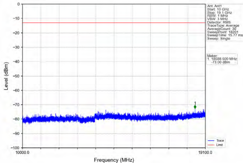
Band2_10MHz_16QAM_LCH_1855MHz_RB_50_0_NTNV
