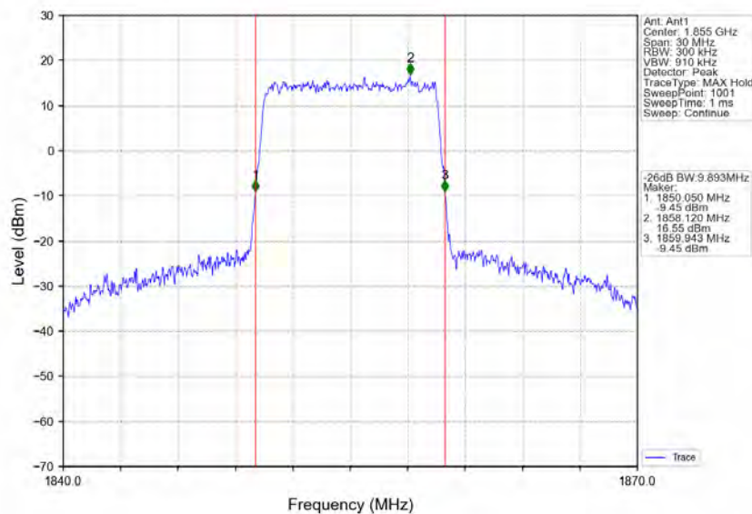
Band2_10MHz_16QAM_LCH_1855MHz_RB_50_0_NTNV
