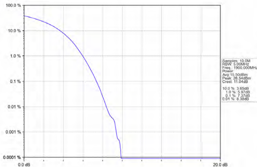
Band2_20MHz_16QAM_HCH_1900MHz_RB_100_0_NTNV
