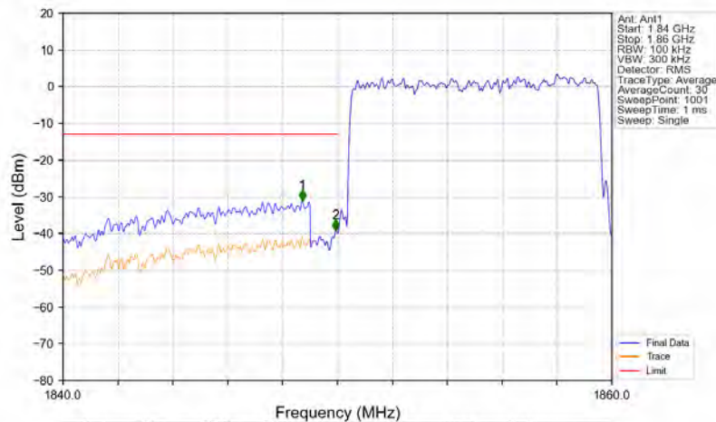
Band2_10MHz_16QAM_LCH_1855MHz_RB_50_0_NTNV
