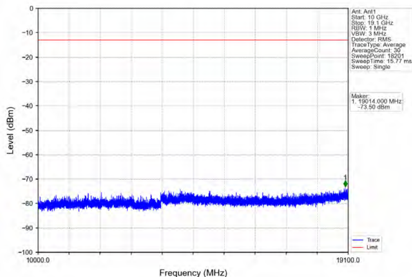
Band2_20MHz_QPSK_HCH_1900MHz_RB_1_0_NTNV
