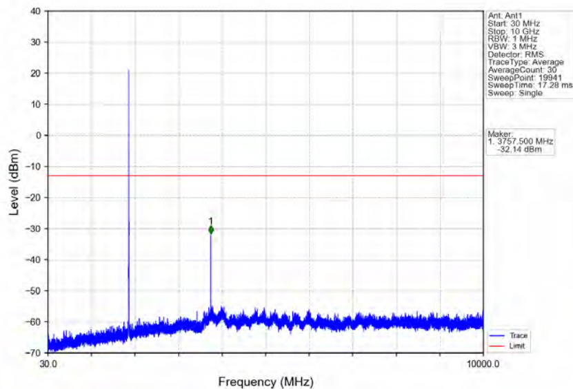
Band2_3MHz_QPSK_MCH_1880MHz_RB_1_0_NTNV
