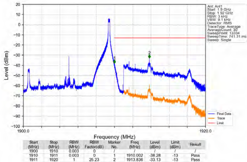
Band2_10MHz_QPSK_HCH_1905MHz_RB_1_49_NTNV
