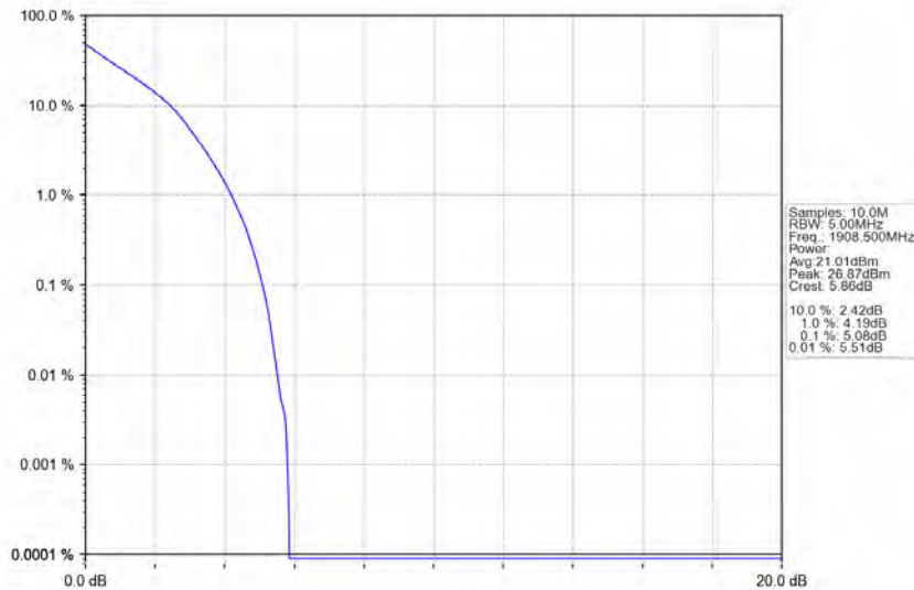
Band2_3MHz_QPSK_HCH_1908.5MHz_RB_15_0_NTNV
