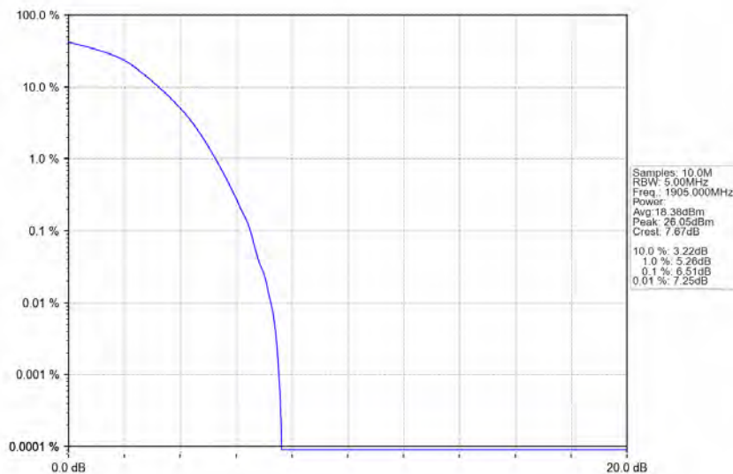
Band2_10MHz_16QAM_HCH_1905MHz_RB_50_0_NTNV
