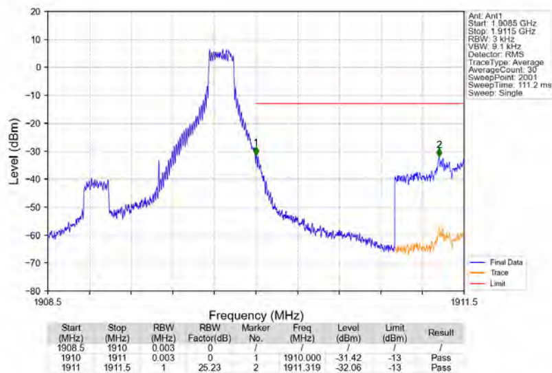
Band2_1.4MHz_QPSK_HCH_1909.3MHz_RB_1_5_NTNV
