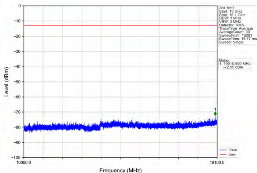
Band2_1.4MHz_QPSK_HCH_1909.3MHz_RB_1_0_NTNV
