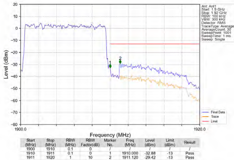
Band2_10MHz_QPSK_HCH_1905MHz_RB_50_0_NTNV
