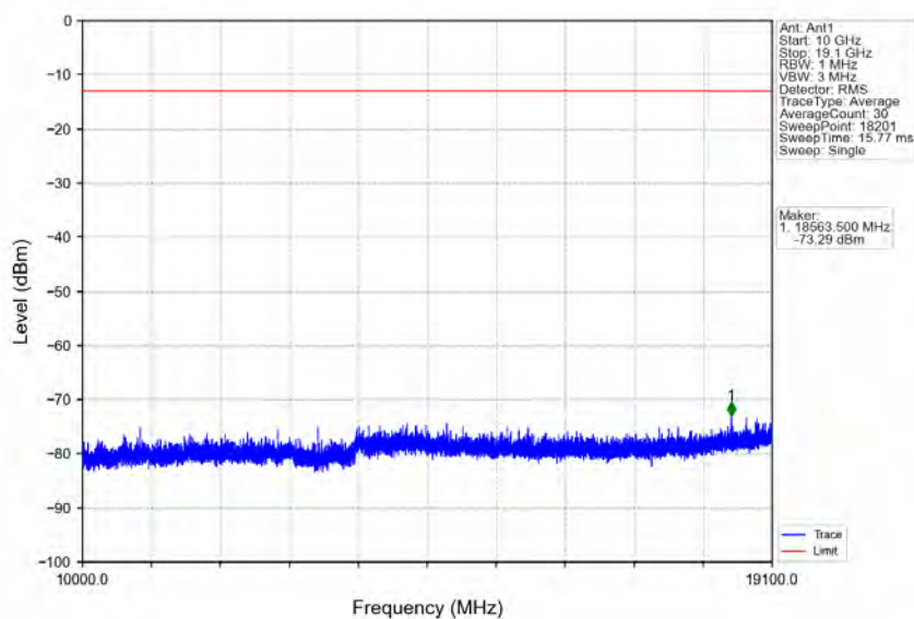
Band2_15MHz_QPSK_MCH_1880MHz_RB_1_0_NTNV
