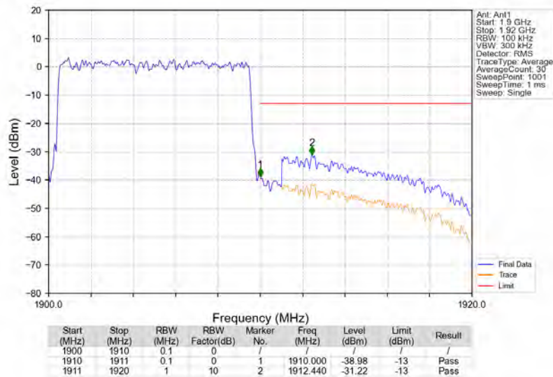
Band2_10MHz_16QAM_HCH_1905MHz_RB_50_0_NTNV
