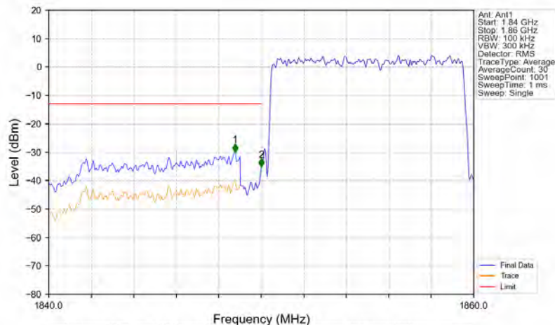
Band2_10MHz_QPSK_LCH_1855MHz_RB_50_0_NTNV
