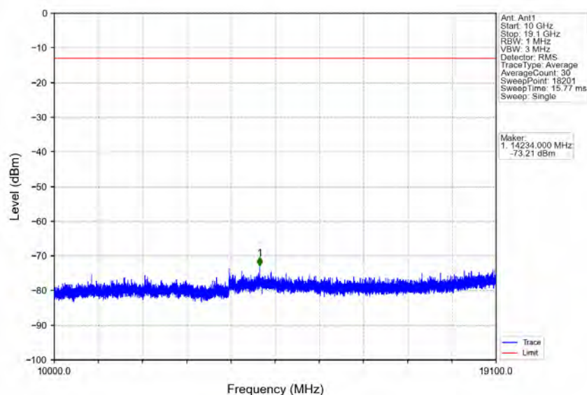
Band2_3MHz_QPSK_MCH_1880MHz_RB_1_0_NTNV
