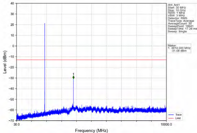
Band2_3MHz_QPSK_HCH_1908.5MHz_RB_1_0_NTNV
