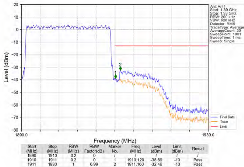
Band2_20MHz_QPSK_HCH_1900MHz_RB_100_0_NTNV
