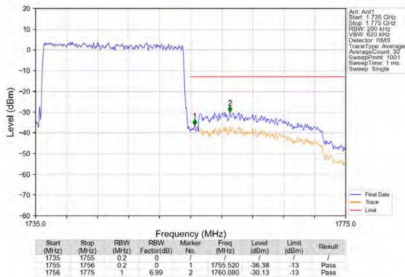
Band4_20MHz_QPSK_HCH_1745MHz_RB_100_0_NTNV
