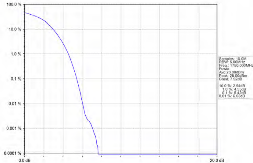
Band4_10MHz_QPSK_HCH_1750MHz_RB_50_0_NTNV
