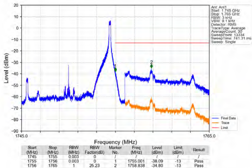
Band4_10MHz_QPSK_HCH_1750MHz_RB_1_49_NTNV
