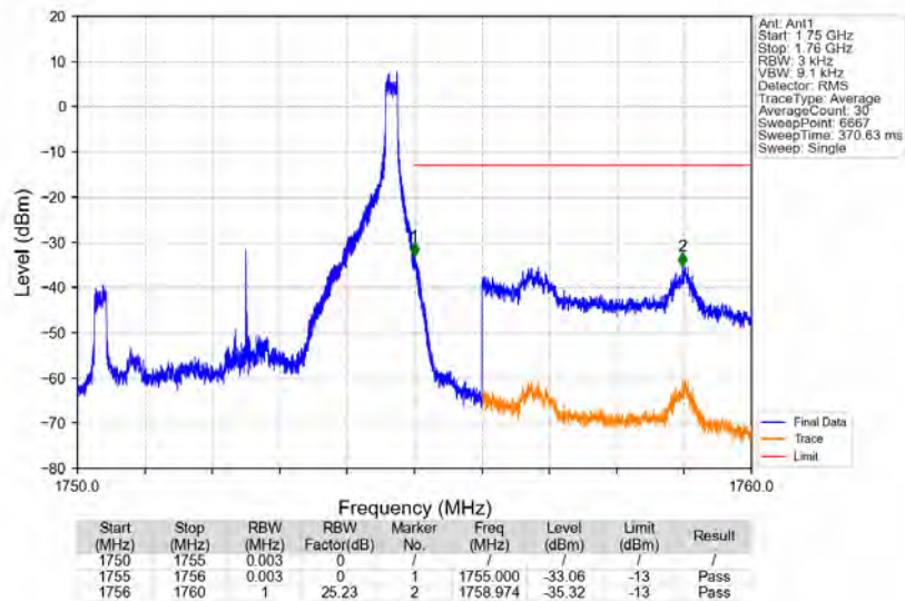
Band4 5MHz QPSK HCH 1752.5MHz_RB_1_24_NTNV
