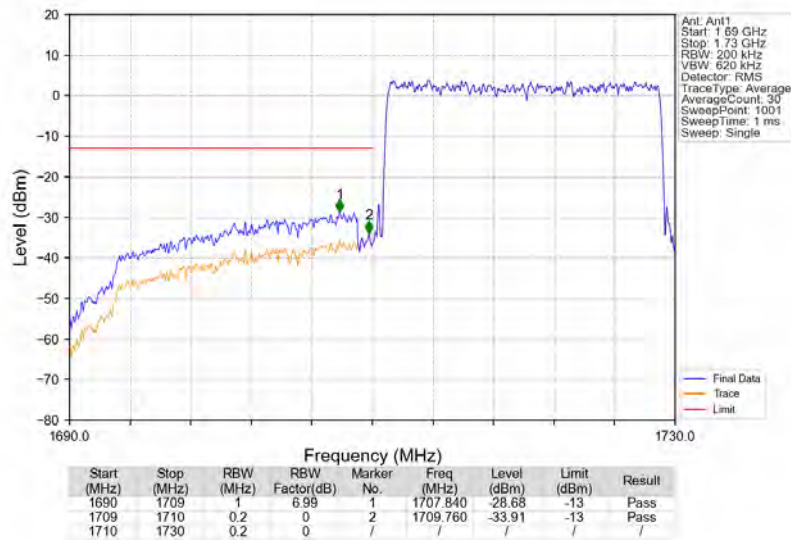
Band4_20MHz_QPSK_LCH_1720MHz_RB_100_0_NTNV
