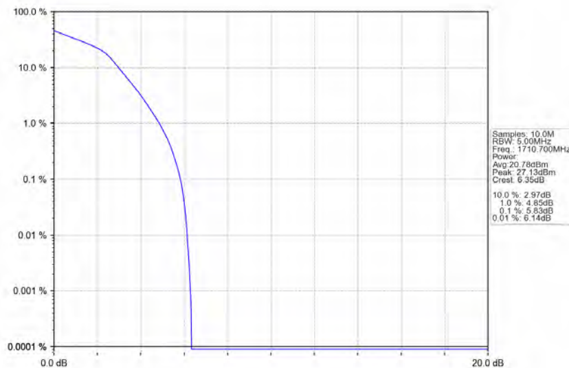
Band4 1.4MHz 16QAM LCH 1710.7MHz RB 6 0 NTNV
