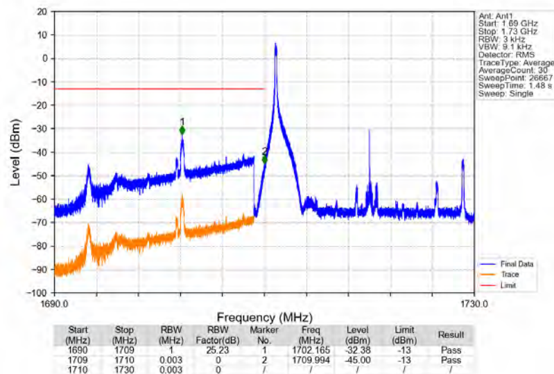
Band4_20MHz_16QAM_LCH_1720MHz_RB_1_0_NTNV
