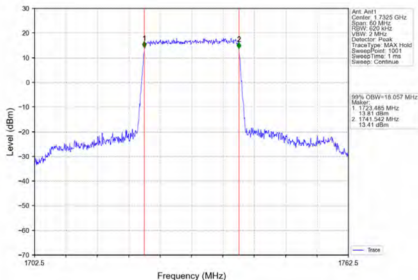
Band4_20MHz_QPSK_MCH_1732.5MHz_RB_100_0_NTNV
