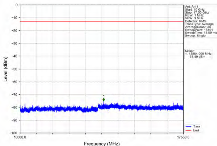
Band4_10MHz_QPSK_HCH_1750MHz_RB_1_0_NTNV
