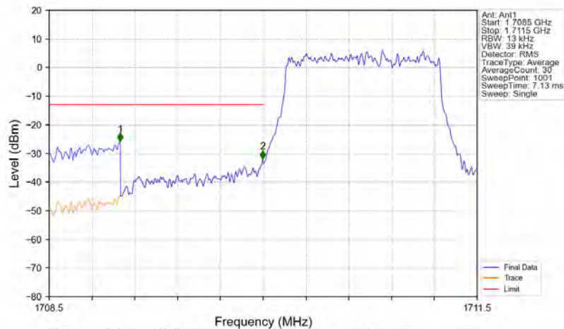
Band4 1.4MHz QPSK LCH 1710.7MHz RB 6 0 NTV
