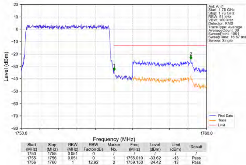
Band4 5MHz QPSK HCH 1752.5MHz_RB_25_0_NTNV
