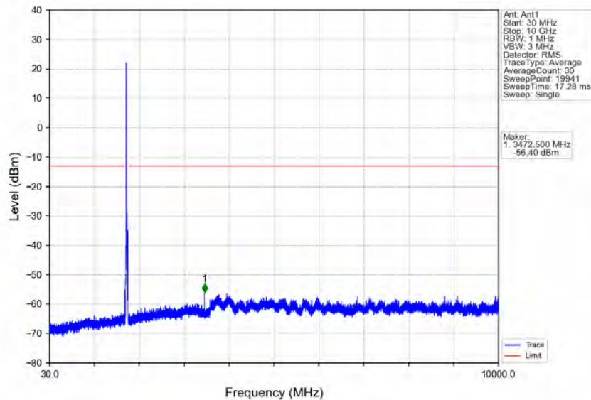
Band4_20MHz_QPSK_HCH_1745MHz_RB_1_0_NTNV
