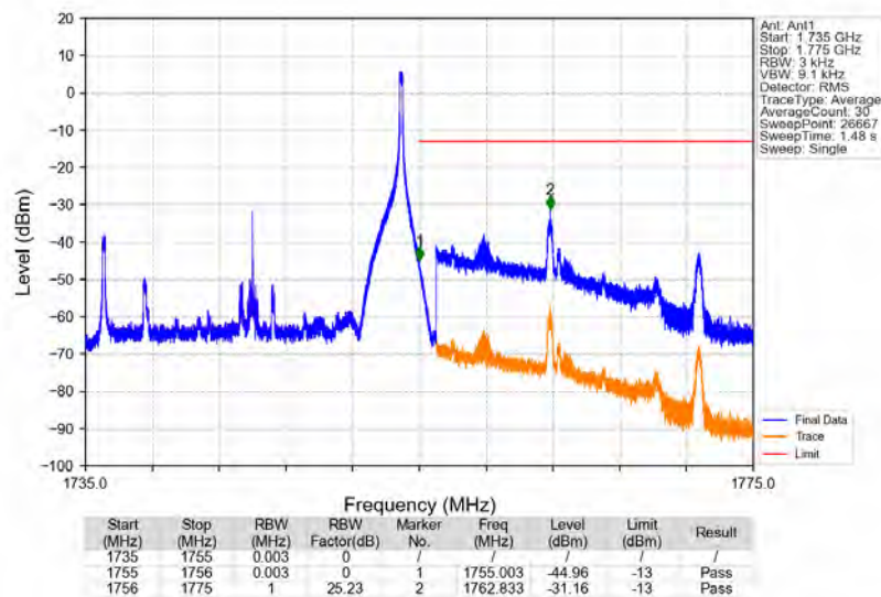
Band4_20MHz_QPSK_HCH_1745MHz_RB_1_99_NTNV
