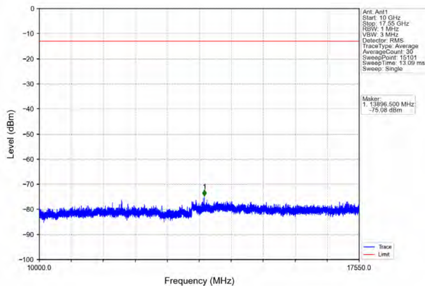
Band4_20MHz_QPSK_HCH_1745MHz_RB_1_0_NTNV
