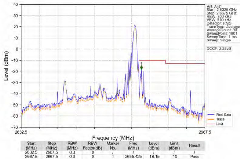
Band41_15MHz_QPSK_HCH_2647.5MHz_RB_1_74_NTNV
