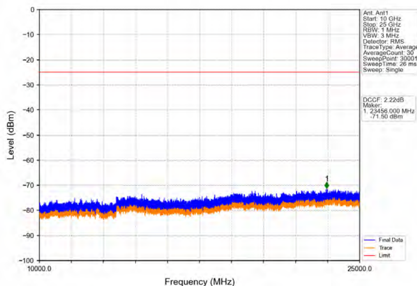
Band41_10MHz_QPSK_HCH_2650MHz_RB_1_0_NTNV
