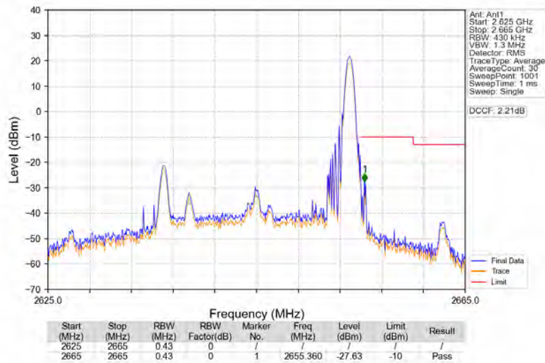
Band41_20MHz_QPSK_HCH_2645MHz_RB_1_99_NTNV
