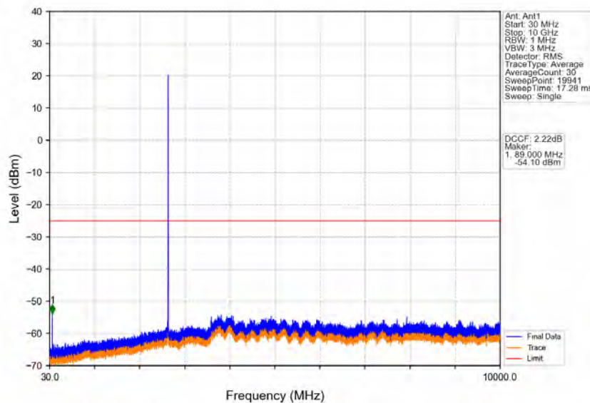
Band41_5MHz_QPSK_HCH_2652.5MHz_RB_1_0_NTNV
