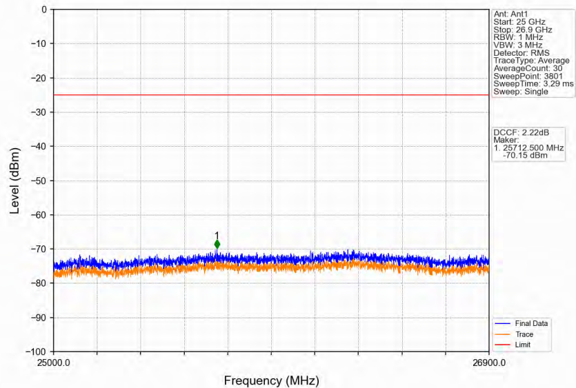
Band41_15MHz_QPSK_HCH_2647.5MHz_RB_1_74_NTNV
