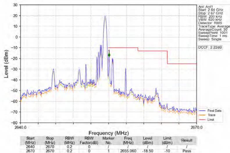
Band41_10MHz_16QAM_HCH_2650MHz_RB_1_49_NTNV
