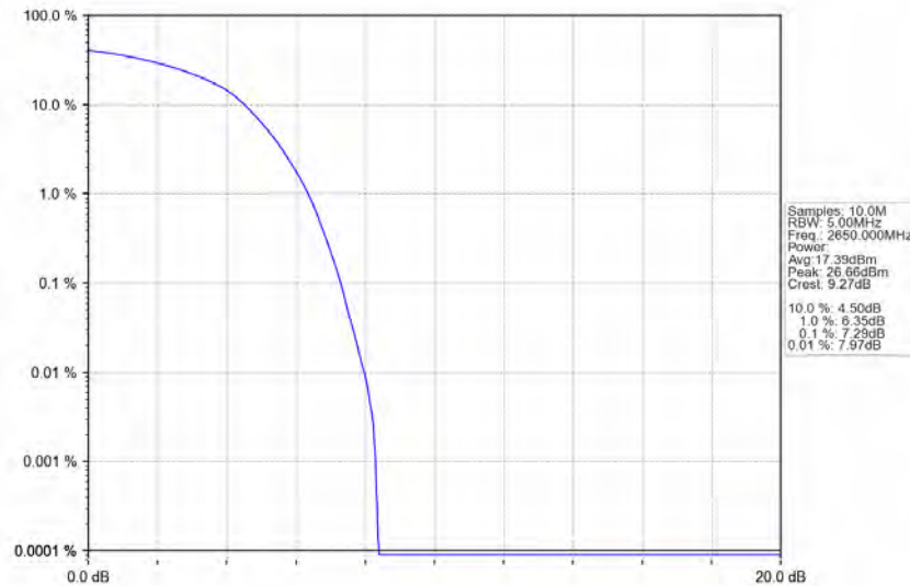
Band41_10MHz_QPSK_HCH_2650MHz_RB_50_0_NTNV
