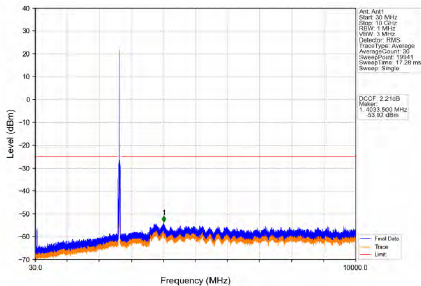
Band41_20MHz_QPSK_HCH_2645MHz_RB_1_0_NTNV
