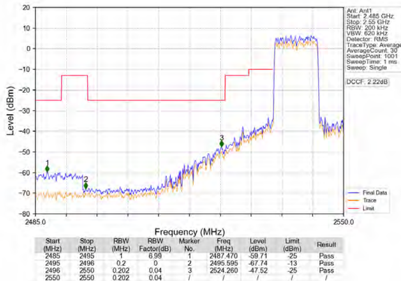
Band41_10MHz_16QAM_LCH_2540MHz_RB_50_0_NTNV
