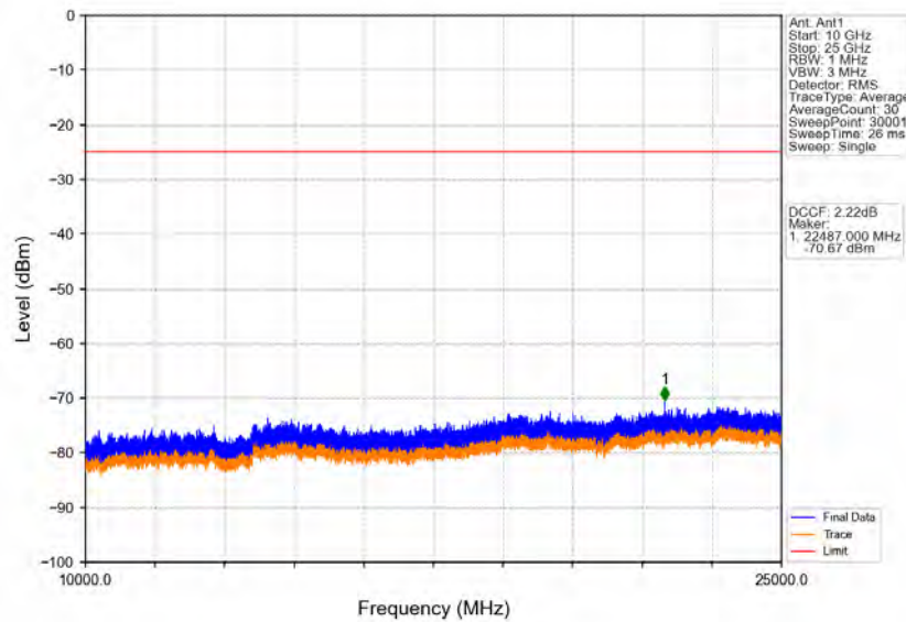
Band41_10MHz_QPSK_MCH_2595MHz_RB_1_0_NTNV
