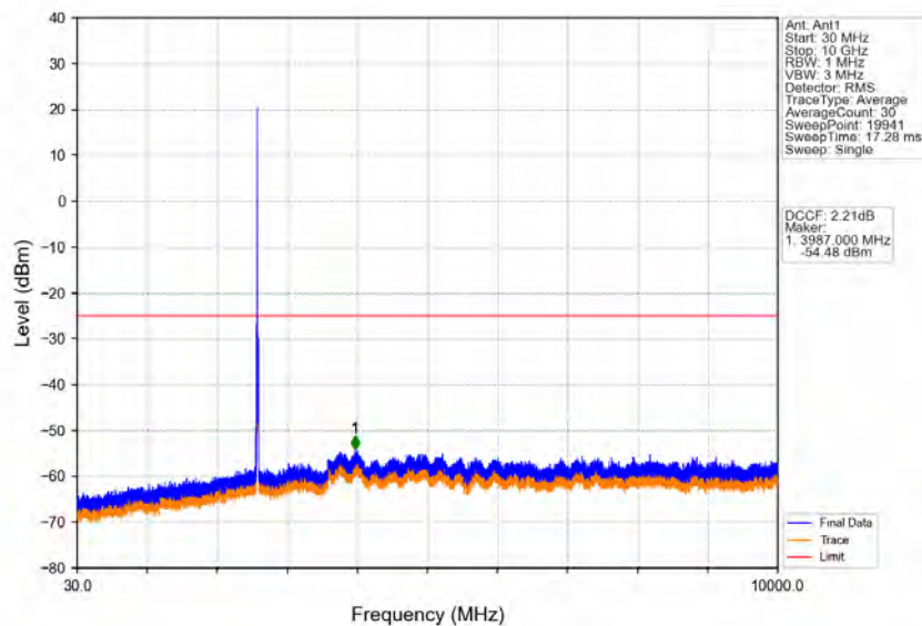
Band41_10MHz_16QAM_MCH_2595MHz_RB_1_0_NTNV
