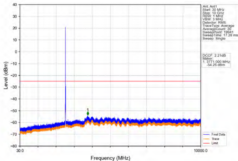
Band41_10MHz_16QAM_LCH_2540MHz_RB_1_0_NTNV
