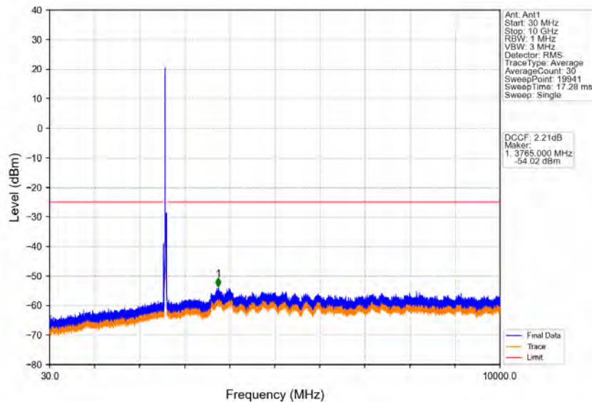
Band41_20MHz_16QAM_MCH_2595MHz_RB_1_0_NTNV
