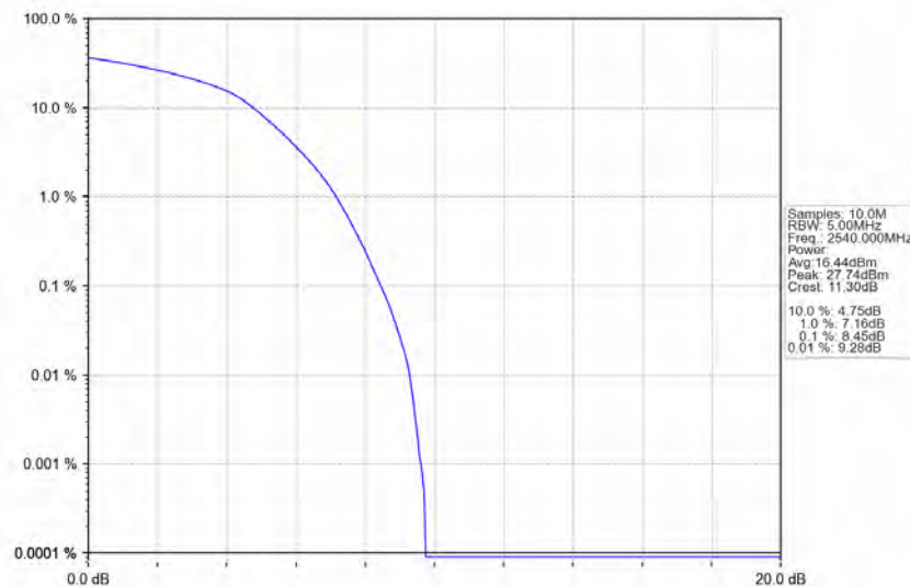
Band41_10MHz_16QAM_LCH_2540MHz_RB_50_0_NTNV
