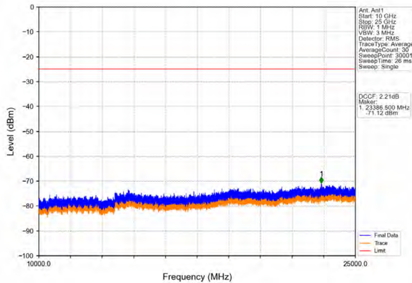
Band41_20MHz_QPSK_LCH_2545MHz_RB_1_0_NTNV
