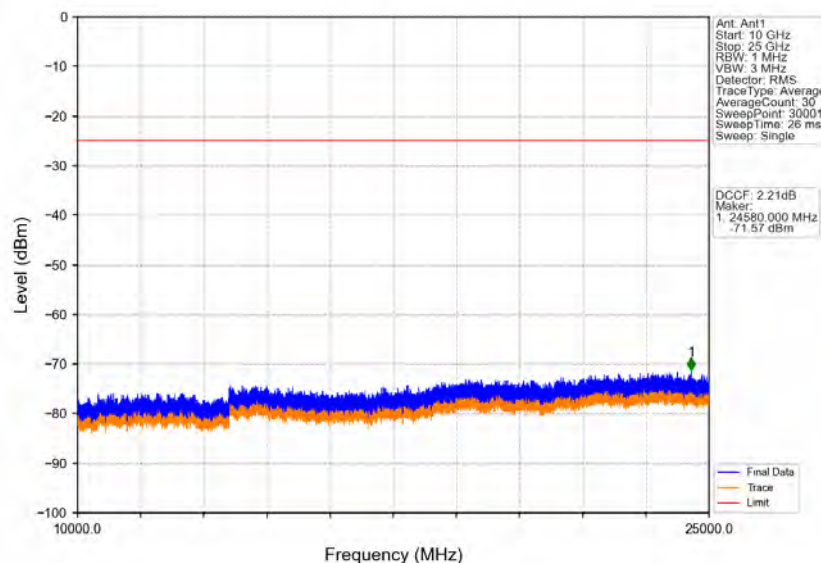
Band41_20MHz_16QAM_MCH_2595MHz_RB_1_0_NTNV
