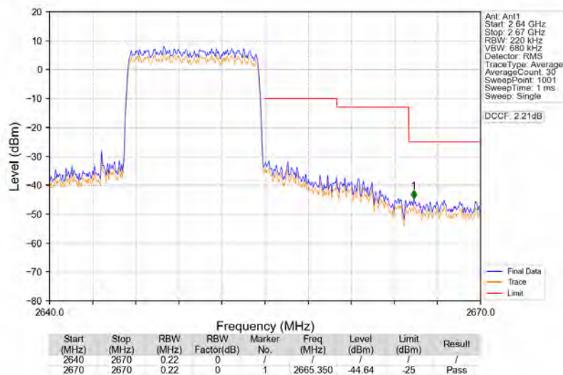
Band41_10MHz_QPSK_HCH_2650MHz_RB_50_0_NTNV
