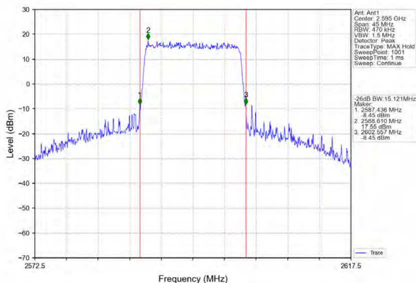
Band41_15MHz_QPSK_MCH_2595MHz_RB_75_0_NTNV
