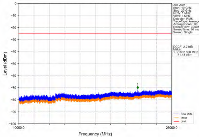
Band41_5MHz_QPSK_MCH_2595MHz_RB_1_0_NTNV
