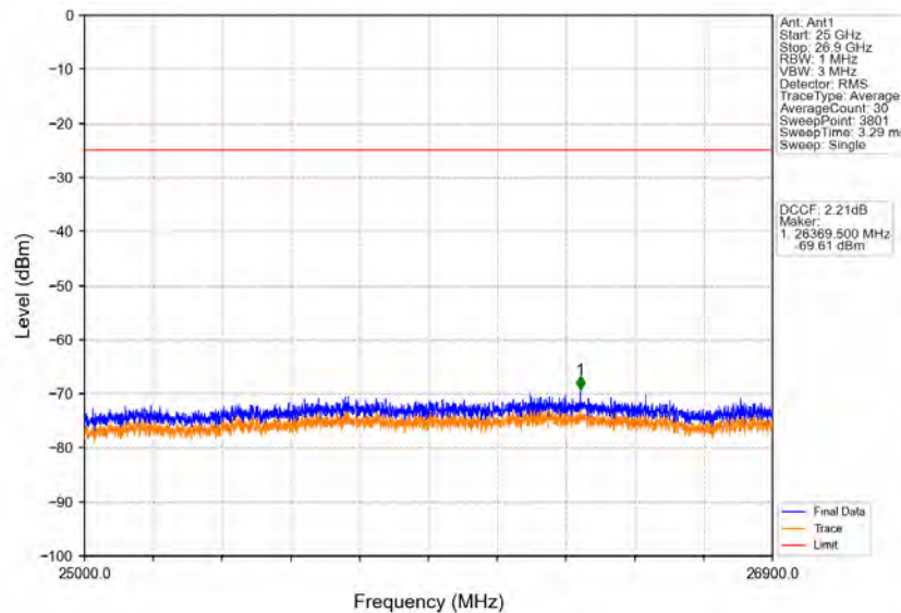
Band41_10MHz_16QAM_LCH_2540MHz_RB_50_0_NTNV
