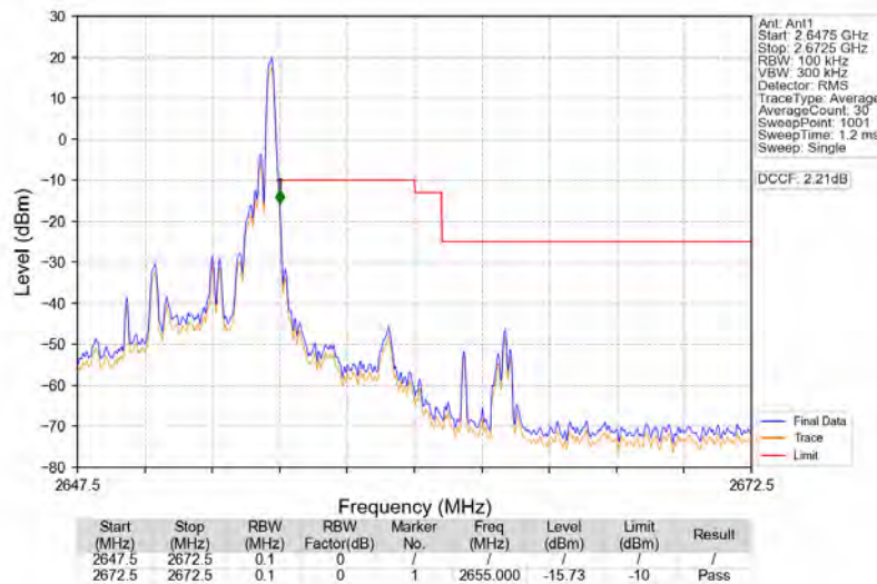
Band41_5MHz_QPSK_HCH_2652.5MHz_RB_1_24_NTNV
