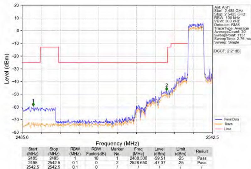
Band41_5MHz_QPSK_LCH_2537.5MHz_RB_25_0_NTNV
