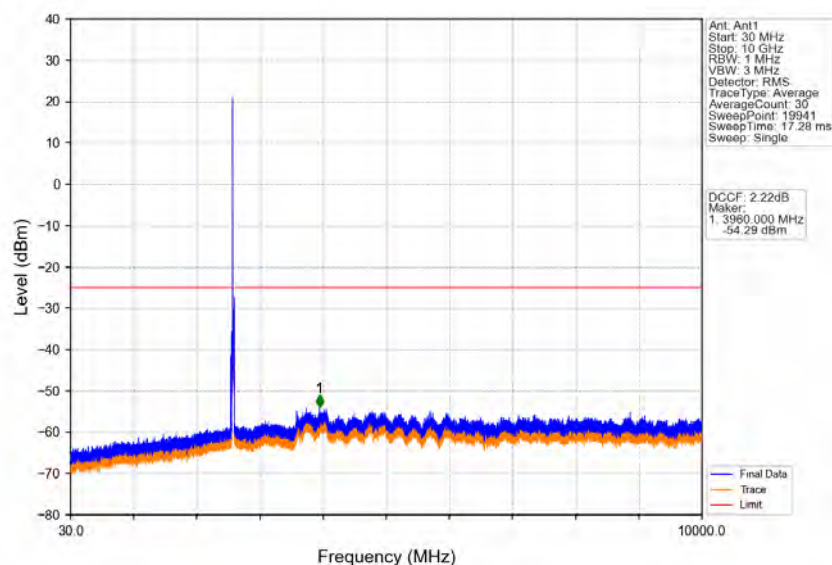
Band41_15MHz_QPSK_MCH_2595MHz_RB_1_0_NTNV
