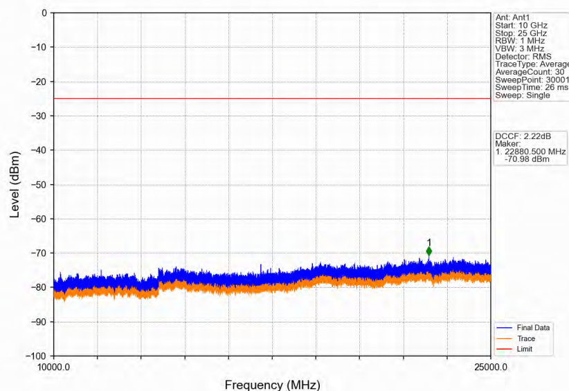
Band41_15MHz_QPSK_HCH_2647.5MHz_RB_1_0_NTNV
