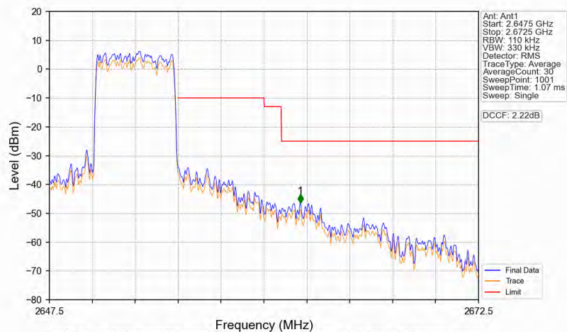
Band41_5MHz_QPSK_HCH_2652.5MHz_RB_25_0_NTNV
