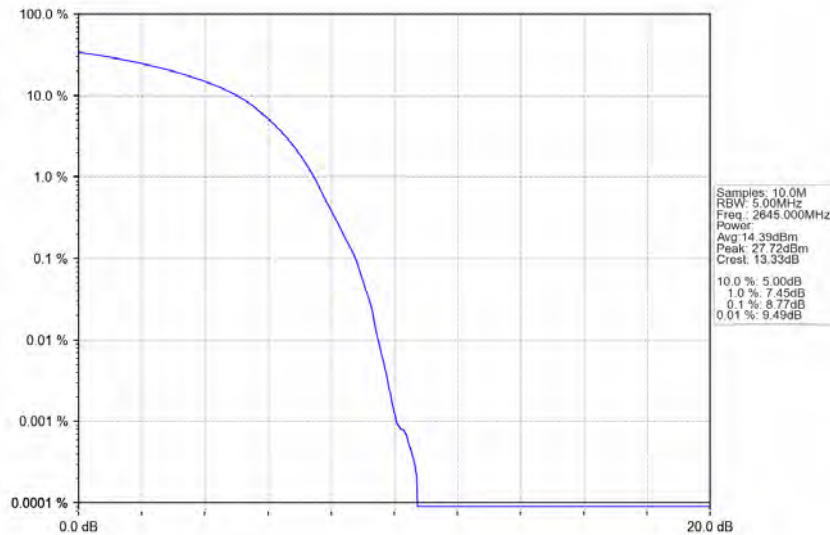
Band41_20MHz_QPSK_HCH_2645MHz_RB_100_0_NTNV
