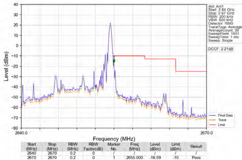
Band41_10MHz_QPSK_HCH_2650MHz_RB_1_49_NTNV
