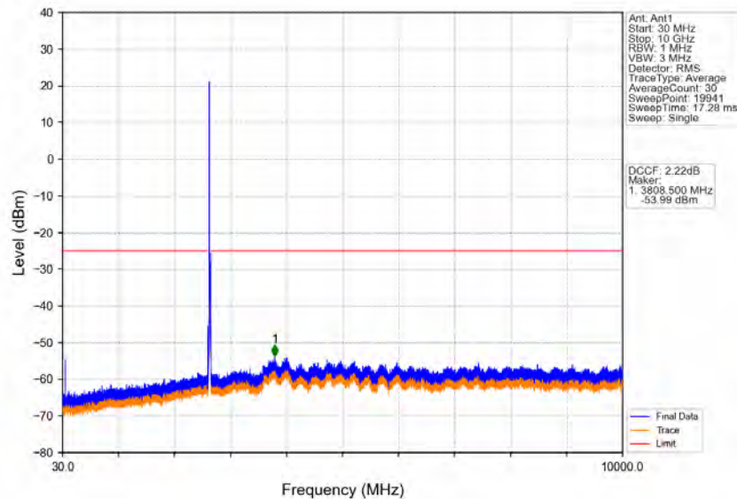
Band41_15MHz_QPSK_HCH_2647.5MHz_RB_1_0_NTNV
