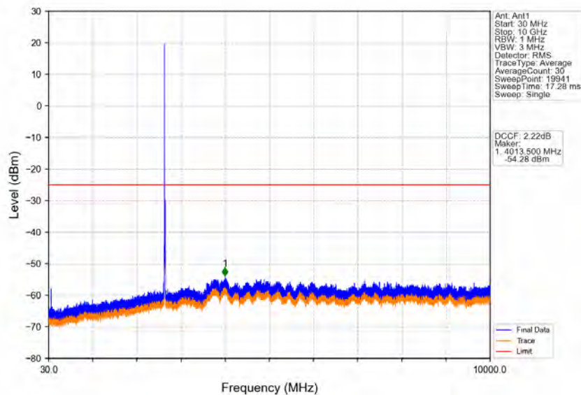
Band41_10MHz_QPSK_HCH_2650MHz_RB_1_0_NTNV
