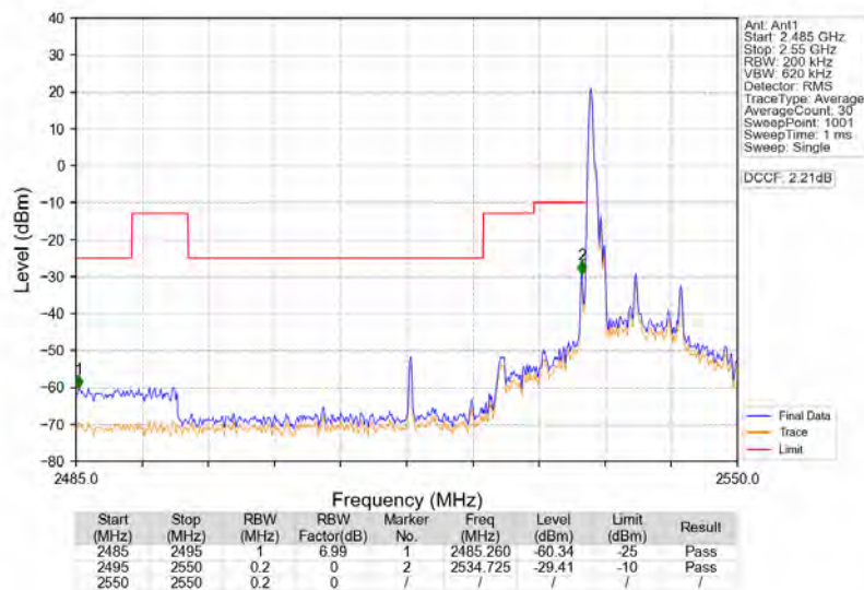
Band41_10MHz_16QAM_LCH_2540MHz_RB_1_0_NTNV
