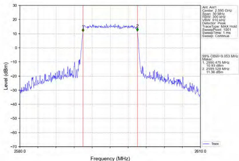
Band41_10MHz_QPSK_MCH_2595MHz_RB_50_0_NTNV
