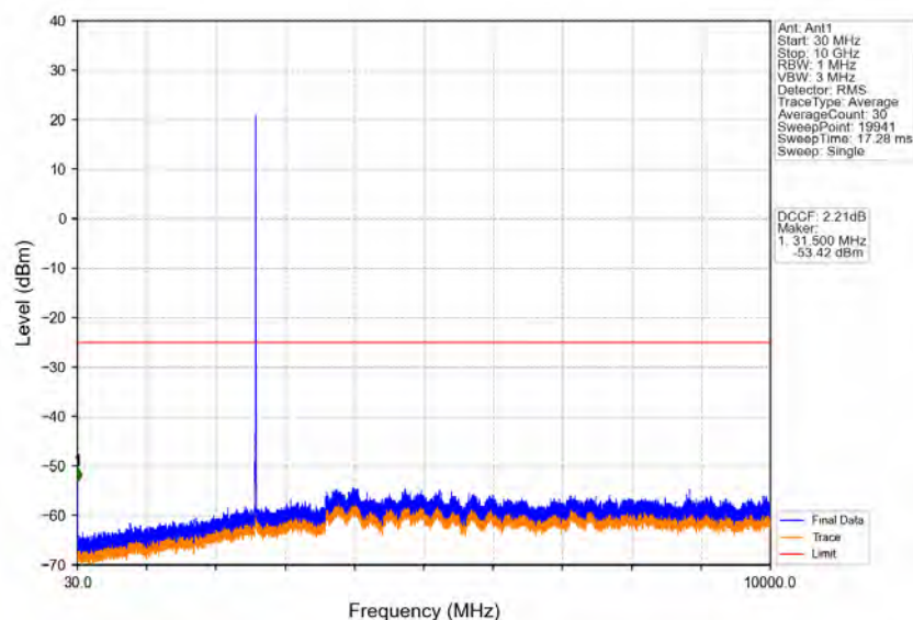
Band41_5MHz_QPSK_MCH_2595MHz_RB_1_0_NTNV
