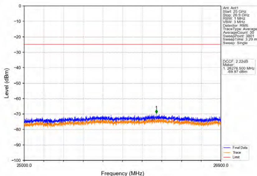
Band41_10MHz_QPSK_LCH_2540MHz_RB_1_0_NTNV
