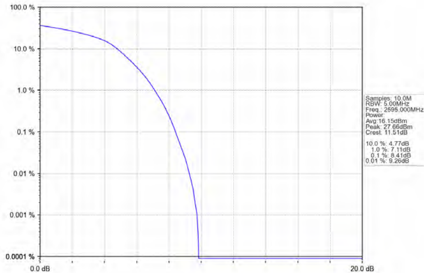
Band41_10MHz_16QAM_MCH_2595MHz_RB_50_0_NTNV
