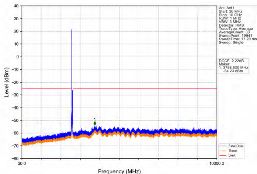
Band41_20MHz_QPSK_MCH_2595MHz_RB_1_0_NTNV
