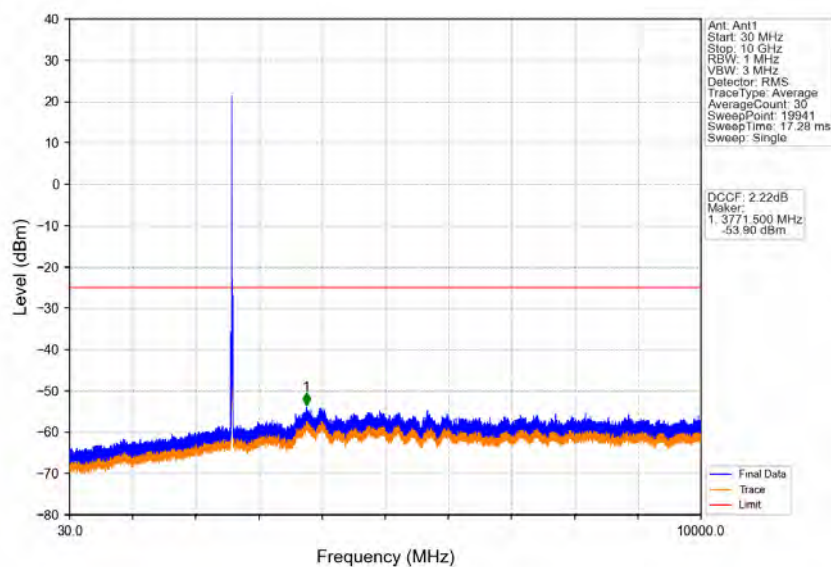
Band41_10MHz_QPSK_MCH_2595MHz_RB_1_0_NTNV
