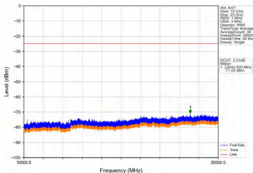
Band41_10MHz_16QAM_MCH_2595MHz_RB_1_0_NTNV
