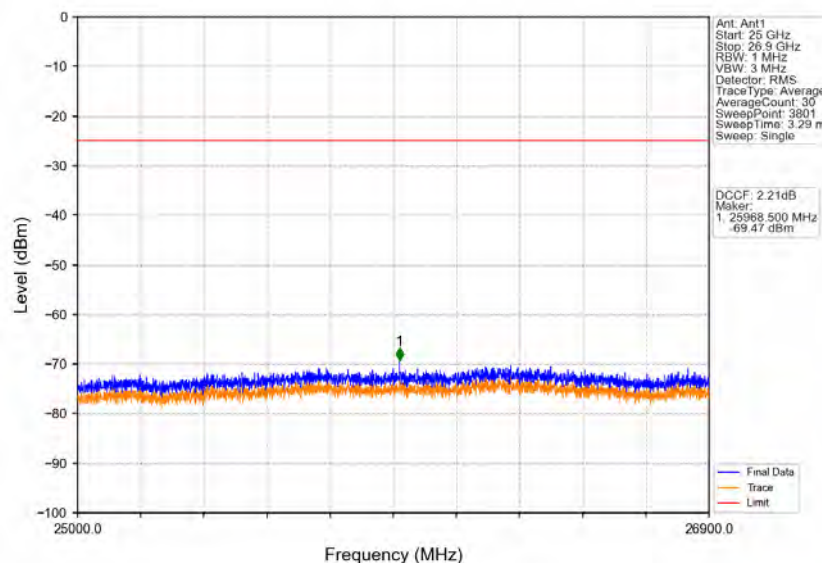
Band41_5MHz_QPSK_LCH_2537.5MHz_RB_1_0_NTNV
