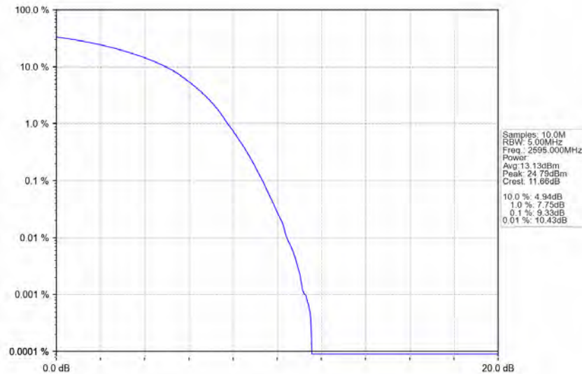
Band41_20MHz_16QAM_MCH_2595MHz_RB_100_0_NTNV
