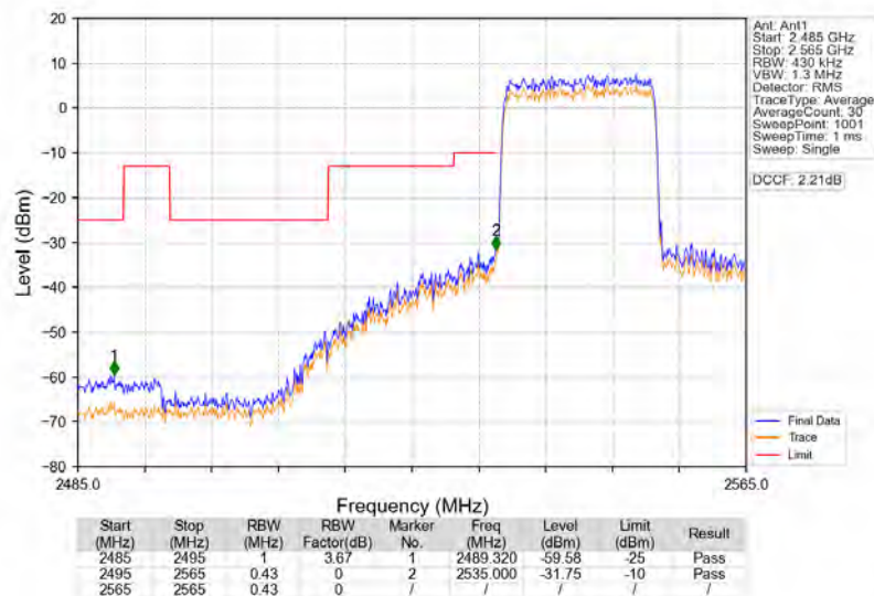
Band41_20MHz_QPSK_LCH_2545MHz_RB_100_0_NTNV
