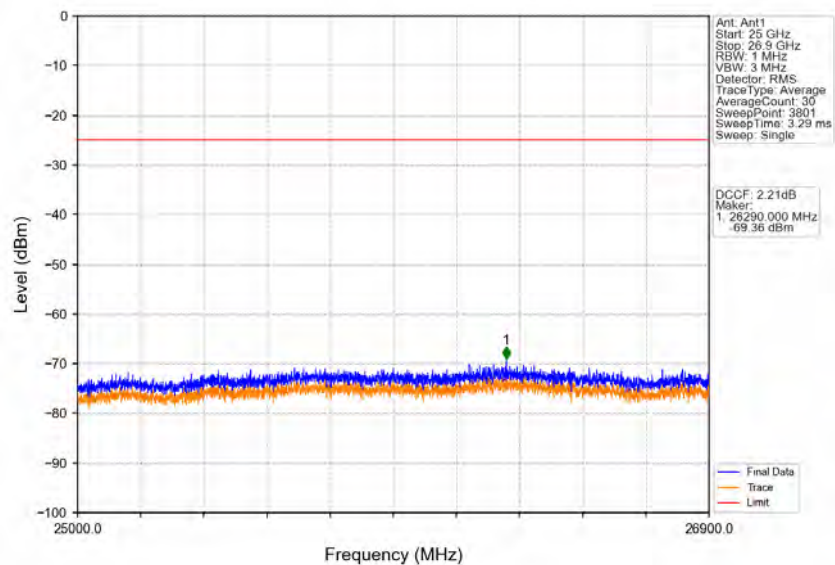
Band41_20MHz_QPSK_HCH_2645MHz_RB_1_99_NTNV
