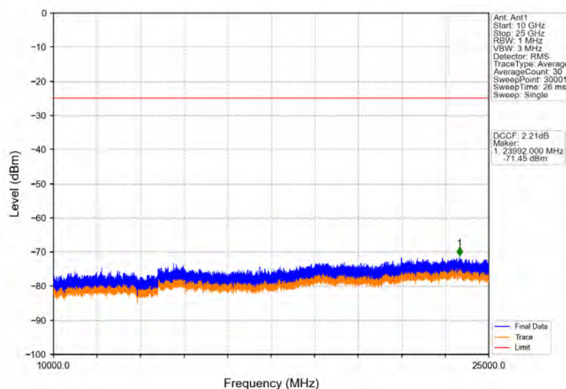
Band41_20MHz_QPSK_HCH_2645MHz_RB_1_0_NTNV
