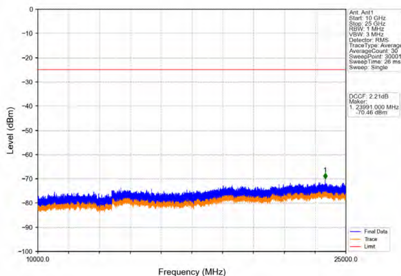
Band41_10MHz_16QAM_LCH_2540MHz_RB_1_0_NTNV
