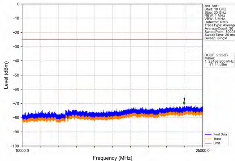
Band41_20MHz_QPSK_MCH_2595MHz_RB_1_0_NTNV
