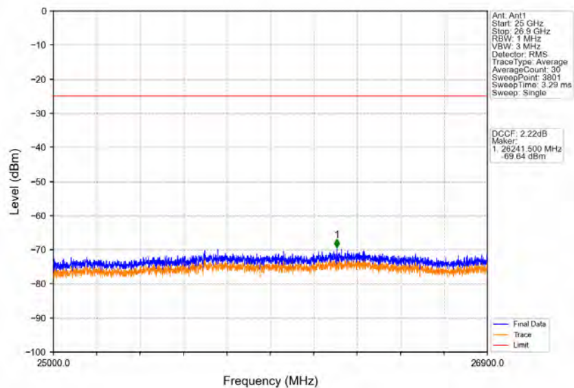
Band41_10MHz_QPSK_HCH_2650MHz_RB_1_49_NTNV
