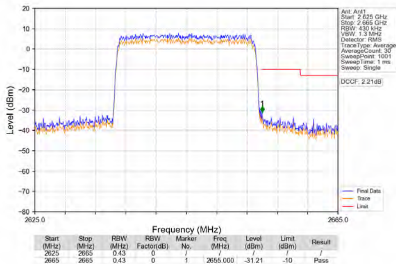
Band41_20MHz_QPSK_HCH_2645MHz_RB_100_0_NTNV
