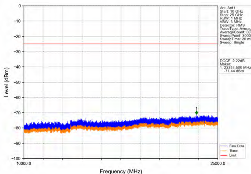
Band41_5MHz_QPSK_HCH_2652.5MHz_RB_1_0_NTNV
