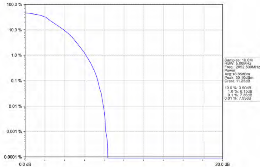
Band41_5MHz_QPSK_HCH_2652.5MHz_RB_25_0_NTNV
