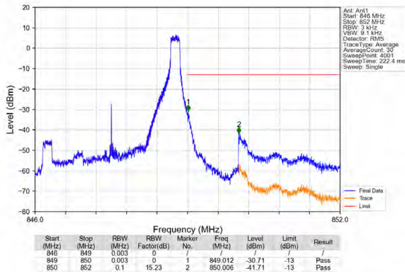
Band5_3MHz_QPSK_HCH_847.5MHz_RB_1_14_NTNV
