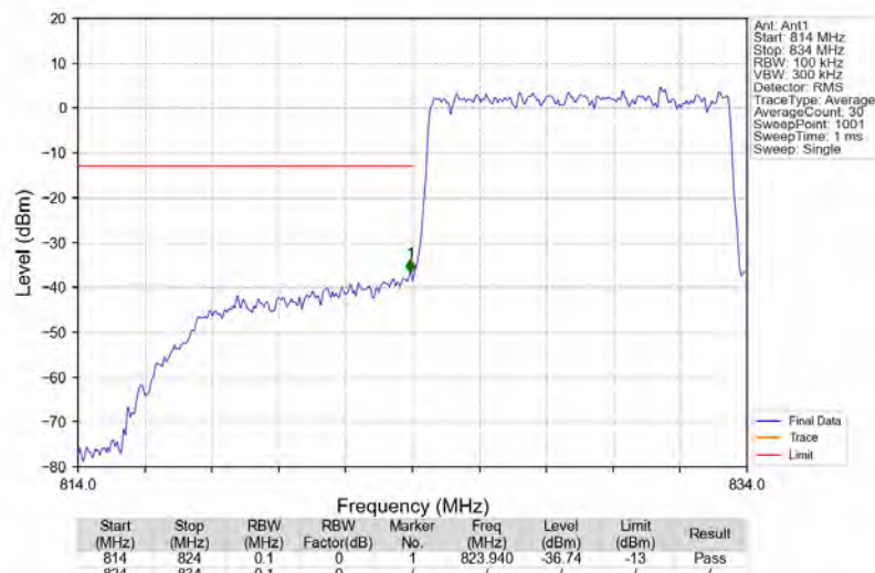
Band5_10MHz_QPSK_LCH_829MHz_RB_50_0_NTNV
