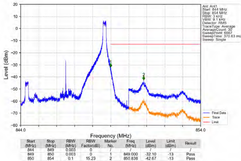
Band5_5MHz_QPSK_HCH_846.5MHz_RB_1_24_NTNV
