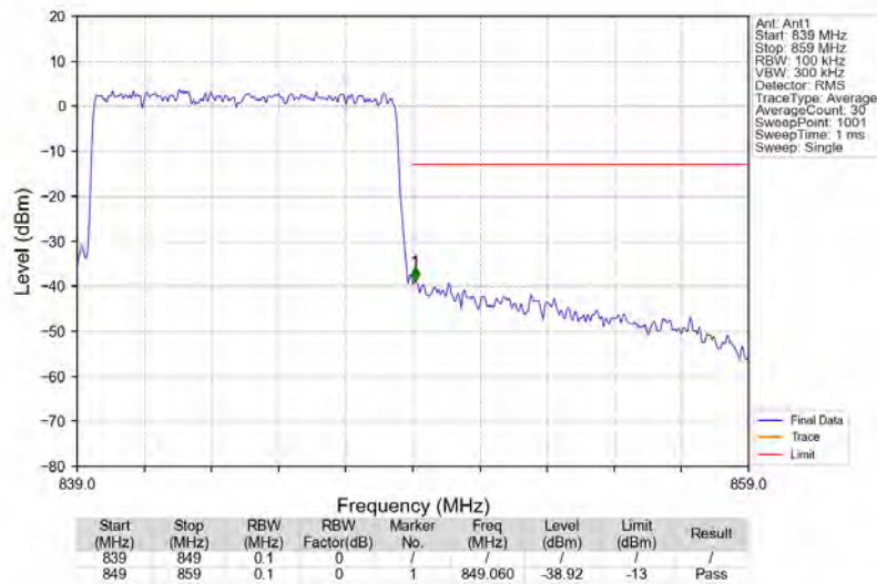
Band5_10MHz_QPSK_HCH_844MHz_RB_50_0_NTNV
