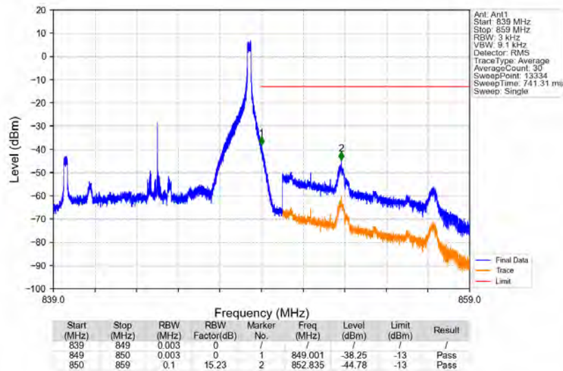
Band5_10MHz_QPSK_HCH_844MHz_RB_1_49_NTNV
