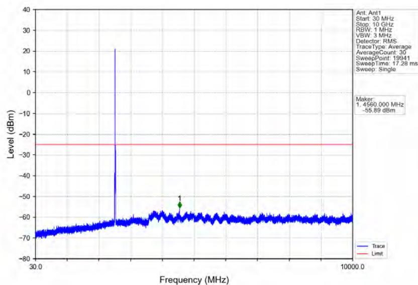
Band7_10MHz_QPSK_MCH_2535MHz_RB_1_0_NTNV
