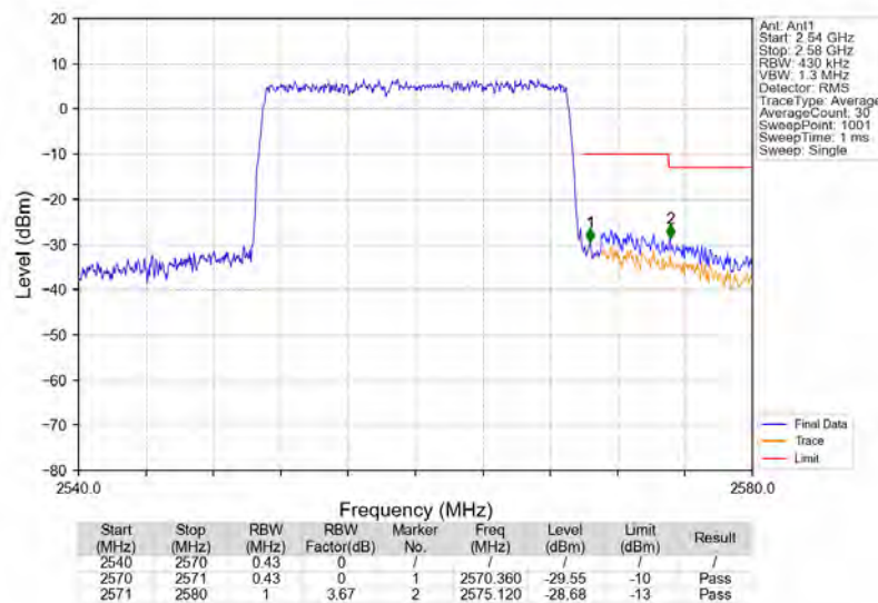
Band7_20MHz_QPSK_HCH_2560MHz_RB_100_0_NTNV
