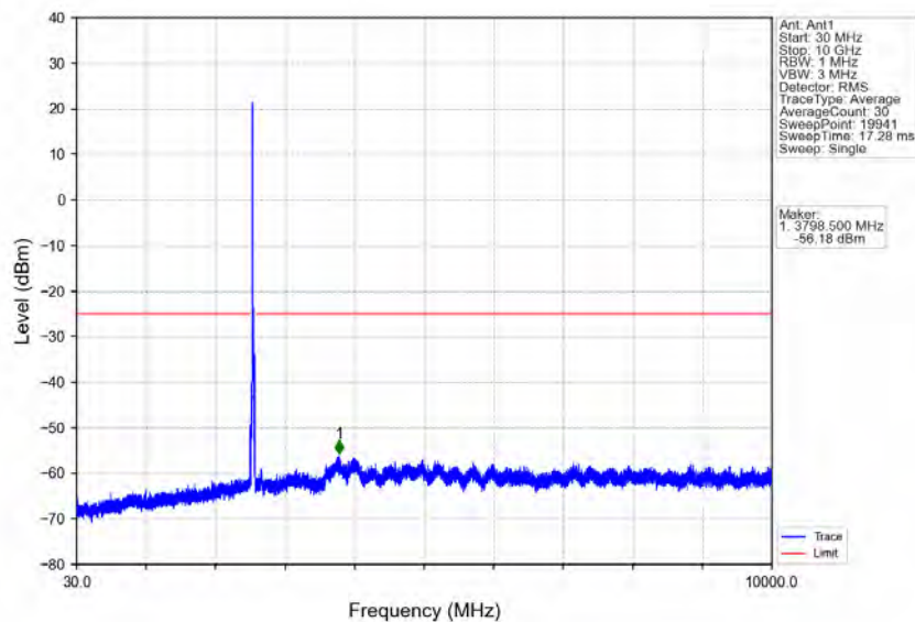
Band7_20MHz_QPSK_HCH_2560MHz_RB_1_0_NTNV
