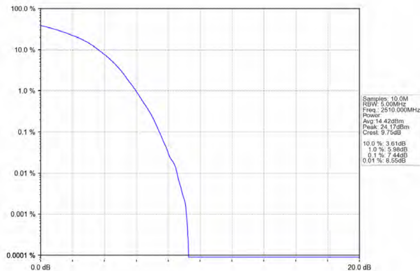
Band7_20MHz_16QAM_LCH_2510MHz_RB_100_0_NTNV
