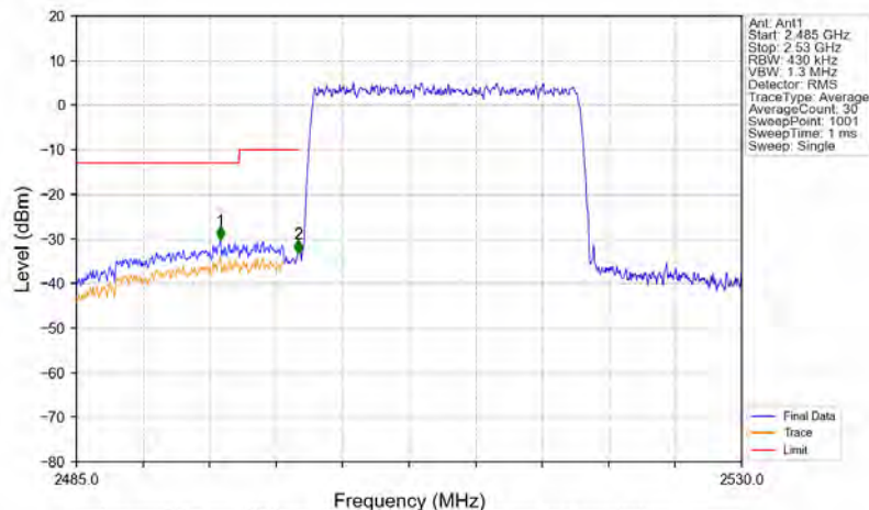
Band7_20MHz_16QAM_LCH_2510MHz_RB_100_0_NTNV
