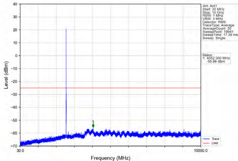
Band7_5MHz_QPSK_HCH_2567.5MHz_RB_1_0_NTNV
