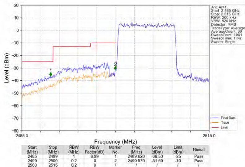
Band7_10MHz_QPSK_LCH_2505MHz_RB_50_0_NTNV
