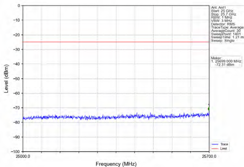
Band7_10MHz_QPSK_MCH_2535MHz_RB_1_0_NTNV
