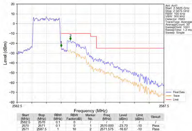
Band7_5MHz_QPSK_HCH_2567.5MHz_RB_25_0_NTNV
