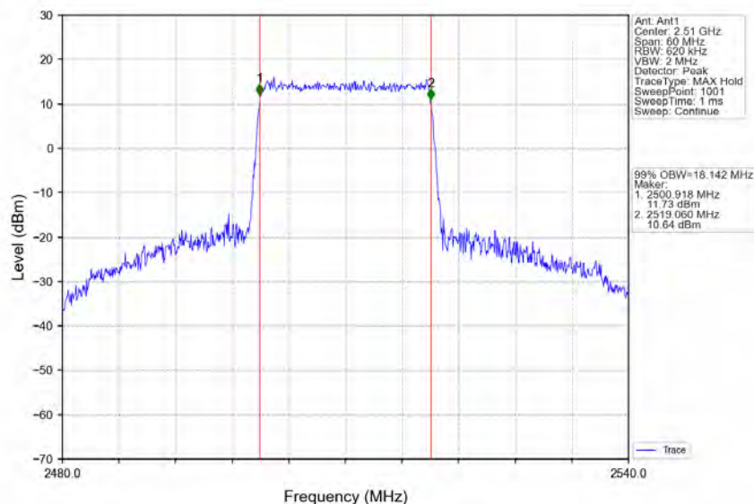
Band7_20MHz_16QAM_LCH_2510MHz_RB_100_0_NTNV
