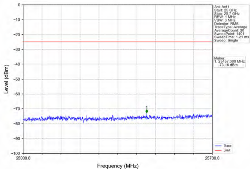
Band7_5MHz_QPSK_HCH_2567.5MHz_RB_1_24_NTNV
