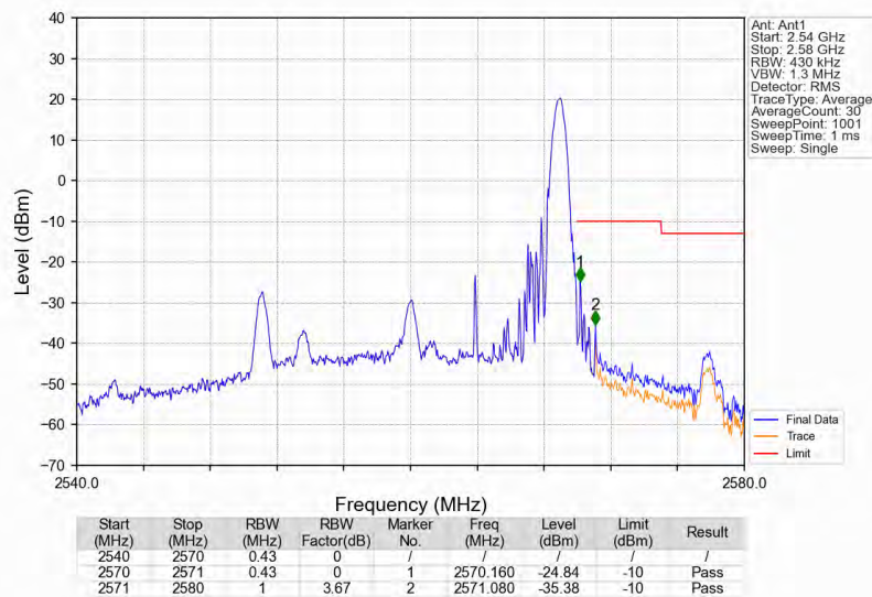
Band7_20MHz_16QAM_HCH_2560MHz_RB_1_99_NTNV
