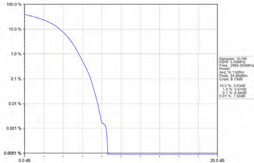
Band7_20MHz_QPSK_HCH_2560MHz_RB_100_0_NTNV
