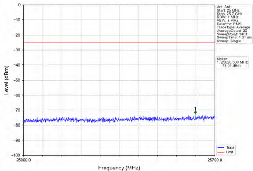
Band7 20MHz 16QAM HCH 2560MHz RB 1 0 NTV
