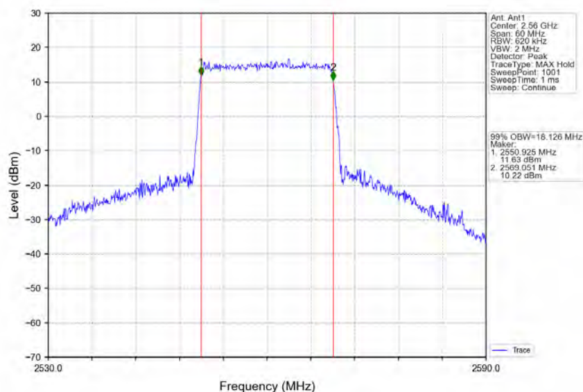
Band7_20MHz_16QAM_HCH_2560MHz_RB_100_0_NTNV
