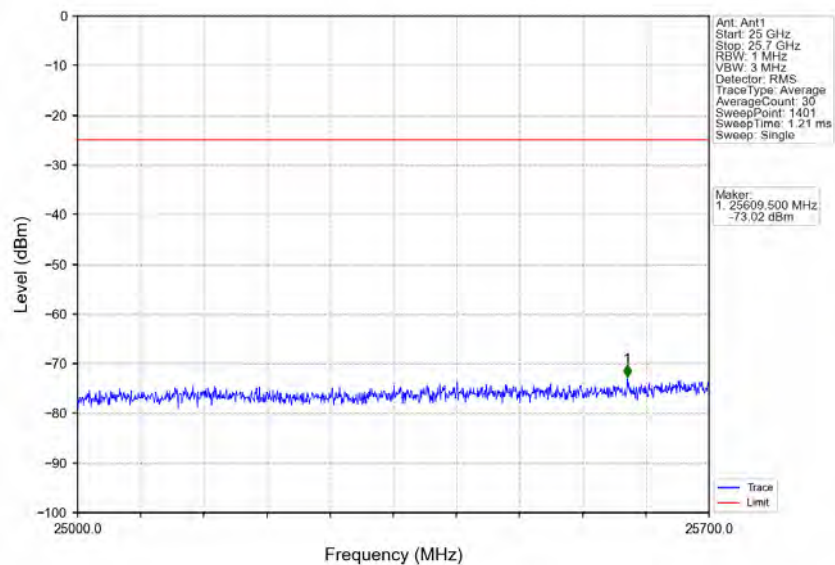
Band7_10MHz_QPSK_HCH_2565MHz_RB_1_49_NTNV
