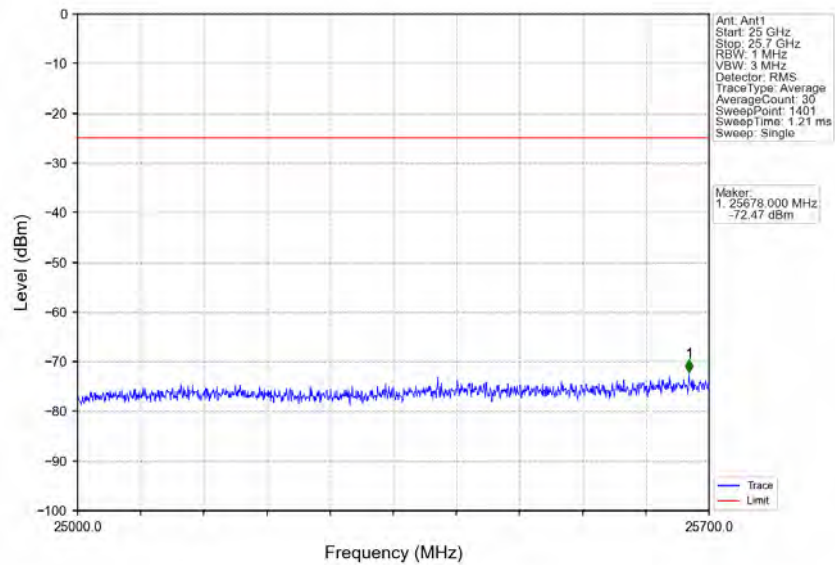
Band7_15MHz_QPSK_HCH_2562.5MHz_RB_1_74_NTNV
