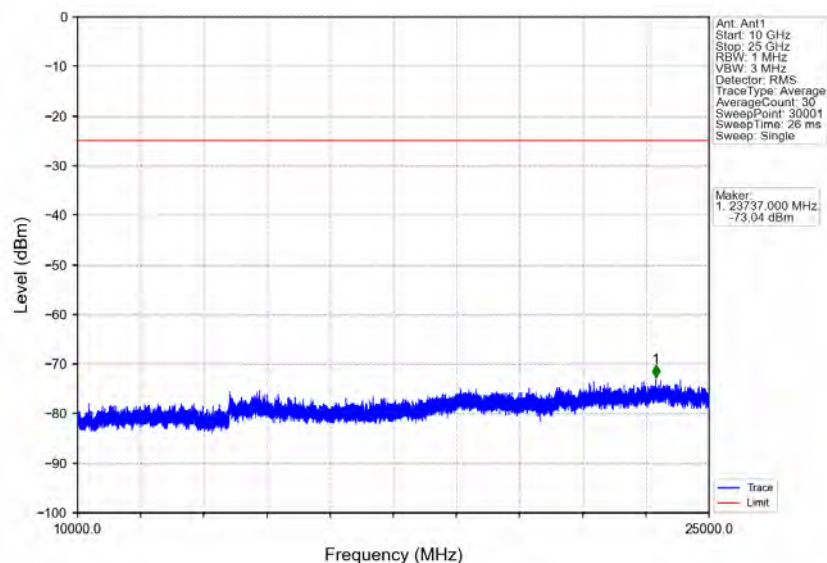
Band7_5MHz_QPSK_HCH_2567.5MHz_RB_1_0_NTNV
