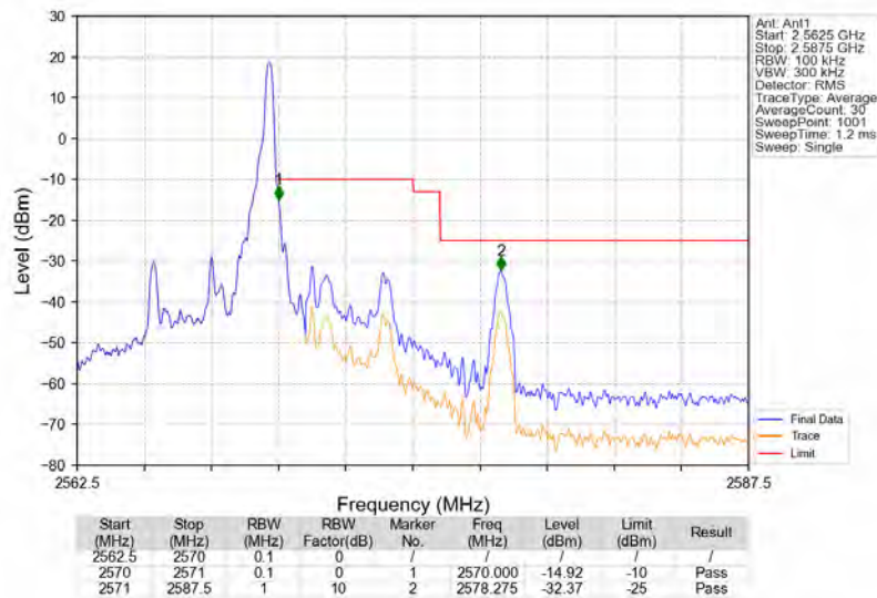
Band7_5MHz_QPSK_HCH_2567.5MHz_RB_1_24_NTNV
