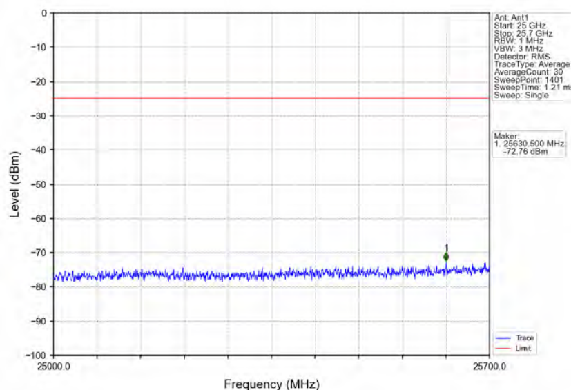
Band7_5MHz_QPSK_MCH_2535MHz_RB_1_0_NTNV
