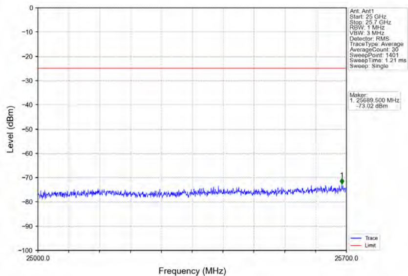
Band7_20MHz_QPSK_HCH_2560MHz_RB_1_99_NTNV
