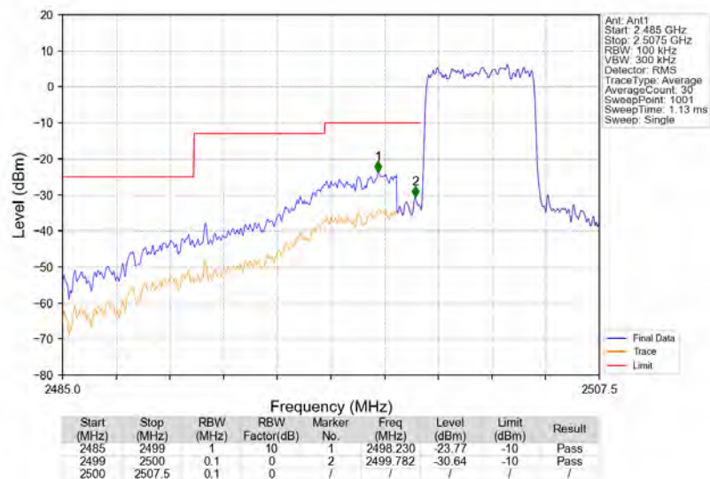
Band7 5MHz QPSK LCH 2502.5MHz RB 25_0 NTNV
