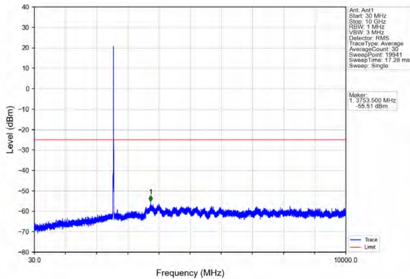
Band7_10MHz_QPSK_HCH_2565MHz_RB_1_0_NTNV
