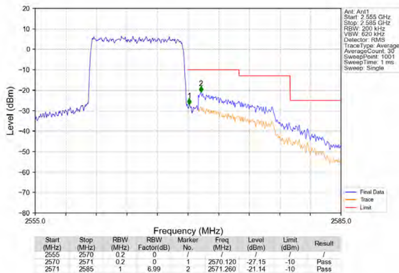
Band7_10MHz_QPSK_HCH_2565MHz_RB_50_0_NTNV
