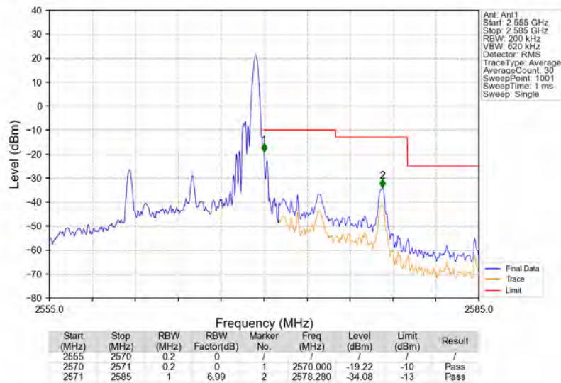
Band7_10MHz_QPSK_HCH_2565MHz_RB_1_49_NTNV
