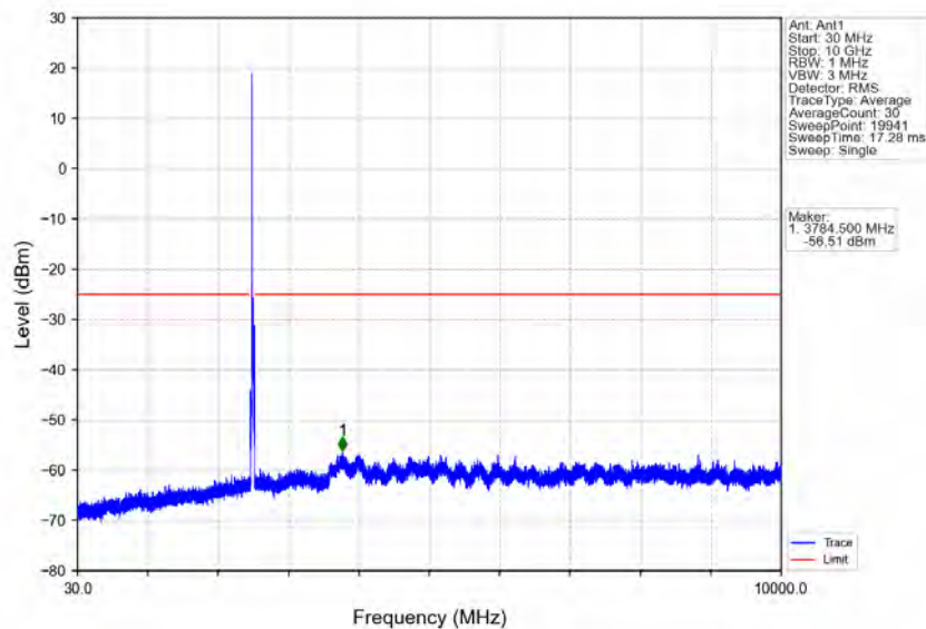
Band7_20MHz_16QAM_LCH_2510MHz_RB_1_0_NTNV
