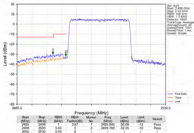
Band7_20MHz_QPSK_LCH_2510MHz_RB_100_0_NTNV
