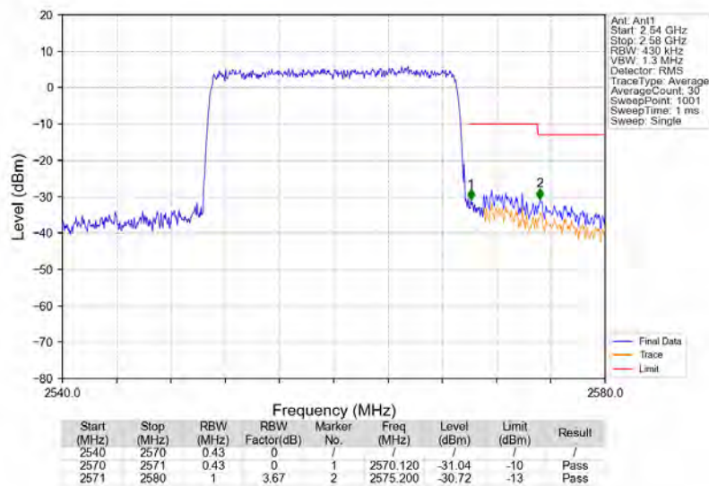
Band7_20MHz_16QAM_HCH_2560MHz_RB_100_0_NTNV
