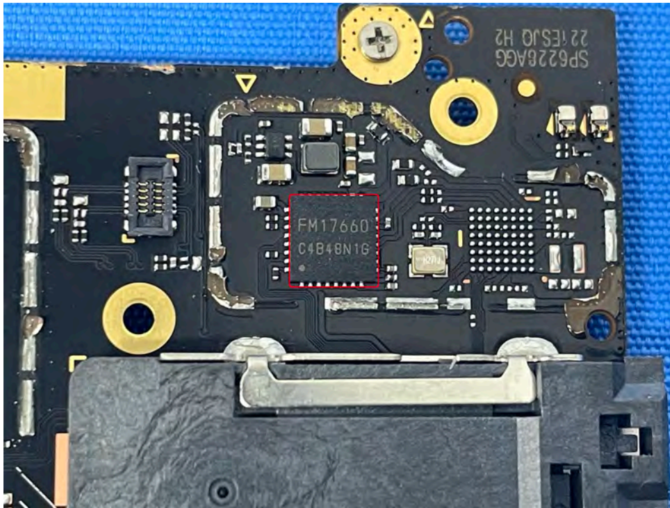
NFC module
