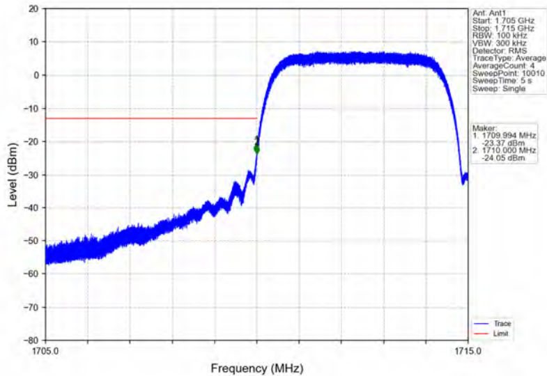
Band4_HSUPA_LCH_1712.4MHz_Subtest 1_NTNV
