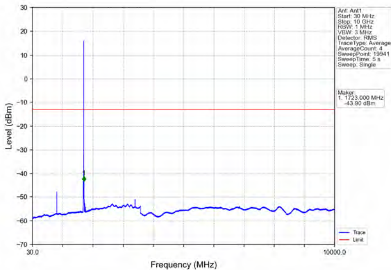
Band4_HSUPA_LCH_1712.4MHz_Subtest 1_NTNV
