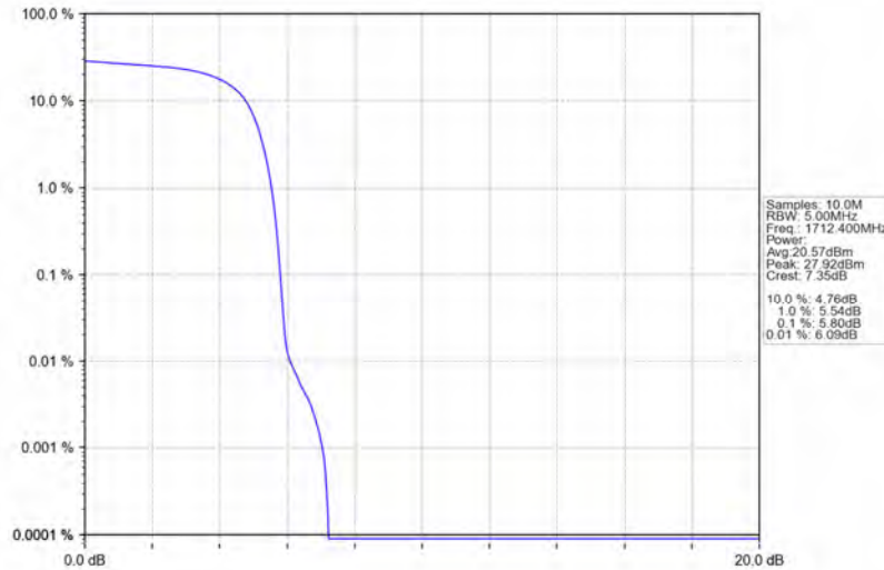
Band4_HSUPA_LCH_1712.4MHz_Subtest 1_NTNV
