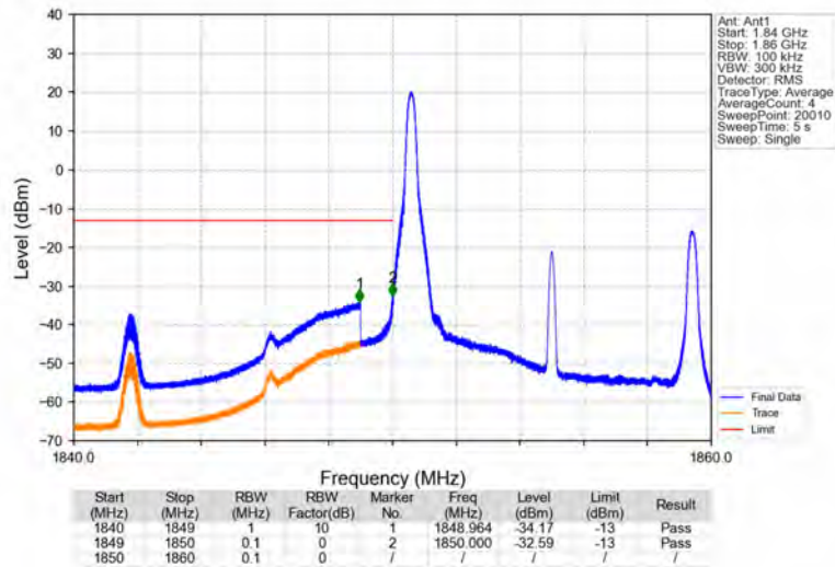
Band2_10MHz_16QAM_LCH_1855MHz_RB_1_0_NTNV
