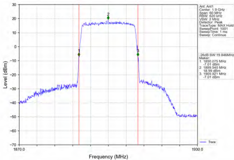
Band2_20MHz_QPSK_HCH_1900MHz_RB_100_0_NTNV
