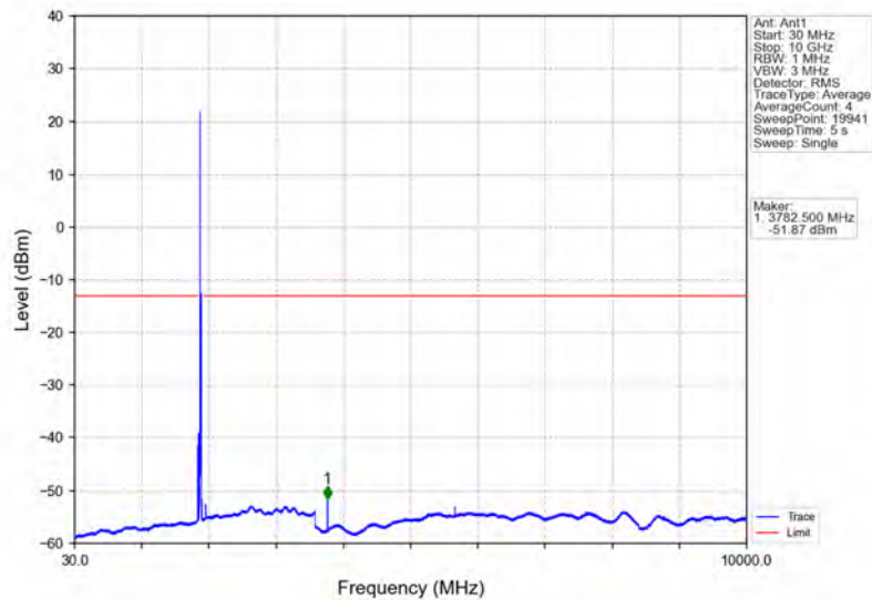
Band2_20MHz_16QAM_HCH_1900MHz_RB_1_0_NTNV
