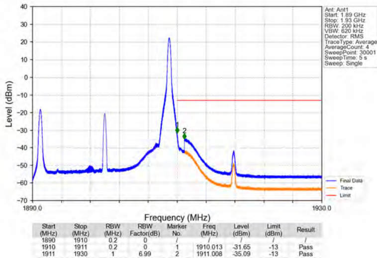
Band2_20MHz_QPSK_HCH_1900MHz_RB_1_99_NTNV
