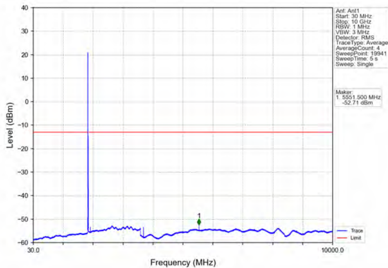
Band2_10MHz_64QAM_LCH_1855MHz_RB_1_0_NTNV
