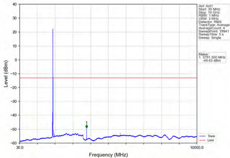
Band2_15MHz_QPSK_HCH_1902.5MHz_RB_1_0_NTNV
