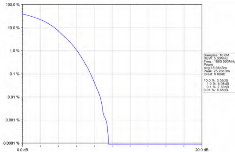
Band2_20MHz_16QAM_LCH_1860MHz_RB_100_0_NTNV
