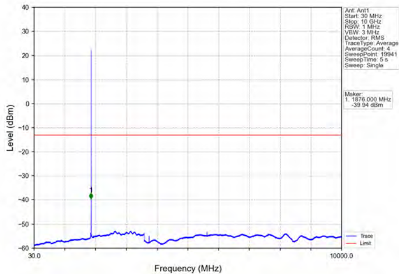
Band2_1.4MHz_QPSK_MCH_1880MHz_RB_1_0_NTNV
