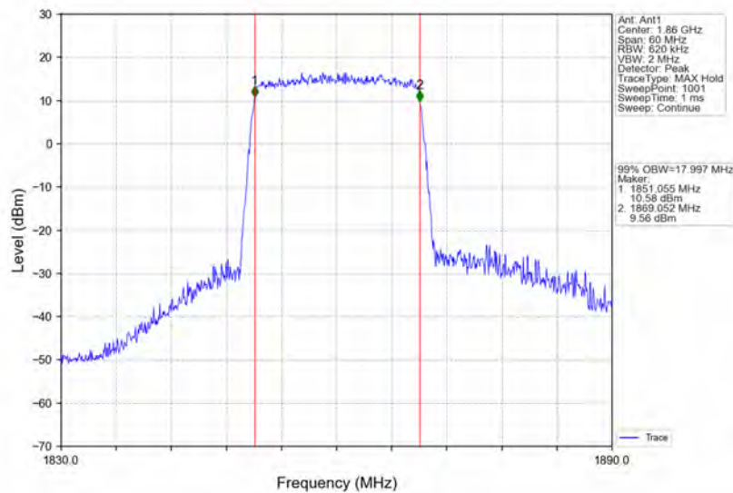
Band2_20MHz_64QAM_LCH_1860MHz_RB_100_0_NTNV
