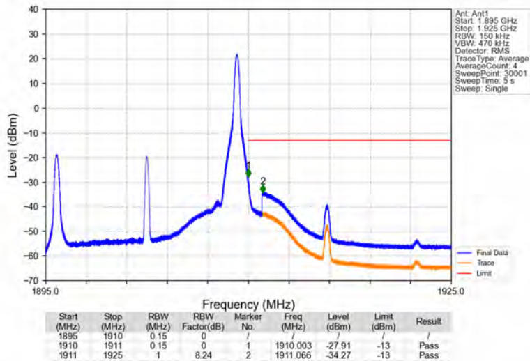
Band2_15MHz_QPSK_HCH_1902.5MHz_RB_1_74_NTNV
