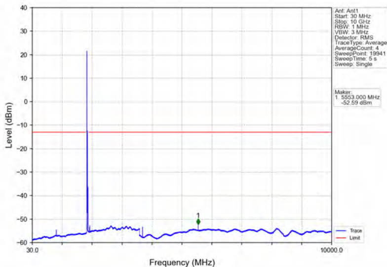
Band2_20MHz_16QAM_LCH_1860MHz_RB_1_0_NTNV
