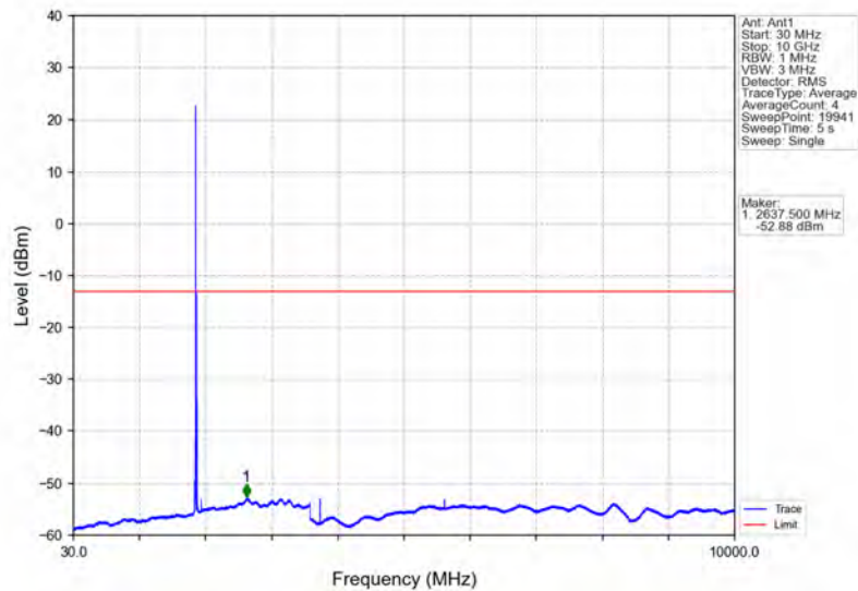
Band2_10MHz_16QAM_MCH_1880MHz_RB_1_0_NTNV
