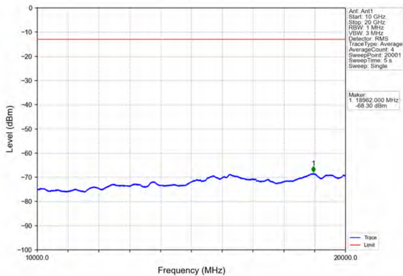
Band2_3MHz_QPSK_MCH_1880MHz_RB_1_0_NTNV
