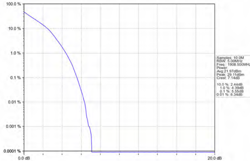
Band2_3MHz_QPSK_HCH_1908.5MHz_RB_15_0_NTNV
