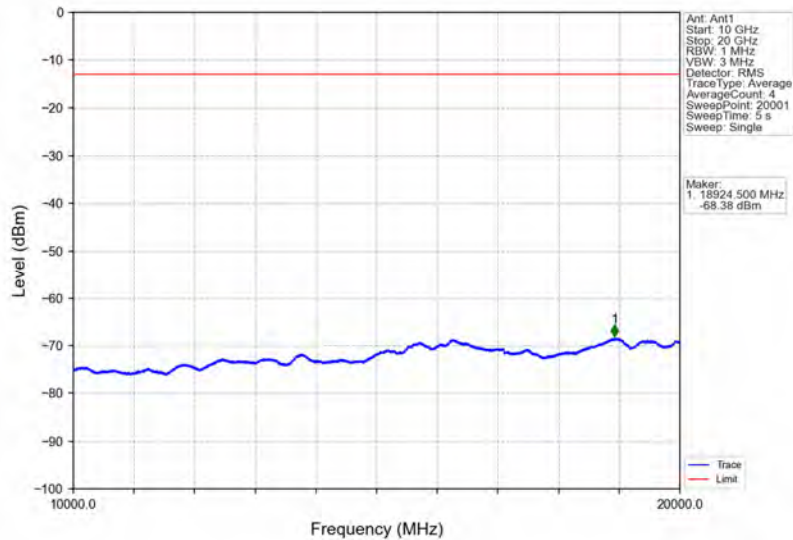
Band2_20MHz_QPSK_LCH_1860MHz_RB_100_0_NTNV
