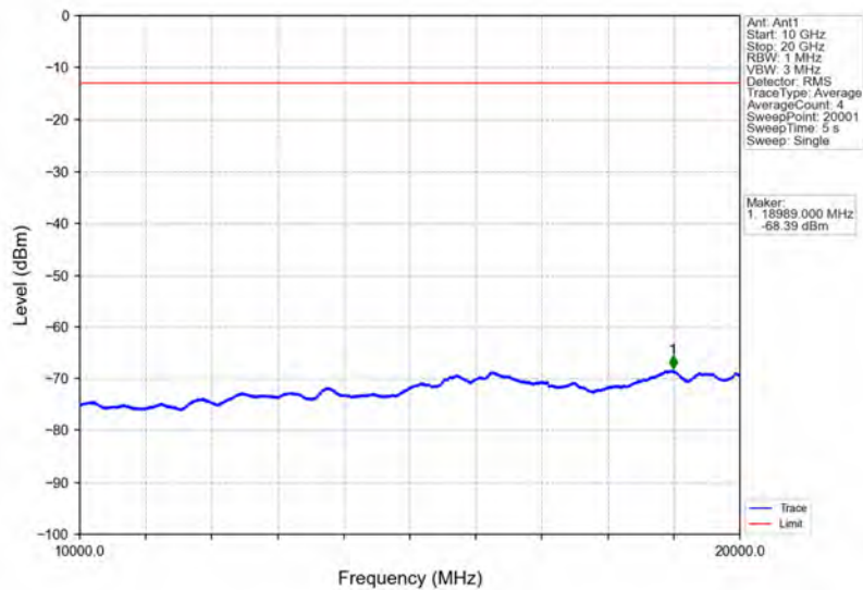
Band2_10MHz_QPSK_LCH_1855MHz_RB_50_0_NTNV
