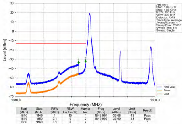
Band2_10MHz_64QAM_LCH_1855MHz_RB_1_0_NTNV
