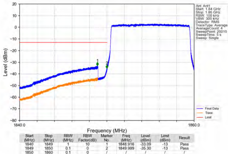
Band2_10MHz_16QAM_LCH_1855MHz_RB_50_0_NTNV
