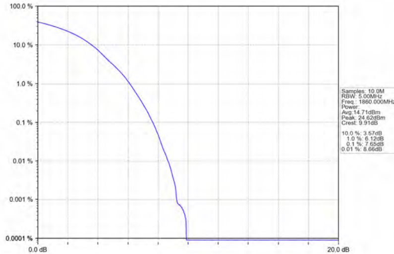
Band2_20MHz_64QAM_LCH_1860MHz_RB_100_0_NTNV
