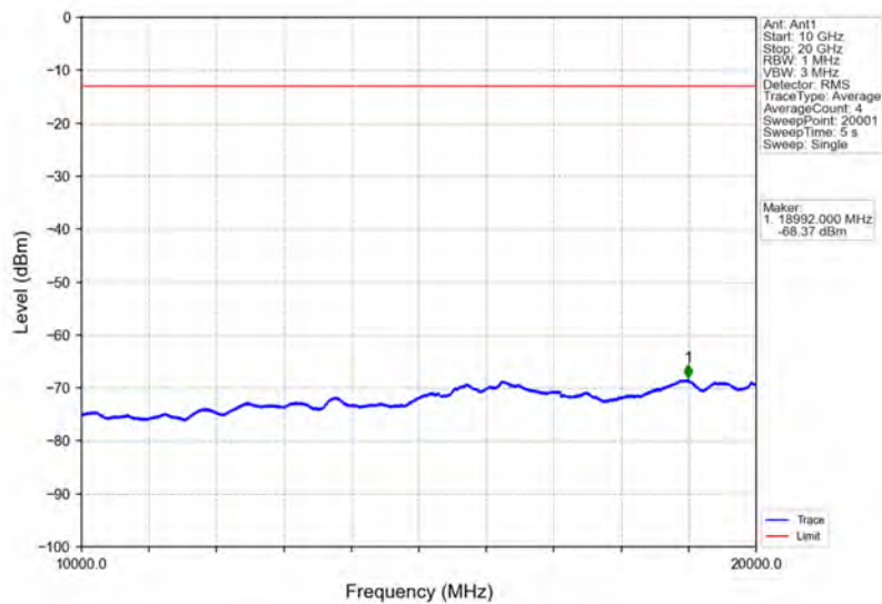
Band2_20MHz_QPSK_HCH_1900MHz_RB_1_0_NTNV
