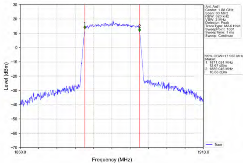
Band2_20MHz_16QAM_MCH_1880MHz_RB_100_0_NTNV
