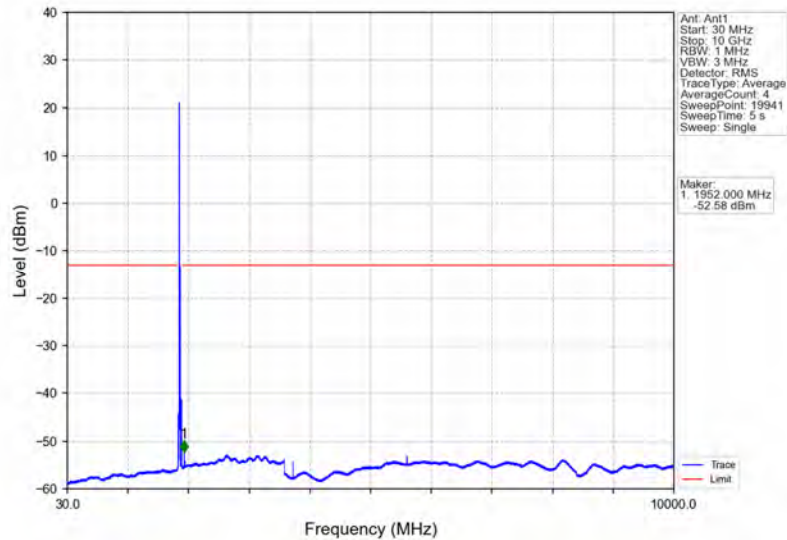
Band2_20MHz_64QAM_MCH_1880MHz_RB_1_0_NTNV
