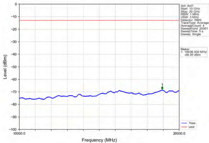
Band2_1.4MHz_QPSK_HCH_1909.3MHz_RB_1_0_NTNV
