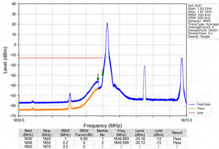
Band2_20MHz_16QAM_LCH_1860MHz_RB_1_0_NTNV
