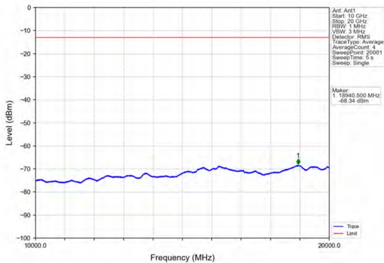
Band2_20MHz_64QAM_MCH_1880MHz_RB_1_0_NTNV
