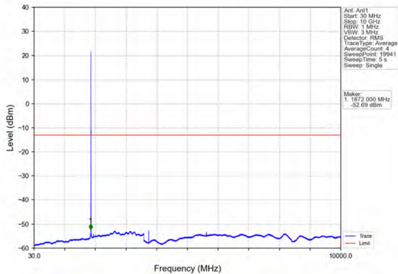
Band2_3MHz_16QAM_MCH_1880MHz_RB_1_0_NTNV
