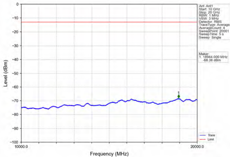
Band2_10MHz_64QAM_LCH_1855MHz_RB_50_0_NTNV
