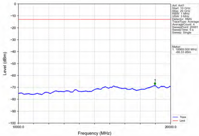
Band2_15MHz_QPSK_HCH_1902.5MHz_RB_1_0_NTNV
