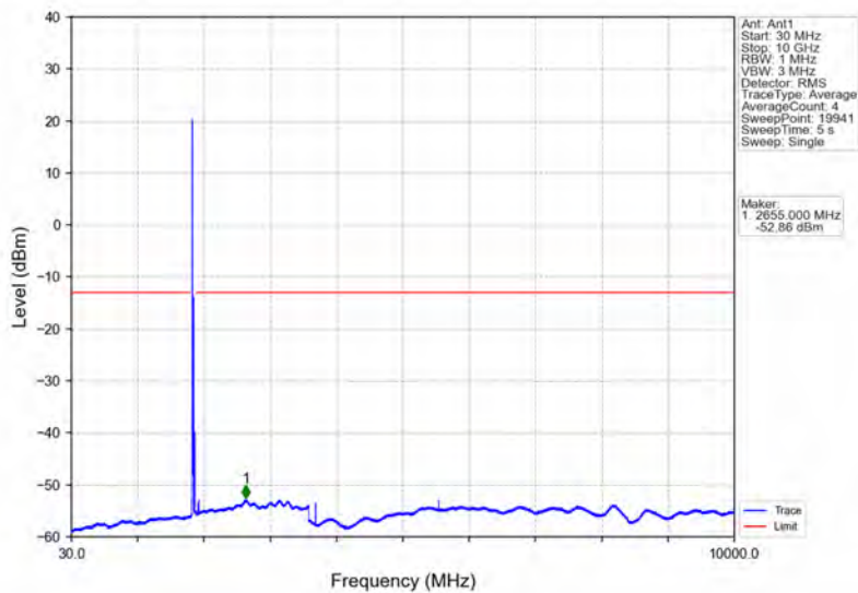
Band2_20MHz_64QAM_LCH_1860MHz_RB_1_0_NTNV
