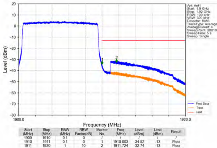
Band2_10MHz_QPSK_HCH_1905MHz_RB_50_0_NTNV
