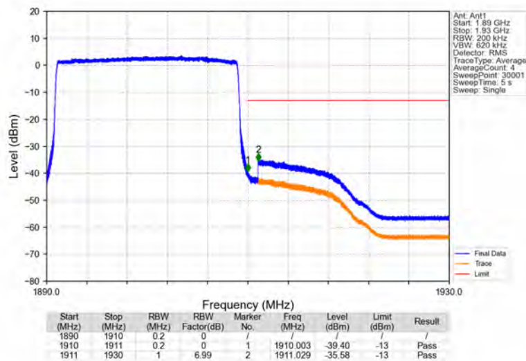
Band2_20MHz_16QAM_HCH_1900MHz_RB_100_0_NTNV
