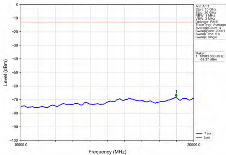
Band2_20MHz_16QAM_HCH_1900MHz_RB_1_0_NTNV
