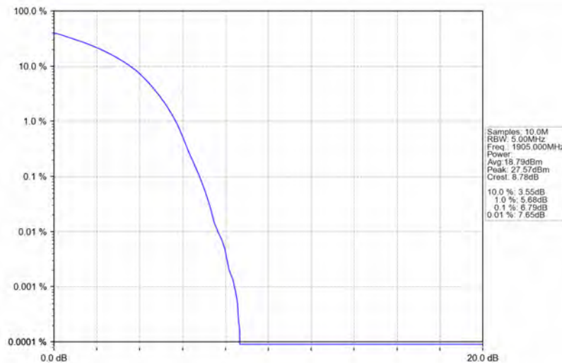
Band2_10MHz_16QAM_HCH_1905MHz_RB_50_0_NTNV
