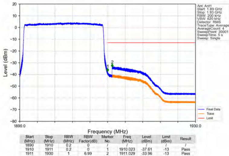
Band2_20MHz_QPSK_HCH_1900MHz_RB_100_0_NTNV
