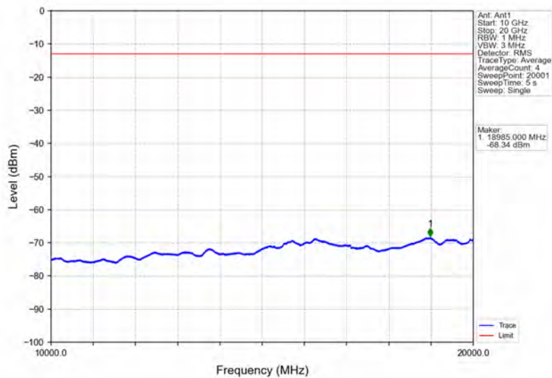
Band2_10MHz_16QAM_MCH_1880MHz_RB_1_0_NTNV
