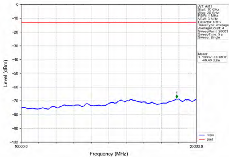
Band2_3MHz_QPSK_HCH_1908.5MHz_RB_1_0_NTNV
