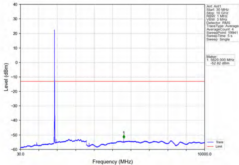
Band2_15MHz_QPSK_MCH_1880MHz_RB_1_0_NTNV
