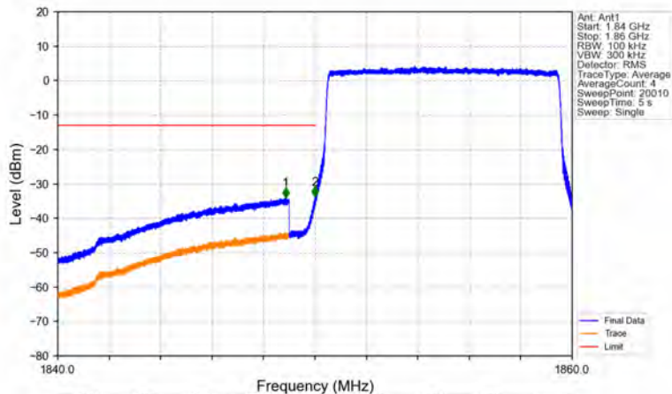
Band2_10MHz_QPSK_LCH_1855MHz_RB_50_0_NTNV
