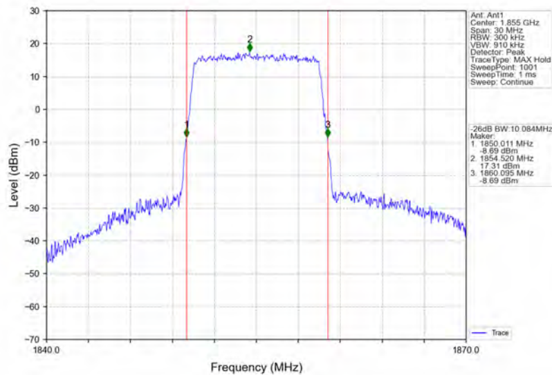
Band2_10MHz_QPSK_LCH_1855MHz_RB_50_0_NTNV
