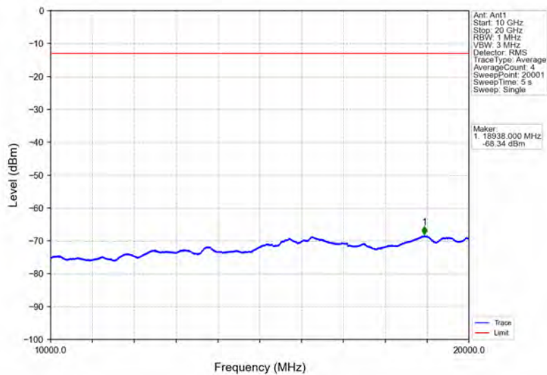
Band2_20MHz_QPSK_MCH_1880MHz_RB_1_0_NTNV
