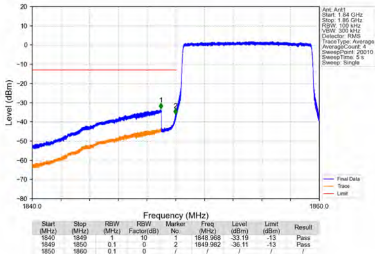
Band2_10MHz_64QAM_LCH_1855MHz_RB_50_0_NTNV
