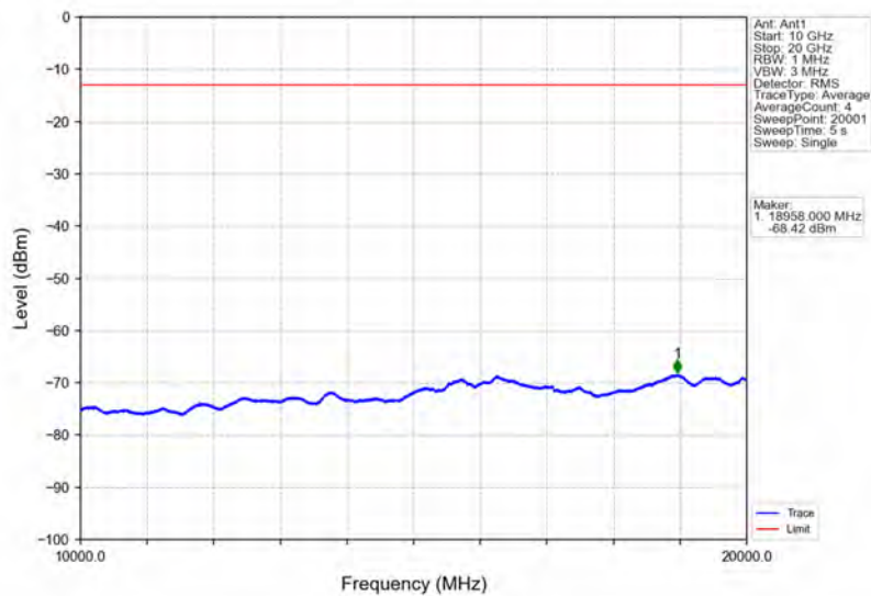
Band2_10MHz_QPSK_MCH_1880MHz_RB_1_0_NTNV
