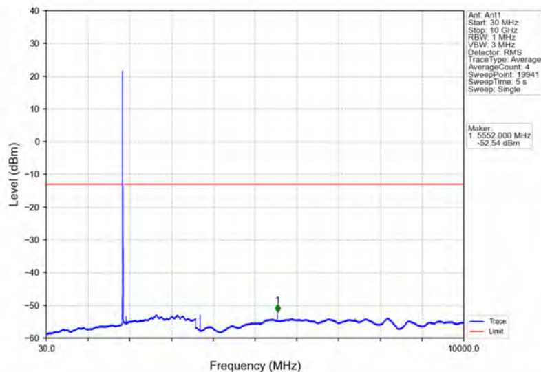
Band2_10MHz_16QAM_LCH_1855MHz_RB_1_0_NTNV
