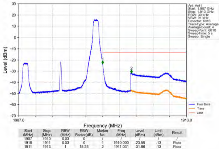
Band2_3MHz_QPSK_HCH_1908.5MHz_RB_1_14_NTNV
