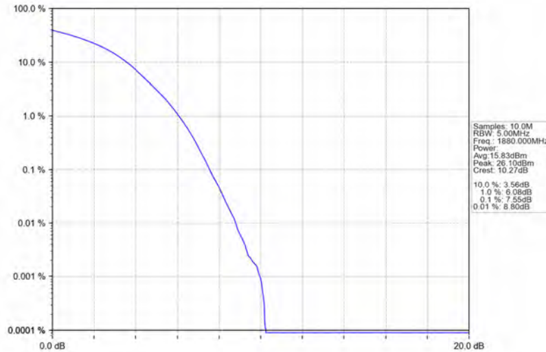
Band2_20MHz_16QAM_MCH_1880MHz_RB_100_0_NTNV
