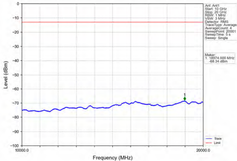
Band2_10MHz_16QAM_LCH_1855MHz_RB_50_0_NTNV
