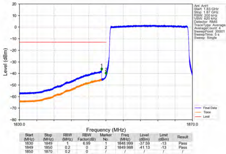
Band2_20MHz_64QAM_LCH_1860MHz_RB_100_0_NTNV
