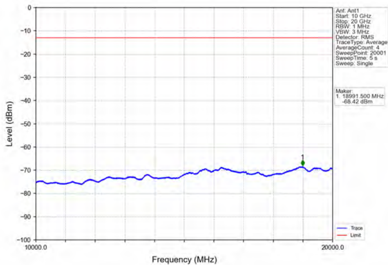
Band2_5MHz_QPSK_MCH_1880MHz_RB_1_0_NTNV
