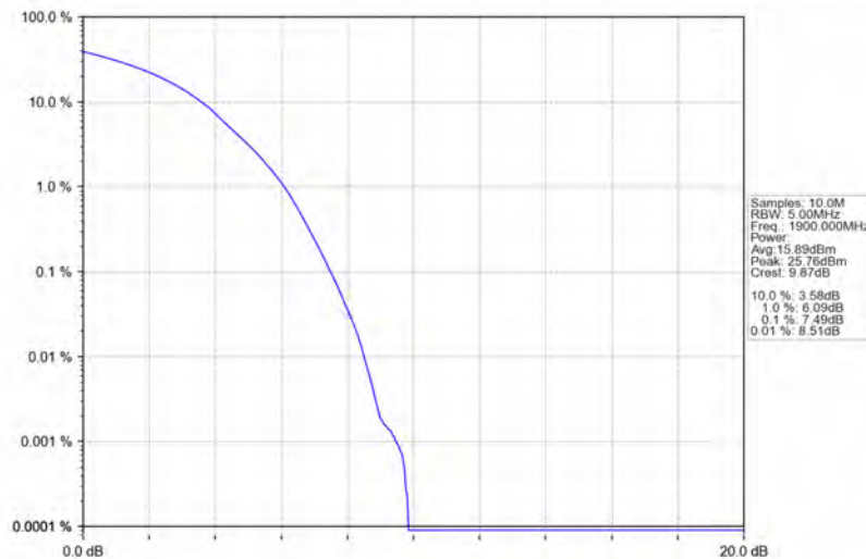
Band2_20MHz_16QAM_HCH_1900MHz_RB_100_0_NTNV
