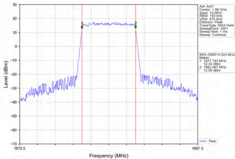
Band2_5MHz_QPSK_MCH_1880MHz_RB_25_0_NTNV
