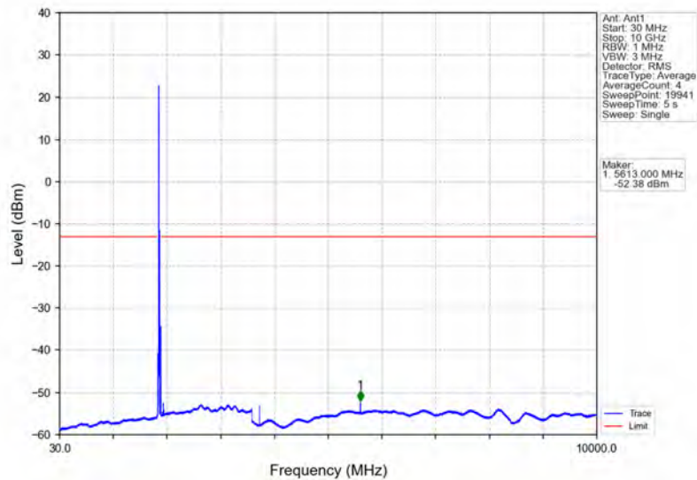
Band2_20MHz_QPSK_MCH_1880MHz_RB_1_0_NTNV
