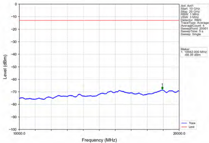
Band2_20MHz_16QAM_MCH_1880MHz_RB_1_0_NTNV
