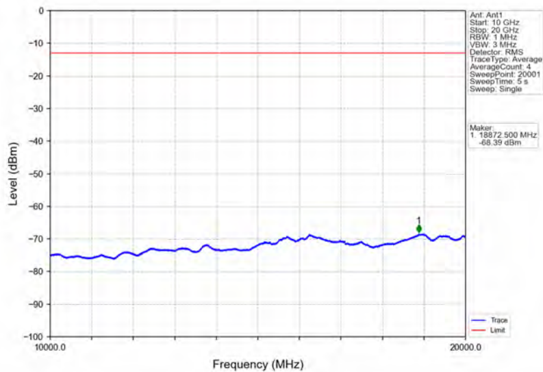
Band2_10MHz_16QAM_HCH_1905MHz_RB_1_0_NTNV
