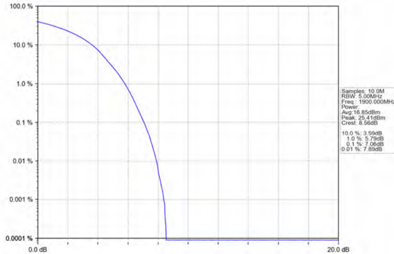
Band2_20MHz_QPSK_HCH_1900MHz_RB_100_0_NTNV
