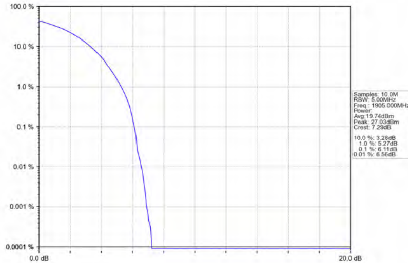
Band2_10MHz_QPSK_HCH_1905MHz_RB_50_0_NTNV
