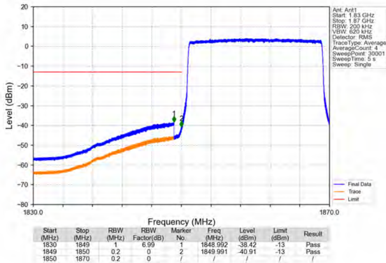
Band2_20MHz_QPSK_LCH_1860MHz_RB_100_0_NTNV
