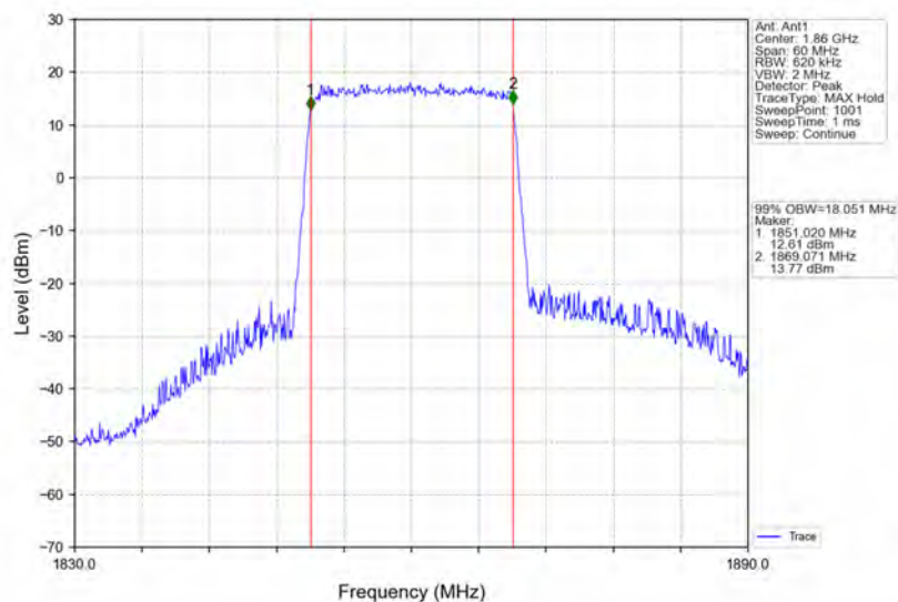
Band2_20MHz_QPSK_LCH_1860MHz_RB_100_0_NTNV
