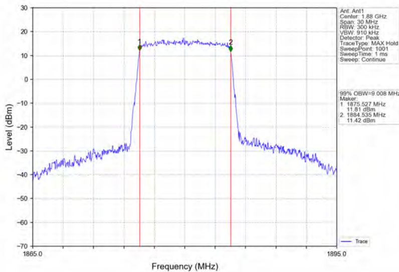
Band2_10MHz_16QAM_MCH_1880MHz_RB_50_0_NTNV
