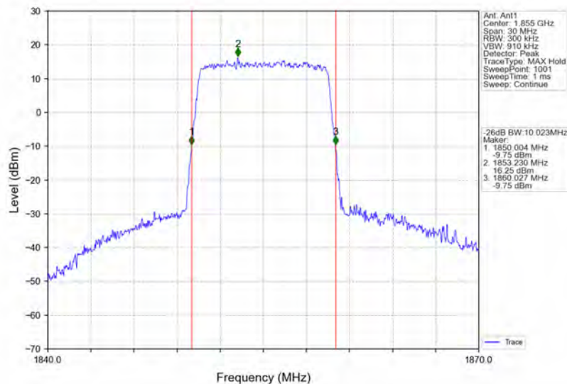
Band2_10MHz_64QAM_LCH_1855MHz_RB_50_0_NTNV
