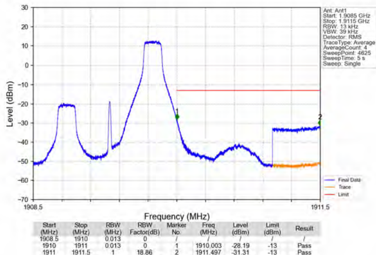
Band2_1.4MHz_QPSK_HCH_1909.3MHz_RB_1_5_NTNV
