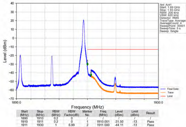
Band2_20MHz_64QAM_HCH_1900MHz_RB_1_99_NTNV
