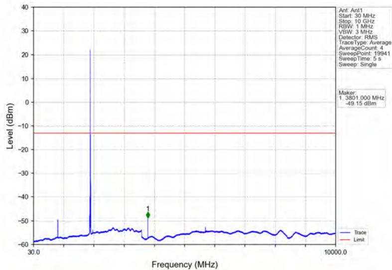
Band2_10MHz_16QAM_HCH_1905MHz_RB_1_0_NTNV
