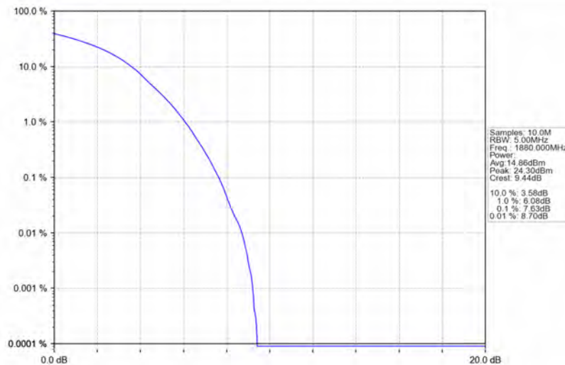
Band2_20MHz_64QAM_MCH_1880MHz_RB_100_0_NTNV
