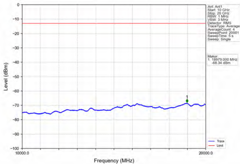
Band2_1.4MHz_QPSK_MCH_1880MHz_RB_1_0_NTNV
