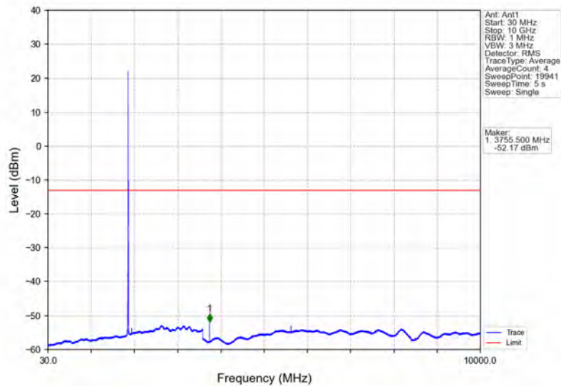
Band2_5MHz_QPSK_MCH_1880MHz_RB_1_0_NTNV
