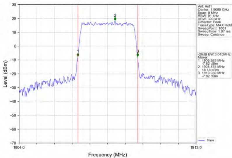
Band2_3MHz_QPSK_HCH_1908.5MHz_RB_15_0_NTNV
