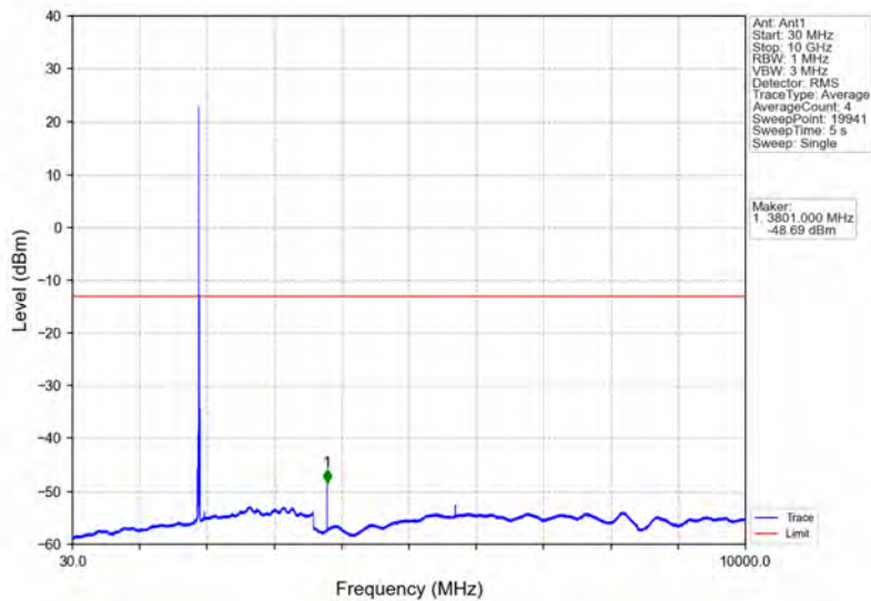
Band2_10MHz_QPSK_HCH_1905MHz_RB_1_0_NTNV
