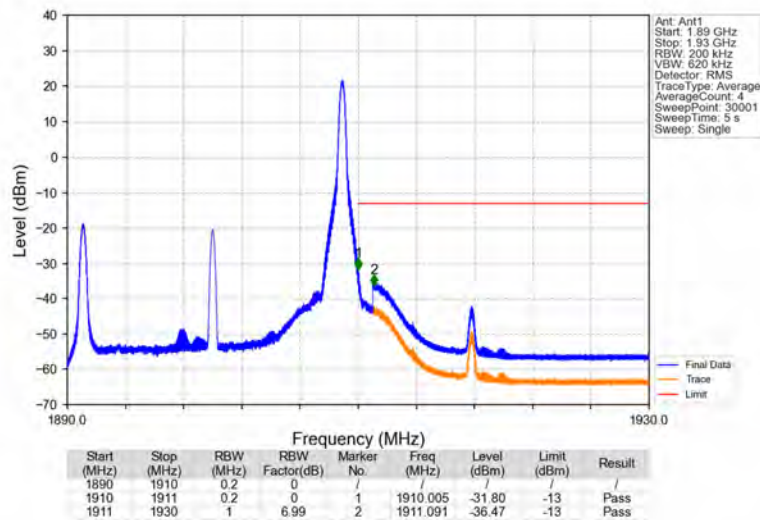
Band2_20MHz_16QAM_HCH_1900MHz_RB_1_99_NTNV
