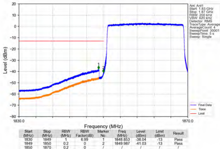
Band2_20MHz_16QAM_LCH_1860MHz_RB_100_0_NTNV
