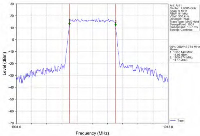
Band2_3MHz_QPSK_HCH_1908.5MHz_RB_15_0_NTNV
