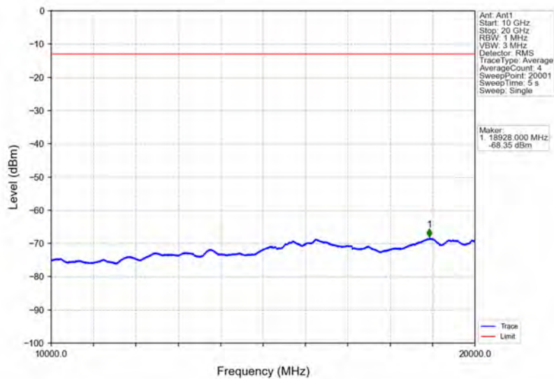
Band2_10MHz_QPSK_HCH_1905MHz_RB_1_0_NTNV
