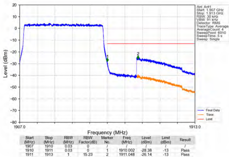
Band2_3MHz_QPSK_HCH_1908.5MHz_RB_15_0_NTNV
