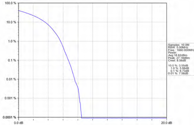
Band2_10MHz_16QAM_MCH_1880MHz_RB_50_0_NTNV
