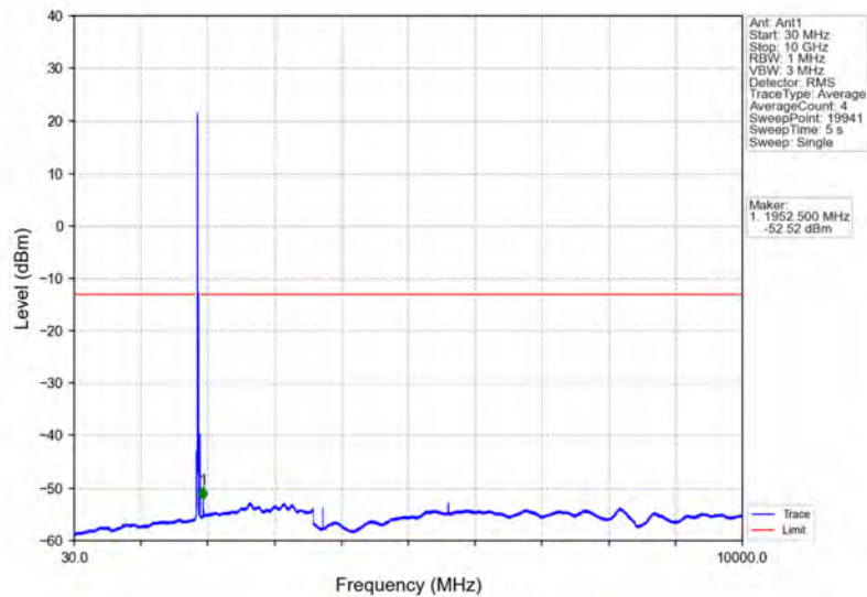
Band2_20MHz_16QAM_MCH_1880MHz_RB_1_0_NTNV
