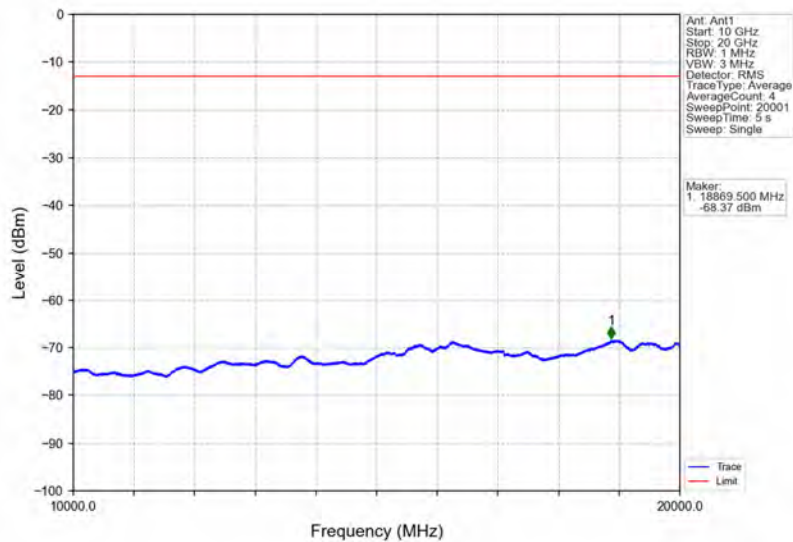
Band2_20MHz_16QAM_LCH_1860MHz_RB_100_0_NTNV
