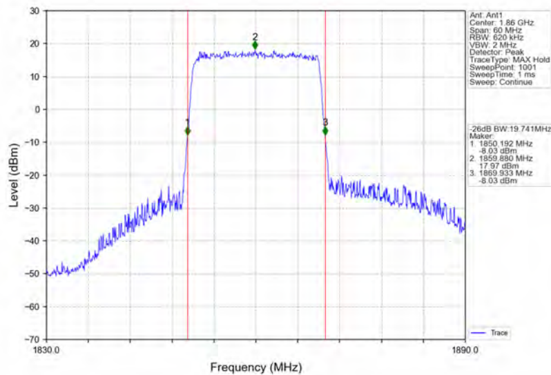
Band2_20MHz_QPSK_LCH_1860MHz_RB_100_0_NTNV
