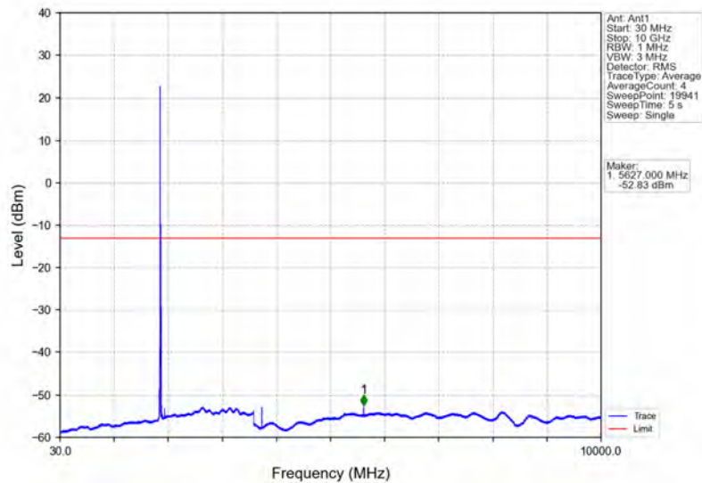
Band2_10MHz_QPSK_MCH_1880MHz_RB_1_0_NTNV
