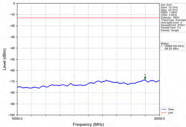
Band2_20MHz_64QAM_LCH_1860MHz_RB_100_0_NTNV
