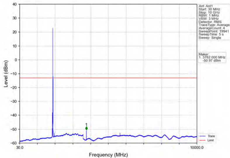
Band2_20MHz_QPSK_HCH_1900MHz_RB_1_0_NTNV
