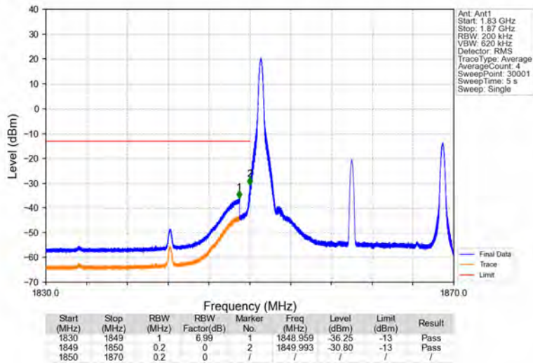
Band2_20MHz_64QAM_LCH_1860MHz_RB_1_0_NTNV
