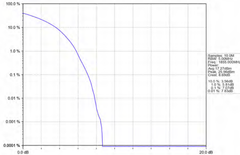
Band2_10MHz_64QAM_LCH_1855MHz_RB_50_0_NTNV
