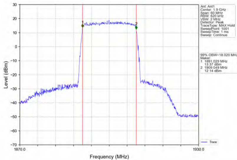
Band2_20MHz_QPSK_HCH_1900MHz_RB_100_0_NTNV
