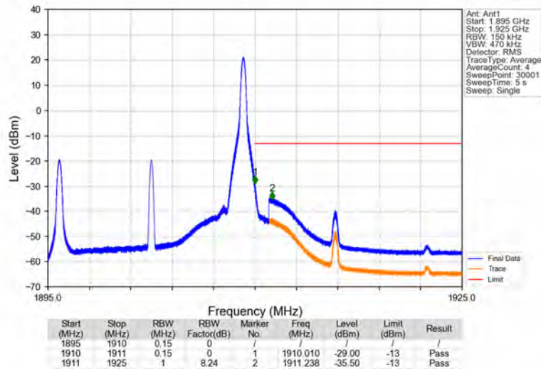
Band2_15MHz_16QAM_HCH_1902.5MHz_RB_1_74_NTNV
