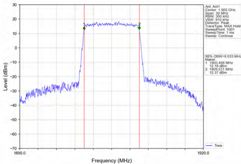
Band2_10MHz_QPSK_HCH_1905MHz_RB_50_0_NTNV
