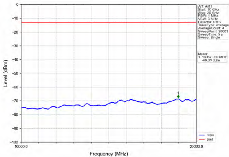
Band2_15MHz_QPSK_MCH_1880MHz_RB_1_0_NTNV
