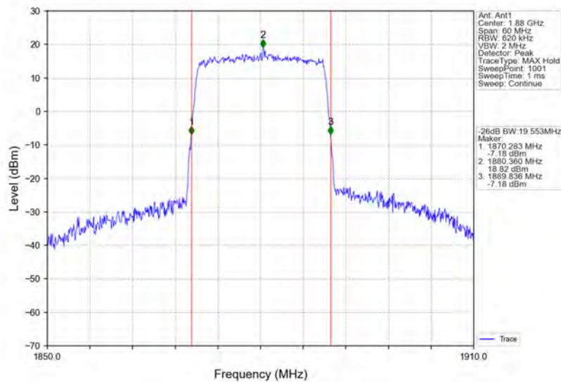
Band2_20MHz_16QAM_MCH_1880MHz_RB_100_0_NTNV
