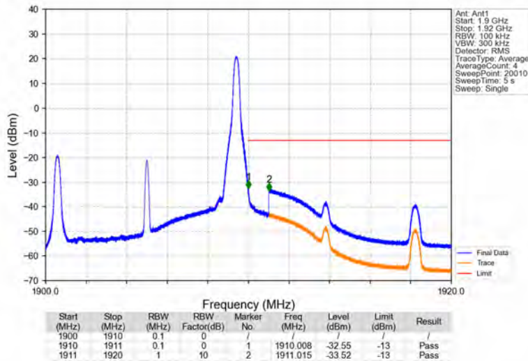
Band2_10MHz_QPSK_HCH_1905MHz_RB_1_49_NTNV
