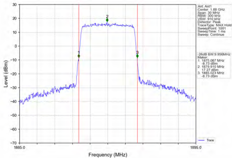
Band2_10MHz_16QAM_MCH_1880MHz_RB_50_0_NTNV
