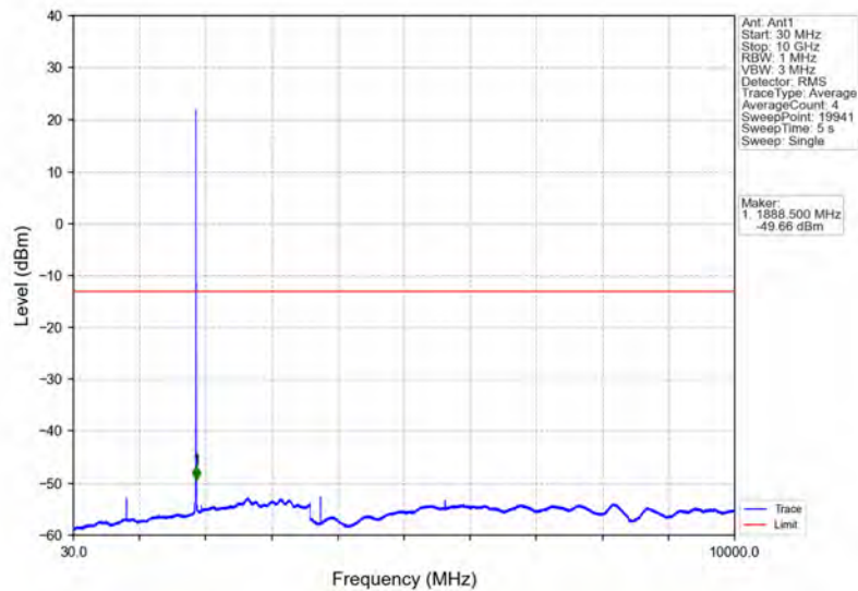
Band2_3MHz_QPSK_MCH_1880MHz_RB_1_0_NTNV
