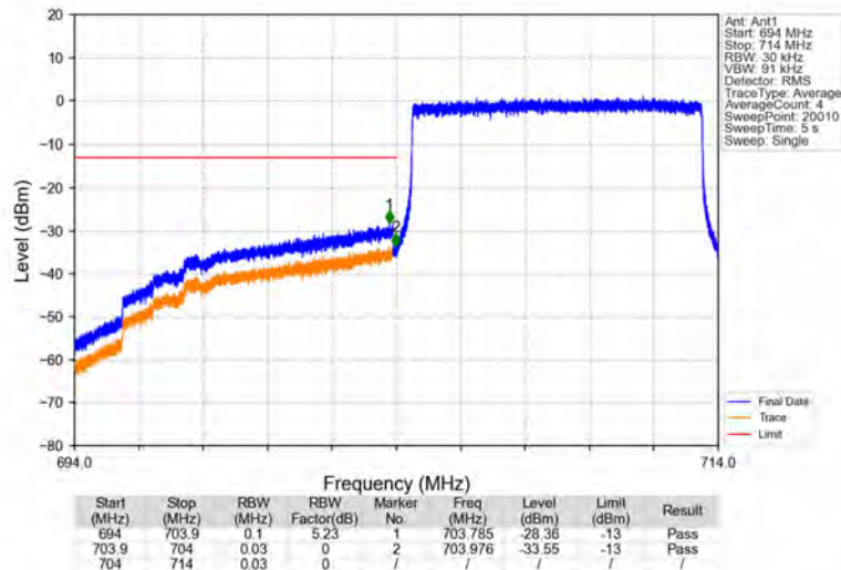
Band17_10MHz_QPSK_LCH_709MHz_RB_50_0_NTNV
