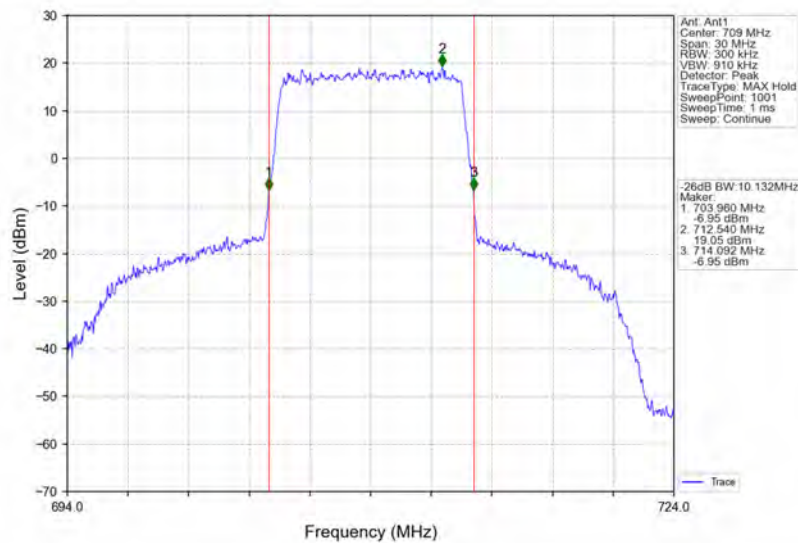
Band17_10MHz_QPSK_LCH_709MHz_RB_50_0_NTNV
