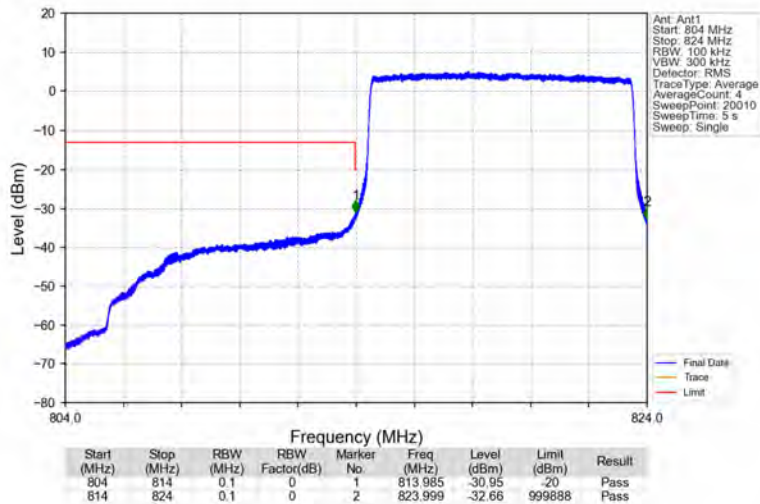
Band26a_10MHz_QPSK_LCH_819MHz_RB_50_0_NTNV
