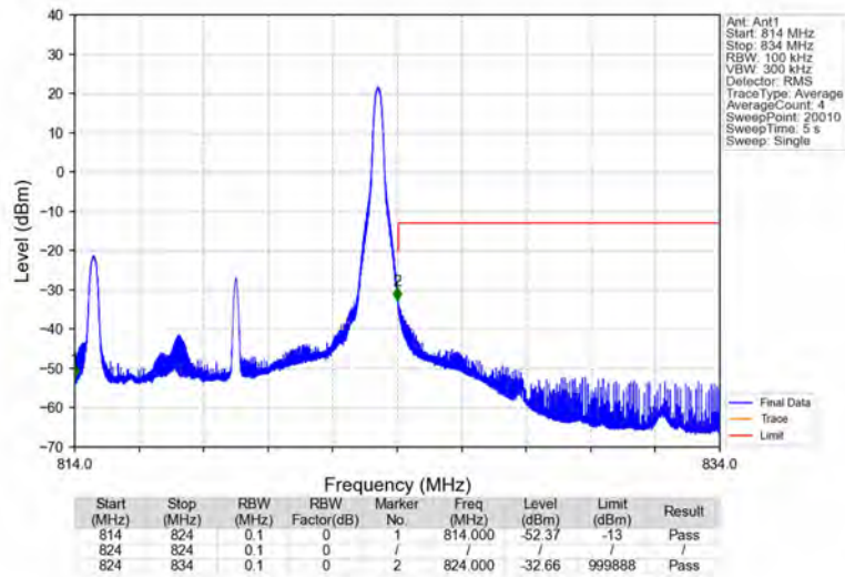
Band26a_10MHz_QPSK_HCH_819MHz_RB_1_49_NTNV
