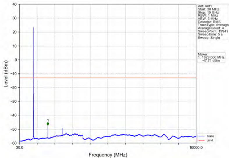
Band26a_10MHz_QPSK_HCH_819MHz_RB_1_49_NTNV
