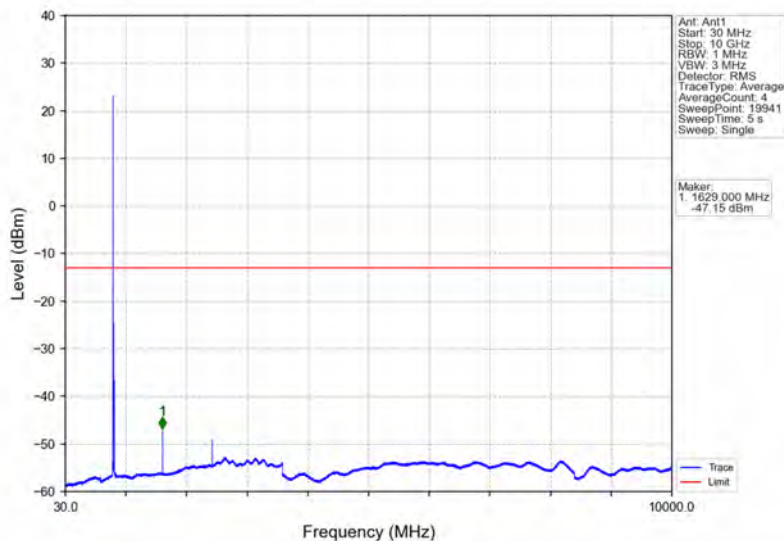
Band26a_10MHz_QPSK_MCH_819MHz_RB_1_0_NTNV
