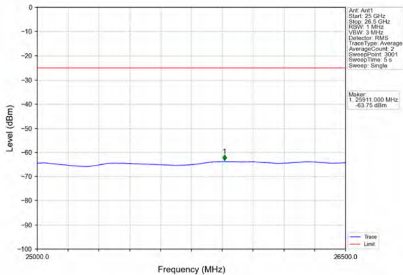
Band41_10MHz_QPSK_HCH_2685MHz_RB_1_49_NTNV
