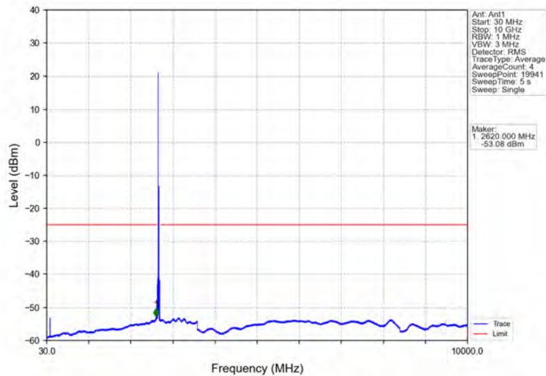
Band41_20MHz_QPSK_HCH_2680MHz_RB_1_0_NTNV
