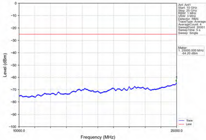
Band41_10MHz_QPSK_MCH_2593MHz_RB_1_0_NTNV
