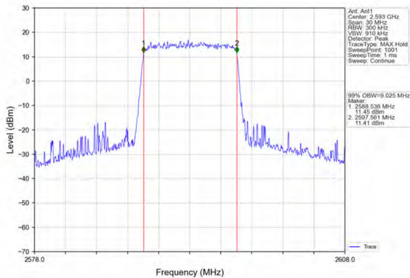
Band41_10MHz_16QAM_MCH_2593MHz_RB_50_0_NTNV
