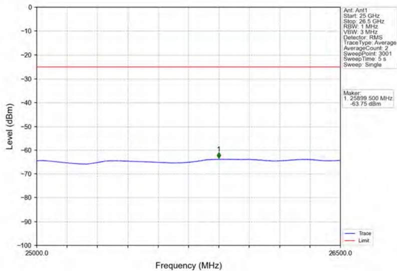
Band41_10MHz_16QAM_HCH_2685MHz_RB_1_0_NTNV
