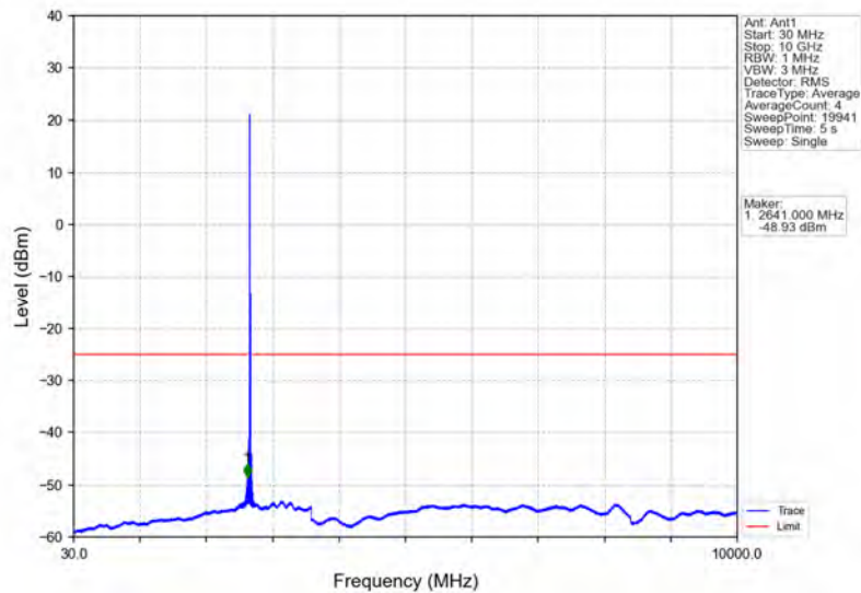
Band41_15MHz_QPSK_HCH_2682.5MHz_RB_1_0_NTNV
