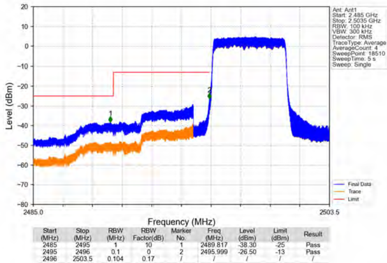
Band41_5MHz_QPSK_LCH_2498.5MHz_RB_25_0_NTNV
