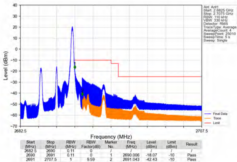
Band41_5MHz_QPSK_HCH_2687.5MHz_RB_1_24_NTNV
