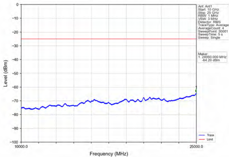
Band41_20MHz_16QAM_MCH_2593MHz_RB_1_0_NTNV
