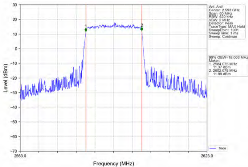
Band41_20MHz_16QAM_MCH_2593MHz_RB_100_0_NTNV
