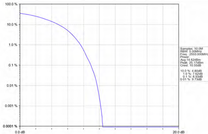
Band41_10MHz_64QAM_MCH_2593MHz_RB_50_0_NTNV
