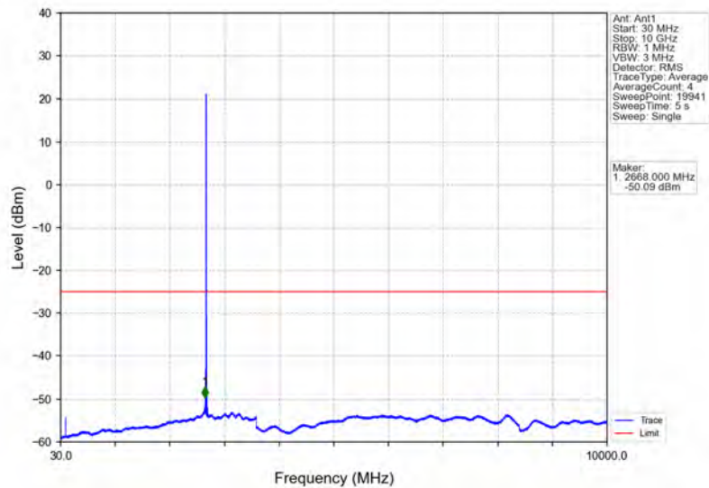
Band41_5MHz_QPSK_HCH_2687.5MHz_RB_1_0_NTNV
