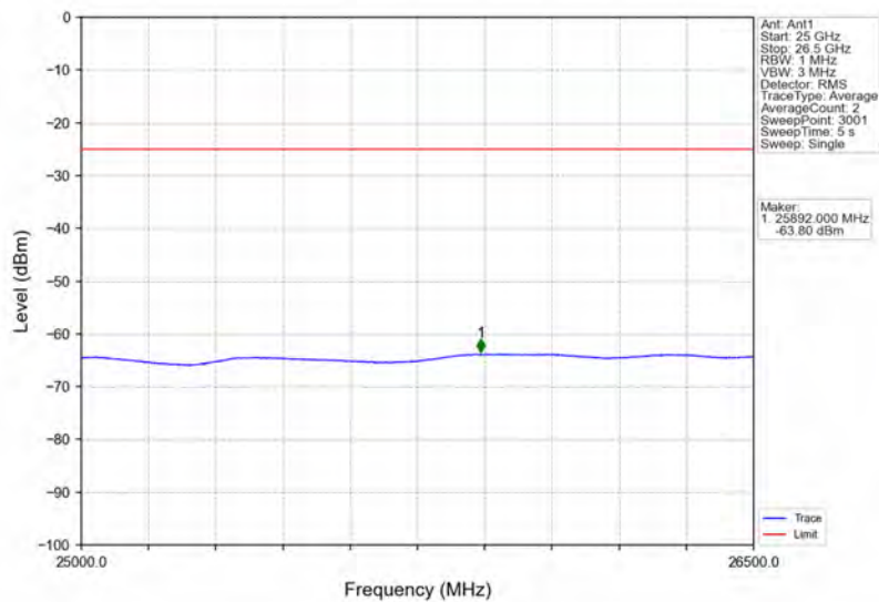
Band41_15MHz_QPSK_MCH_2593MHz_RB_1_0_NTNV
