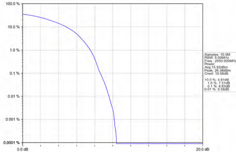
Band41_10MHz_16QAM_MCH_2593MHz_RB_50_0_NTNV
