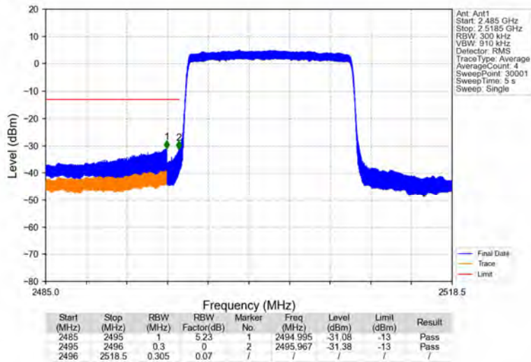
Band41_15MHz_QPSK_LCH_2503.5MHz_RB_75_0_NTNV
