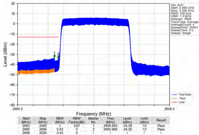
Band41_20MHz_QPSK_LCH_2506MHz_RB_100_0_NTNV
