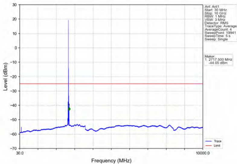
Band41_10MHz_16QAM_HCH_2685MHz_RB_1_0_NTNV
