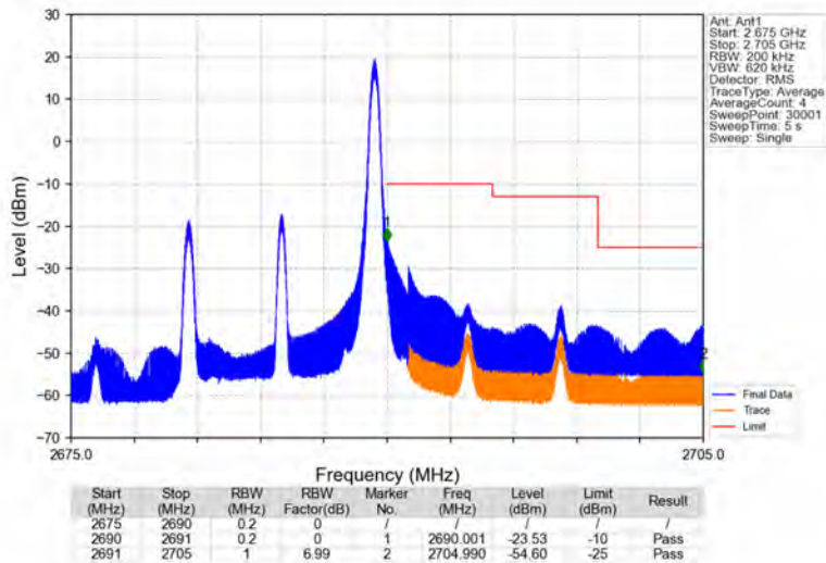
Band41_10MHz_64QAM_HCH_2685MHz_RB_1_49_NTNV
