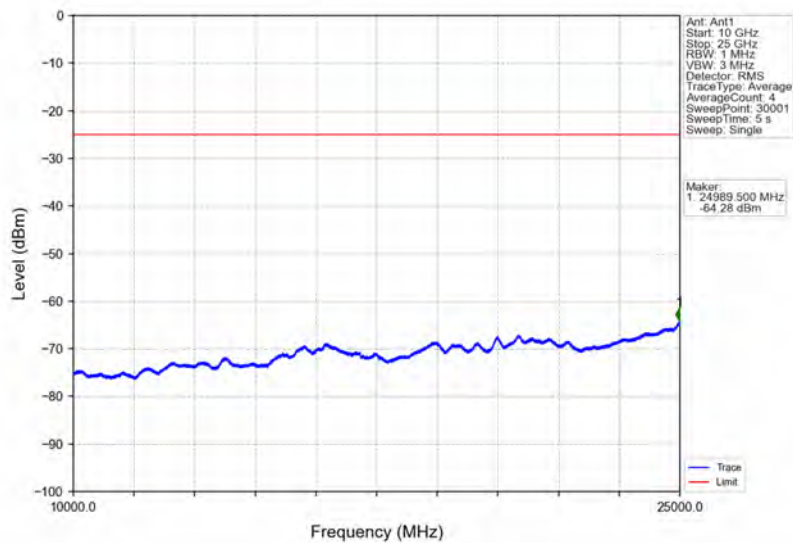
Band41_10MHz_16QAM_LCH_2501MHz_RB_1_0_NTNV
