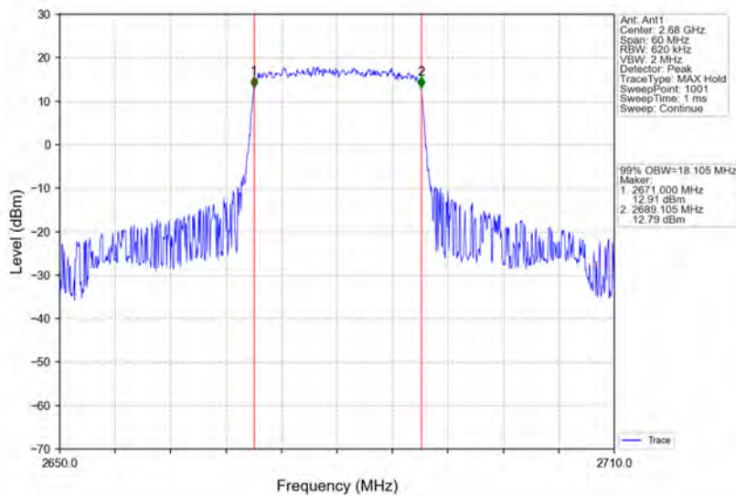
Band41_20MHz_QPSK_HCH_2680MHz_RB_100_0_NTNV
