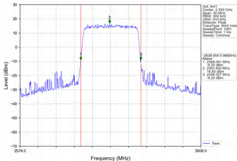
Band41_10MHz_16QAM_MCH_2593MHz_RB_50_0_NTNV
