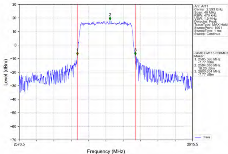
Band41_15MHz_QPSK_MCH_2593MHz_RB_75_0_NTNV
