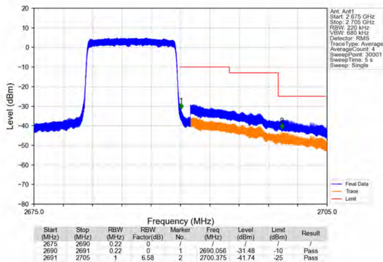
Band41_10MHz_16QAM_HCH_2685MHz_RB_50_0_NTNV
