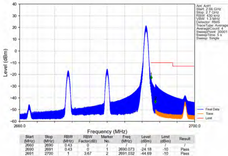
Band41_20MHz_QPSK_HCH_2680MHz_RB_1_99_NTNV
