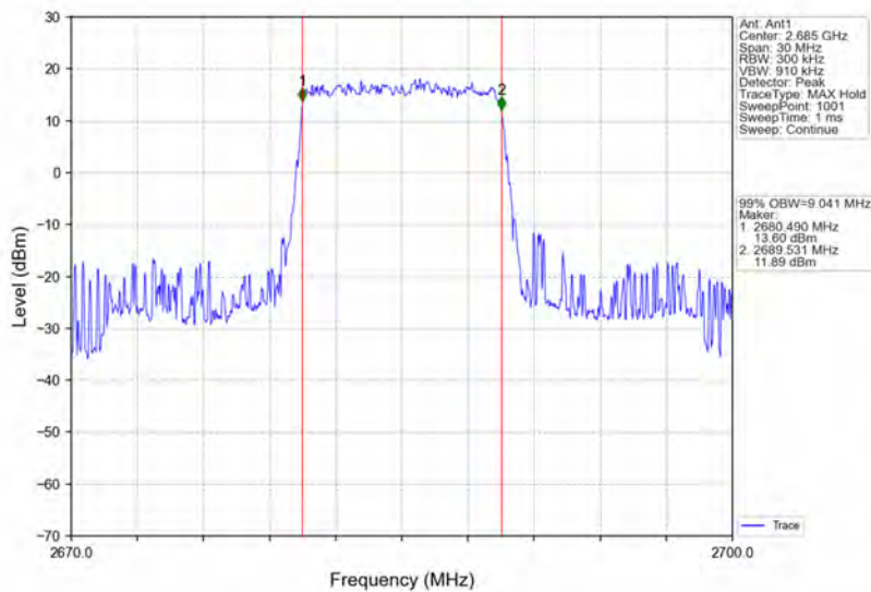
Band41_10MHz_QPSK_HCH_2685MHz_RB_50_0_NTNV
