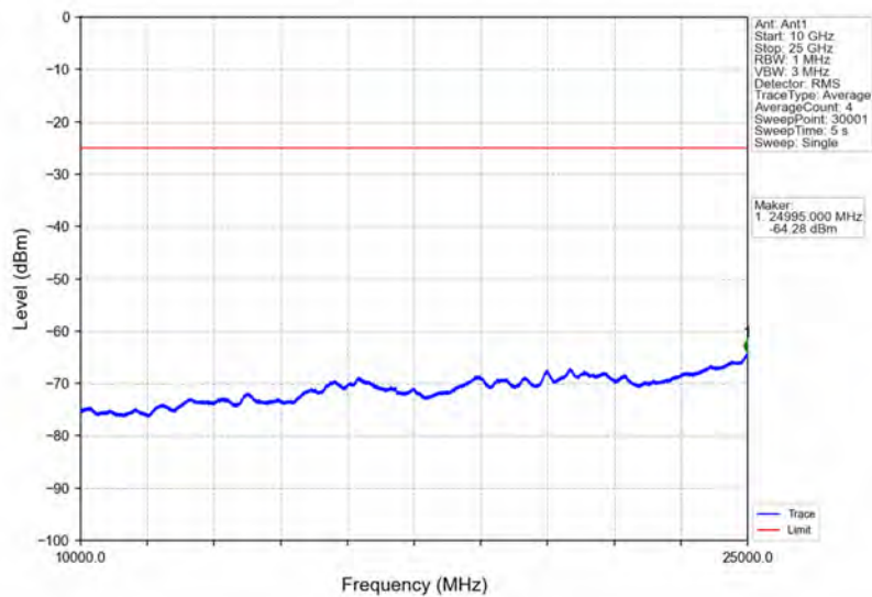
Band41_20MHz_QPSK_HCH_2680MHz_RB_1_0_NTNV
