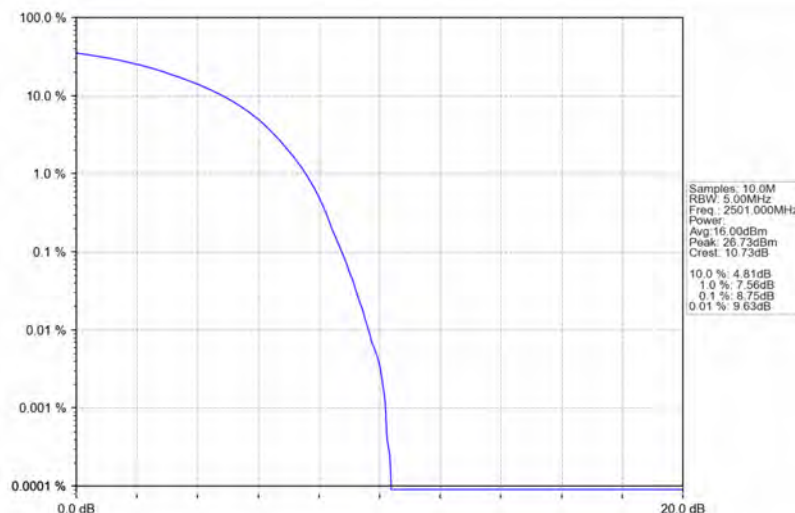
Band41_10MHz_16QAM_LCH_2501MHz_RB_50_0_NTNV
