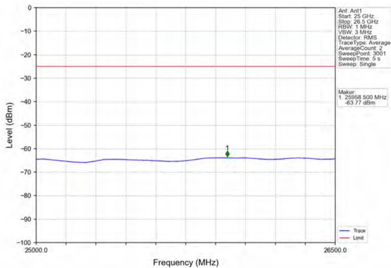
Band41_15MHz_QPSK_LCH_2503.5MHz_RB_1_0_NTNV
