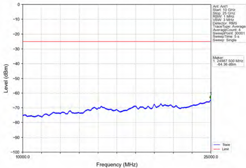
Band41_20MHz_QPSK_LCH_2506MHz_RB_1_0_NTNV
