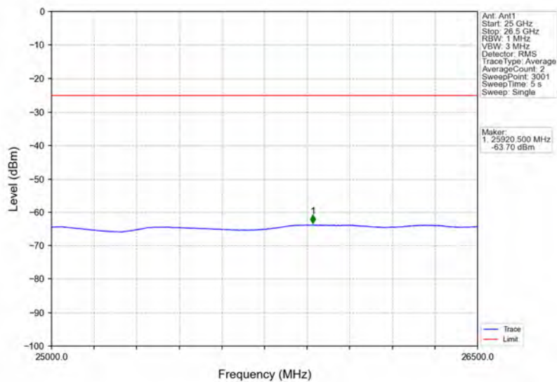
Band41_5MHz_QPSK_HCH_2687.5MHz_RB_1_24_NTNV
