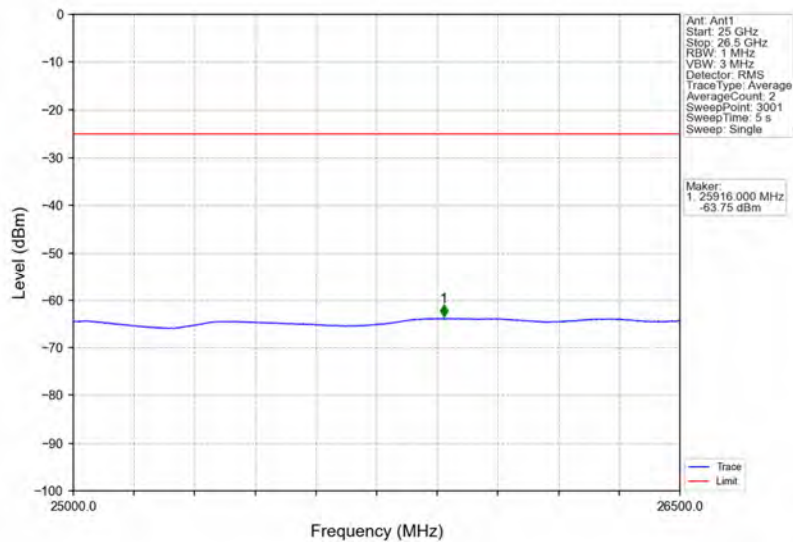
Band41_15MHz_QPSK_HCH_2682.5MHz_RB_1_74_NTNV
