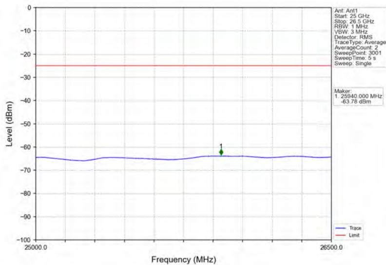
Band41_20MHz_QPSK_MCH_2593MHz_RB_1_0_NTNV
