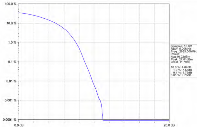
Band41_10MHz_16QAM_HCH_2685MHz_RB_50_0_NTNV
