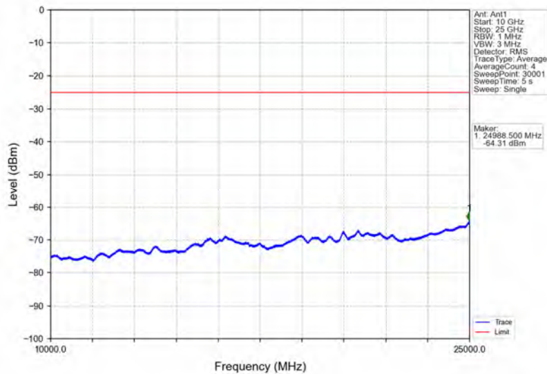
Band41_5MHz_QPSK_MCH_2593MHz_RB_1_0_NTNV
