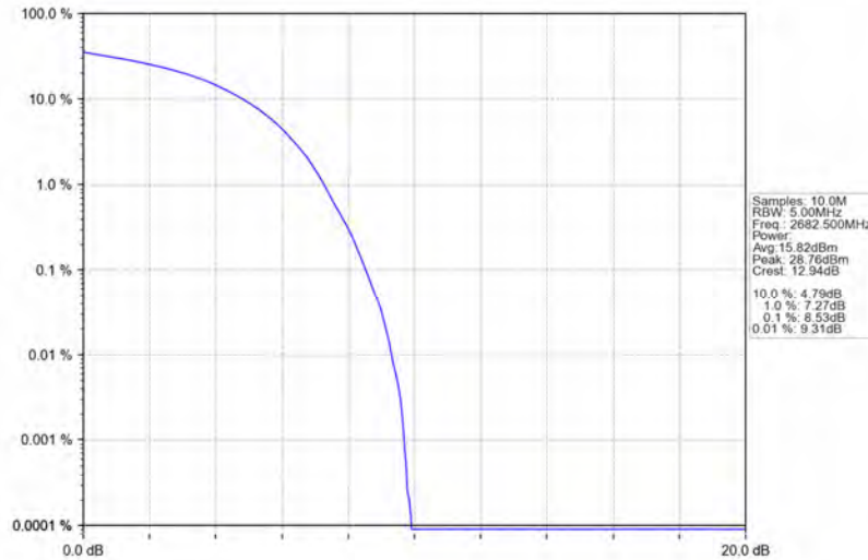
Band41_15MHz_QPSK_HCH_2682.5MHz_RB_75_0_NTNV
