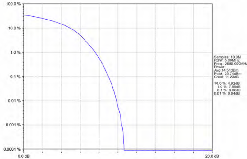
Band41_20MHz_QPSK_HCH_2680MHz_RB_100_0_NTNV
