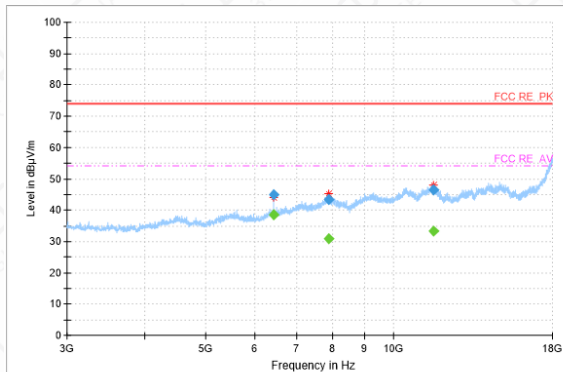
RSE-11B-CH1-3GHz-18GHz
