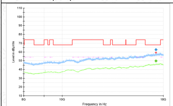
RSE-11N(40M)-CH134-8GHz-18GHz-YLD
