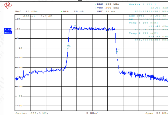
FDD26(PART 22)_Channel Mid_10MHz_836.5MHz _QPSK
