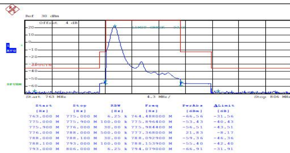
FDD13LowRange_5MHz_QPSK_1RB_LowRange
