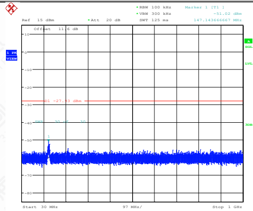
11G-Ant1-2462-30~1000-PASS
