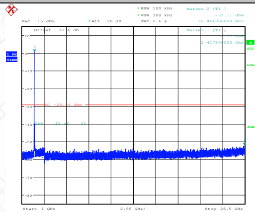
11N20ISO-Ant1-2412-1000~26500-PASS
