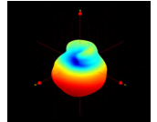
G900/W8(Frequency=940MHz)
