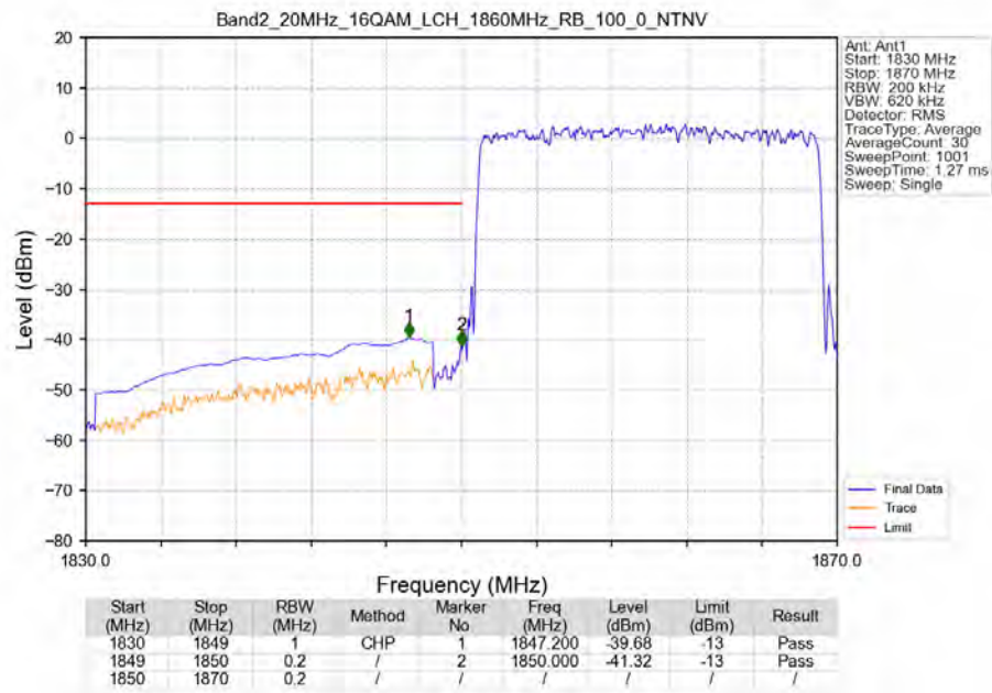
Band2_20MHz_16QAM_LCH_1860MHz_RB_100_0_NTNV
