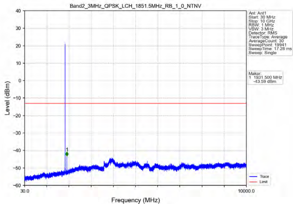
Band2_3MHz_QPSK_LCH_1851.5MHz_RB_1_0_NTNV
