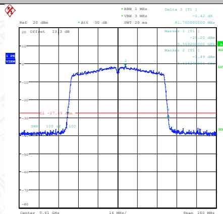
11AC80SISO-Ant1-5610
