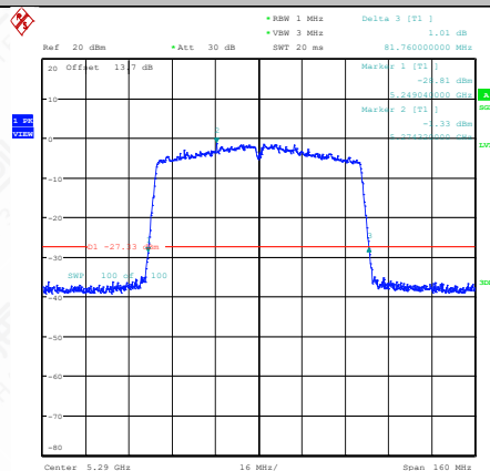
11AC80SISO-Ant1-5290
