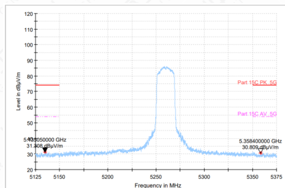
AV detector
