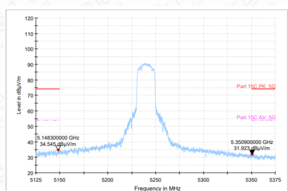
AV detector
