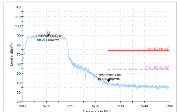
AV detector
