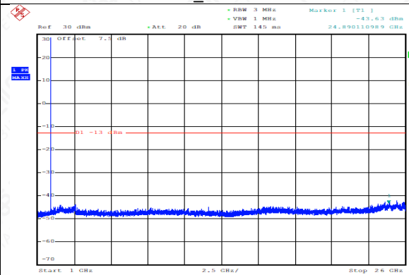
GSM1900_GPRS_810_1000MHz-26000MHz _CSE
