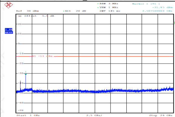
GSM850_EDGE_189_1000MHz-26000MHz_CSE
