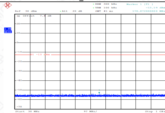
GSM1900_GPRS_661_30MHz-1000MHz _CSE
