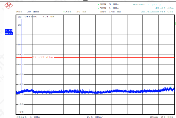
GSM1900_EDGE_661_1000MHz-26000MHz _CSE
