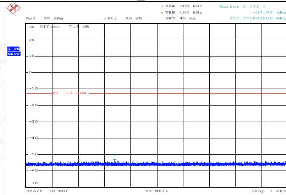
GSM1900_EDGE_512_30MHz-1000MHz _CSE
