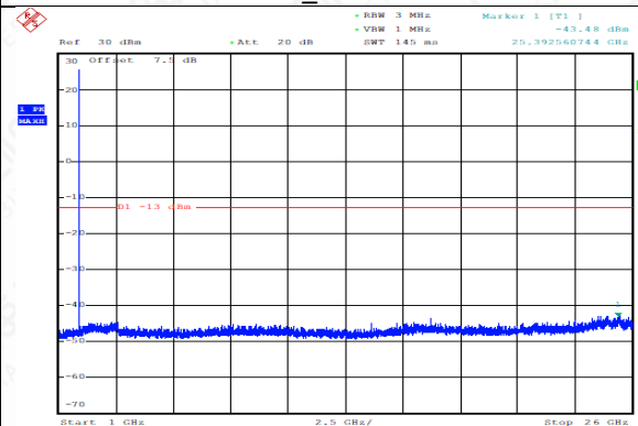
GSM1900_EDGE_810_1000MHz-26000MHz _CSE
