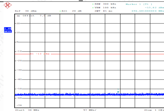
GSM1900_EDGE_810_30MHz-1000MHz _CSE
