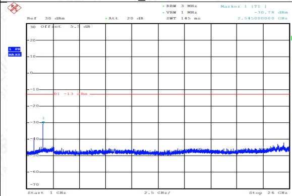
GSM850_EDGE_251_1000MHz-26000MHz_CSE
