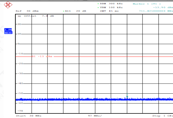
GSM1900_GPRS_512_30MHz-1000MHz _CSE
