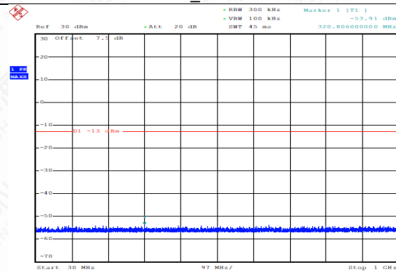
GSM1900_GPRS_810_30MHz-1000MHz _CSE
