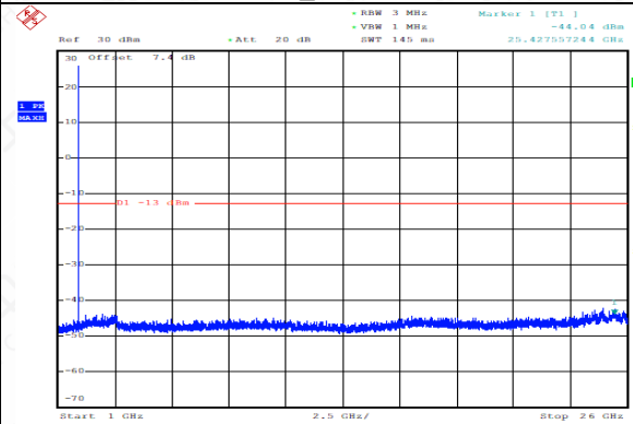
GSM1900_EDGE_512_1000MHz-26000MHz _CSE
