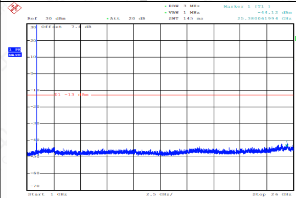
GSM1900_GPRS_512_1000MHz-26000MHz _CSE
