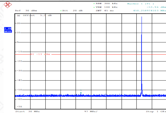
GSM850_EDGE_189_30MHz-1000MHz_CSE
