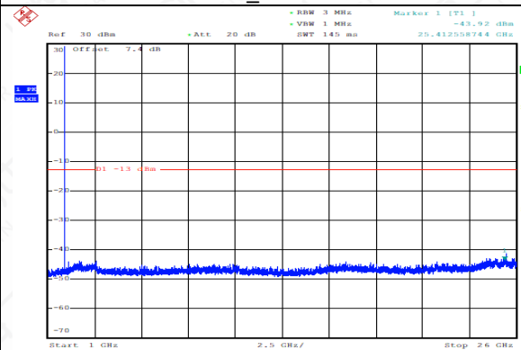
GSM1900_GPRS_661_1000MHz-26000MHz _CSE
